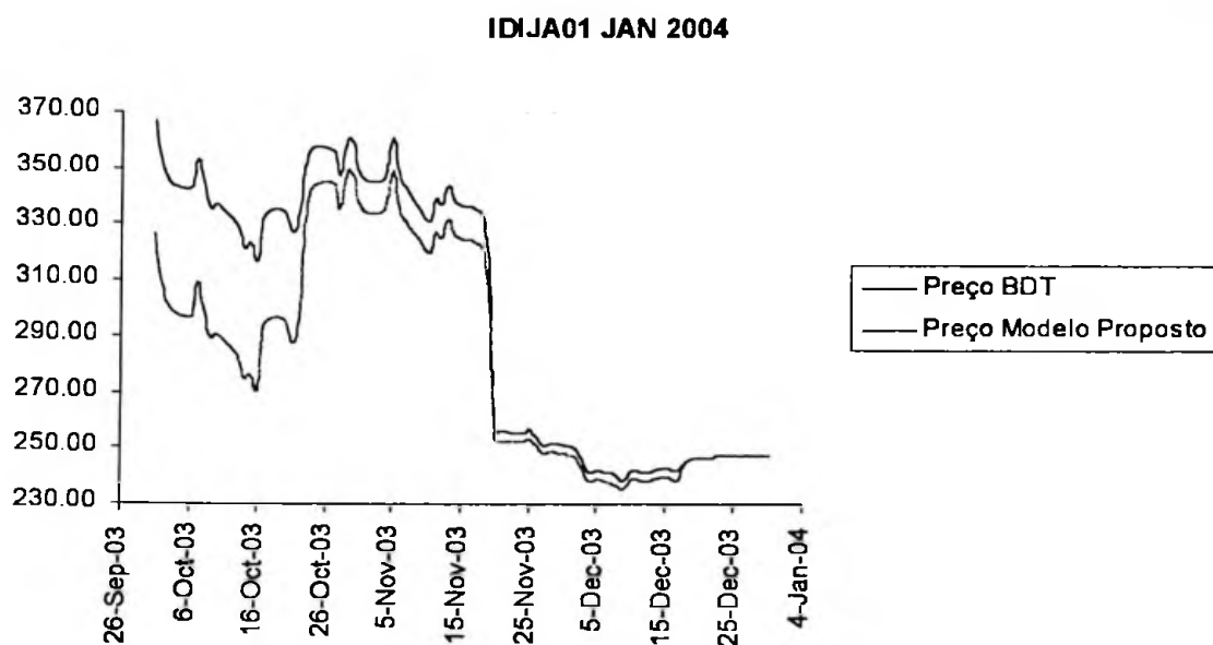
Figura 5-12 Comparação Histórica entre os Preços no Modelo BDT e no Modelo Proposto para a Série IDIJA01 com Vencimento em 02/jan/2004.
