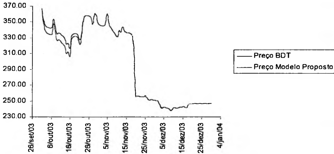
Figura 5-17 Comparação Histórica entre os Preços no Modelo BDT e no Modelo Proposto sem Tendência para a Série IDIJA01 com Vencimento em 02/jan/2004.
