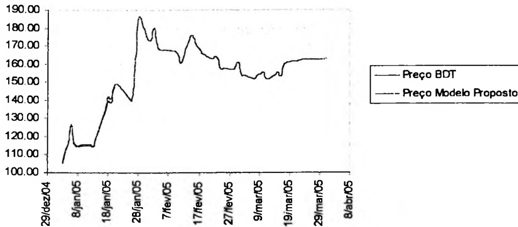
Figura 5-21 Comparação Histórica entre os Preços Pelo Modelo BDT e o Modelo Proposto sem Tendência para a Série IDIAB17 com Vencimento em 01/abr/2005.
