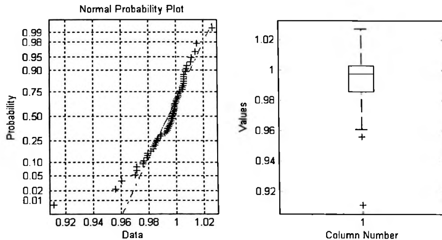
Figura 4-6 Normplot e Boxplot para a série dos percentuais.
