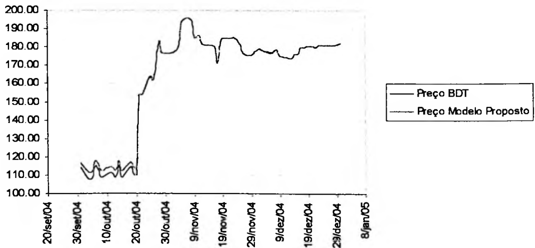
Figura 5-20 Comparação Histórica entre os Preços Pelo Modelo BDT e o Modelo Proposto sem Tendência para a Série IDIJA15 com Vencimento em 03/jan/2005.
