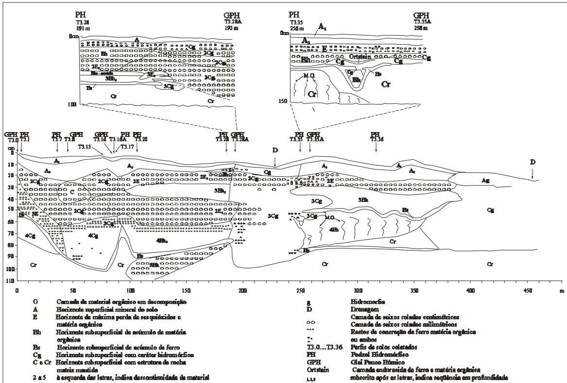
FIGURA 28: Pedotoposequência 3 representando a passagem do solo Podzol para Glei na região do planalto
