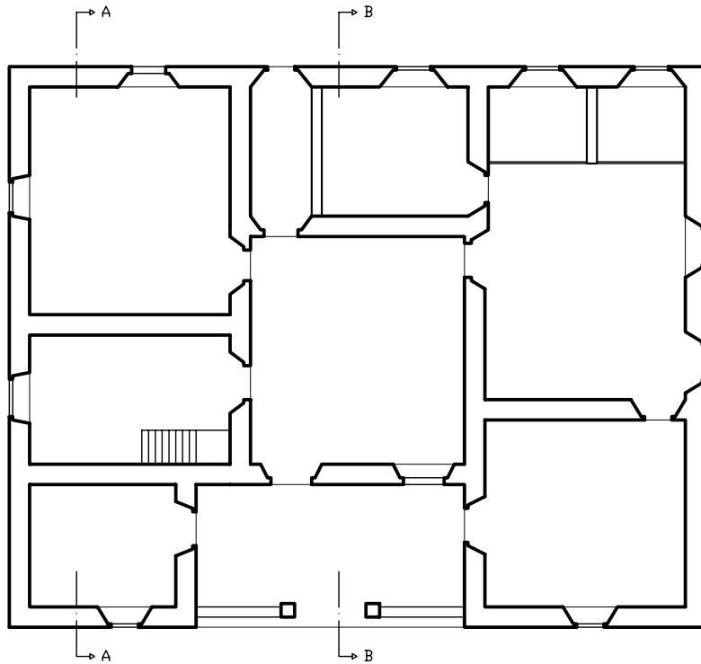
Planta Baixa
