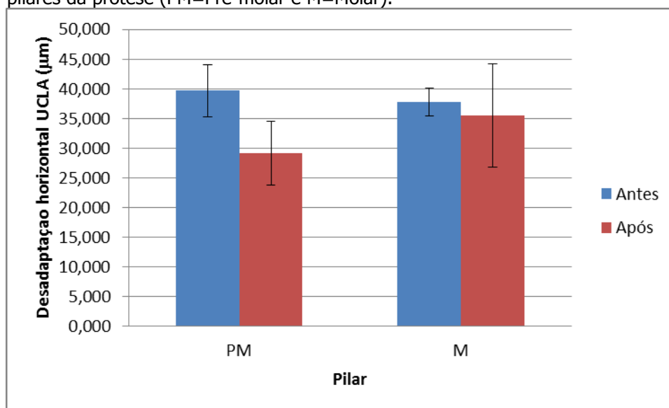
Figura 46: Desadaptação interna horizontal média ( \mu\text{m} ) no grupo UCLA (interface implante/pilar), antes e após ciclagem termomecânica em cada um dos pilares da prótese (PM=Pré-molar e M=Molar).
