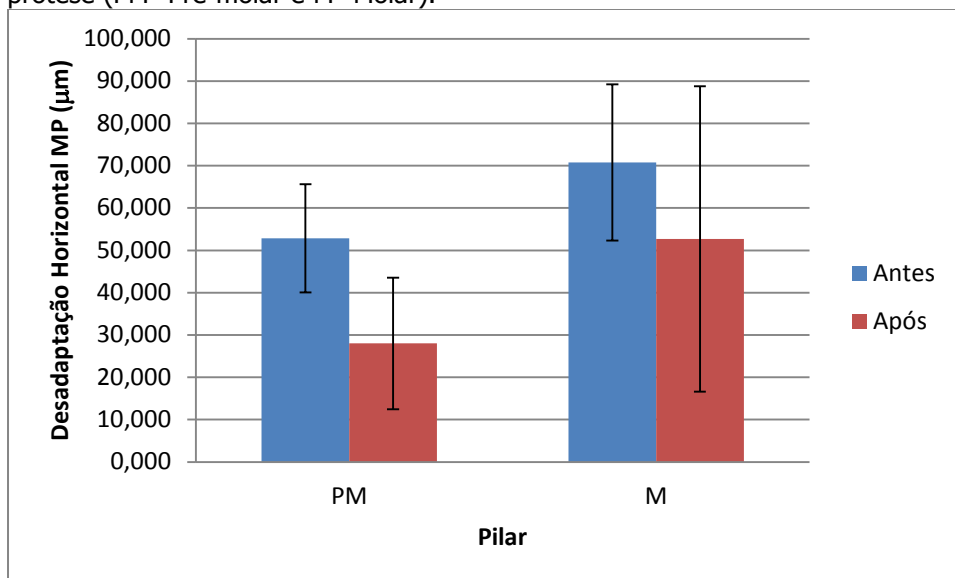
Figura 44: Desadaptação marginal horizontal ( \mu\text{m} ) no grupo Mini-Pilar (interface prótese/pilar), antes e após ciclagem termomecânica em cada um dos pilares da prótese (PM=Pré-molar e M=Molar).
