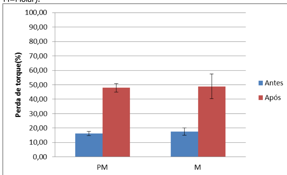
Figura 43: Perda de torque dos parafusos do Mini-Pilar (Grupo 1) antes e após ciclagem termomecânica em cada um dos pilares da prótese (PM=Pré-molar e M=Molar).
