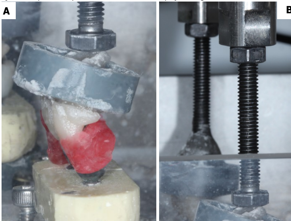
Figura 39: A - Posicionamento dos conjuntos na máquina de ensaios; B - Ajuste do parafuso para união da haste com peça antagonista.
