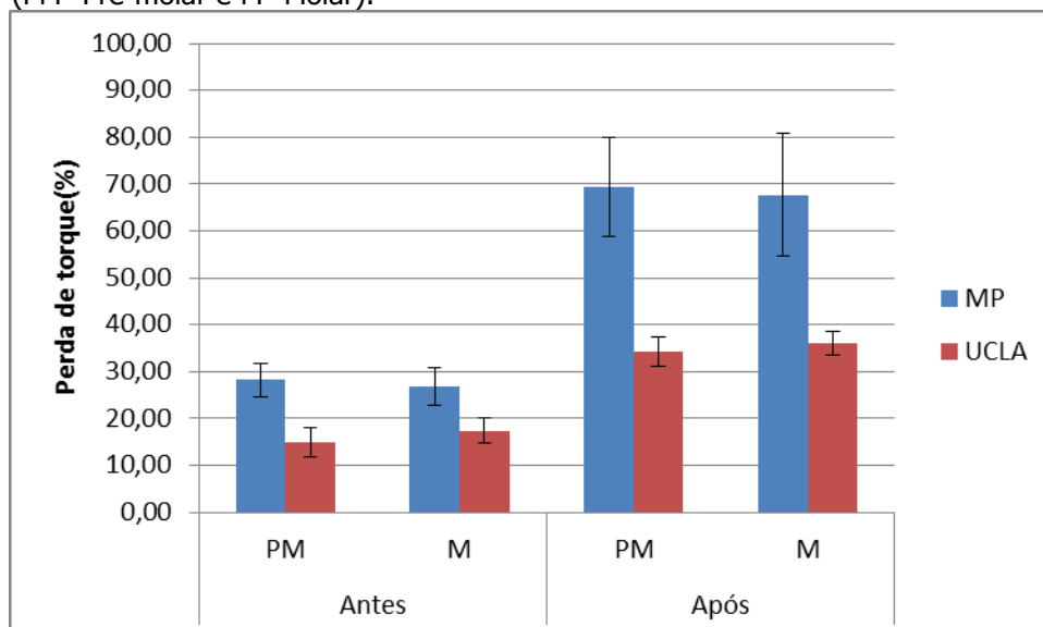
Figura 42: Perda de torque dos parafusos entre os grupos Mini-Pilar e UCLA antes e após ciclagem termomecânica em cada um dos pilares da prótese (PM=Pré-molar e M=Molar).
