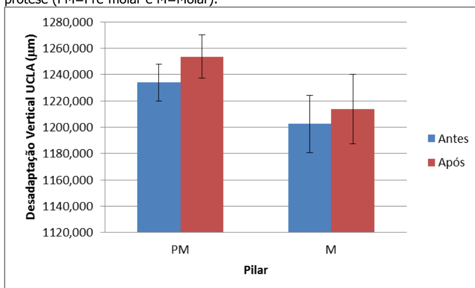
Figura 47: Desadaptação interna vertical média ( \mu\text{m} ) no grupo UCLA (interface implante/pilar), antes e após ciclagem termomecânica em cada um dos pilares da prótese (PM=Pré-molar e M=Molar).
