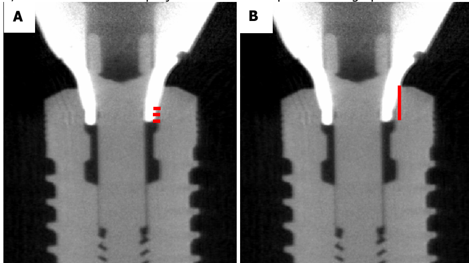
Figura 36: A - Medidas de desadaptação interna horizontal por corte no grupo 2; B - Medida de desadaptação interna vertical por corte no grupo 2.
