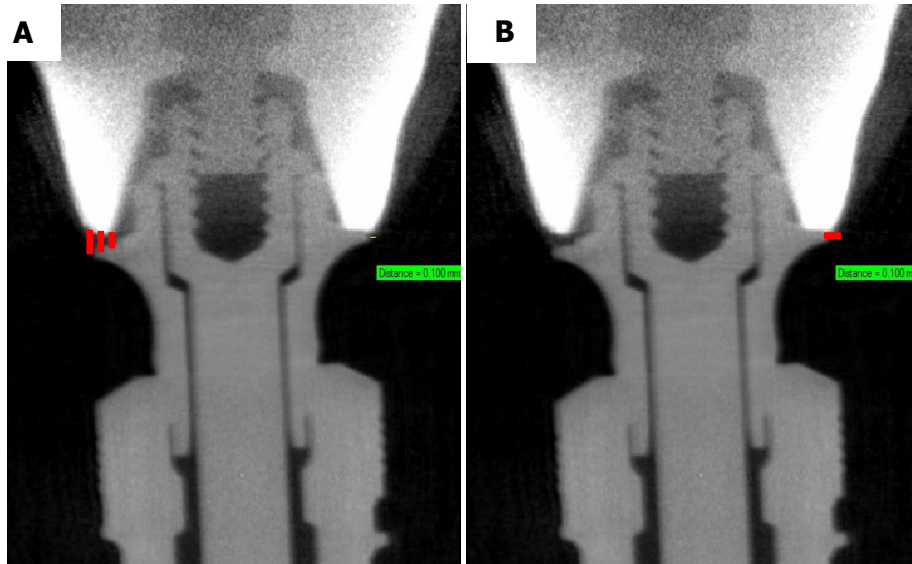
Figura 35: A - Medidas de desadaptação marginal vertical por corte no grupo 1; B - Medida de desadaptação marginal horizontal por corte no grupo 1.
