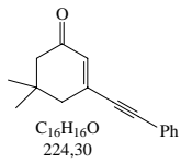
5,5-dimetil-3-(2-feniletinil)ciclohex-2-enona
