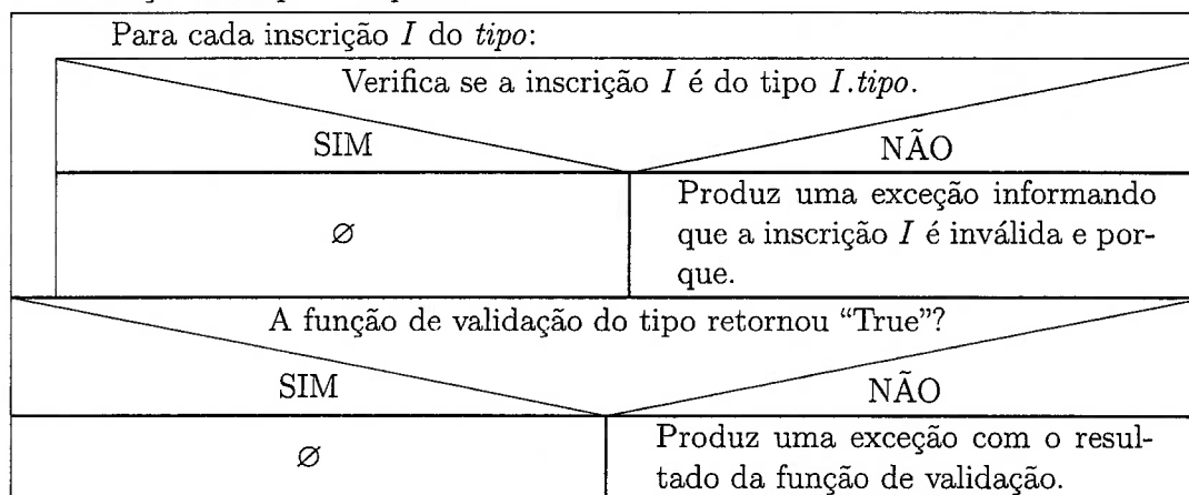
Figura 3.4: Procedimento de validação da rede (Parte II).
