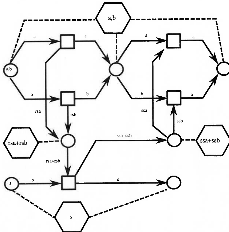
Figura 3.2: Representação gráfica de classes de cores (hexágonos) em uma rede RAC.
