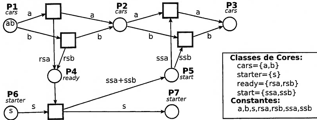
Figura 3.1: Rede arco-constante, adaptação da figura 3.3 de Girault e Valk (2003, p. 31) .
