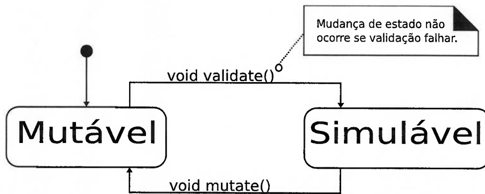
Figura 4.1: Diagrama de estados para a rede.
