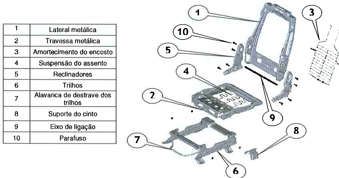
Figura 3.7 – Principais componentes de uma estrutura.
