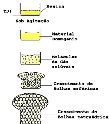
Figura 3.23 Ilustração das reações de polimerização de isocianato e polioli
