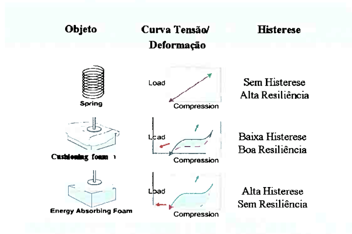
Figura 3.22 Comparação entre efeito mola e histerese
