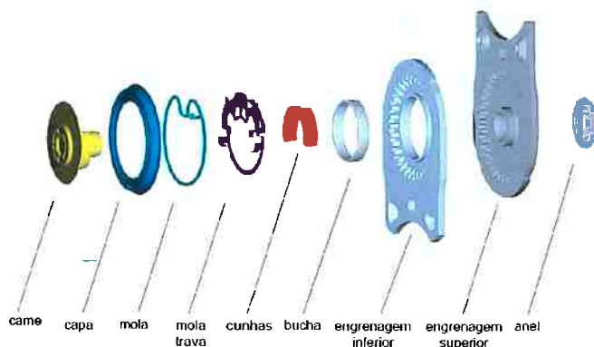
Figura 3.12 – Mecanismo infinitesimal (Modelo T2000 / Fonte: Empresa Keiper)
