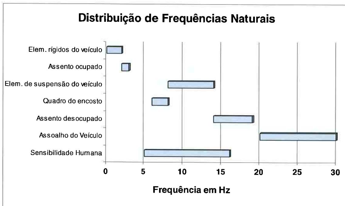
Figura 5.5 Distribuição das frequências naturais de assentos, ocupantes e veículos.
