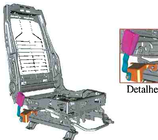
Figura 3.5 – Assento integrado.
