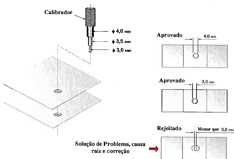
Figura 38 – Critério de aprovação do processo de pré-controle.
