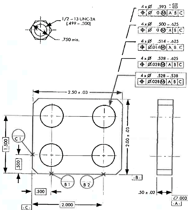
Figura 14 – Exemplos de alternativas de controle de tolerâncias.
