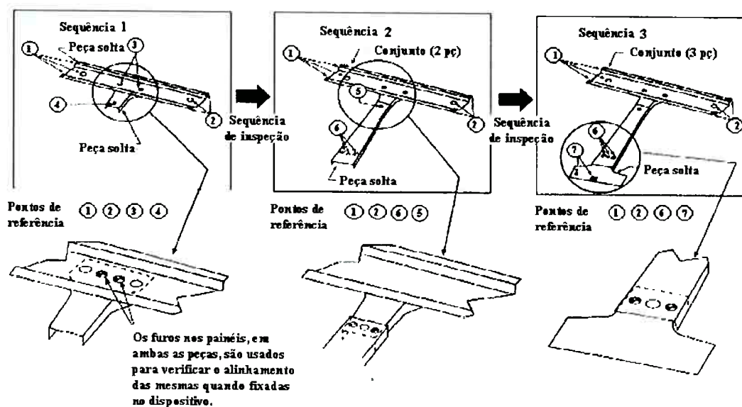
Figura 36 – Procedimento de preparação de peças padrão.
