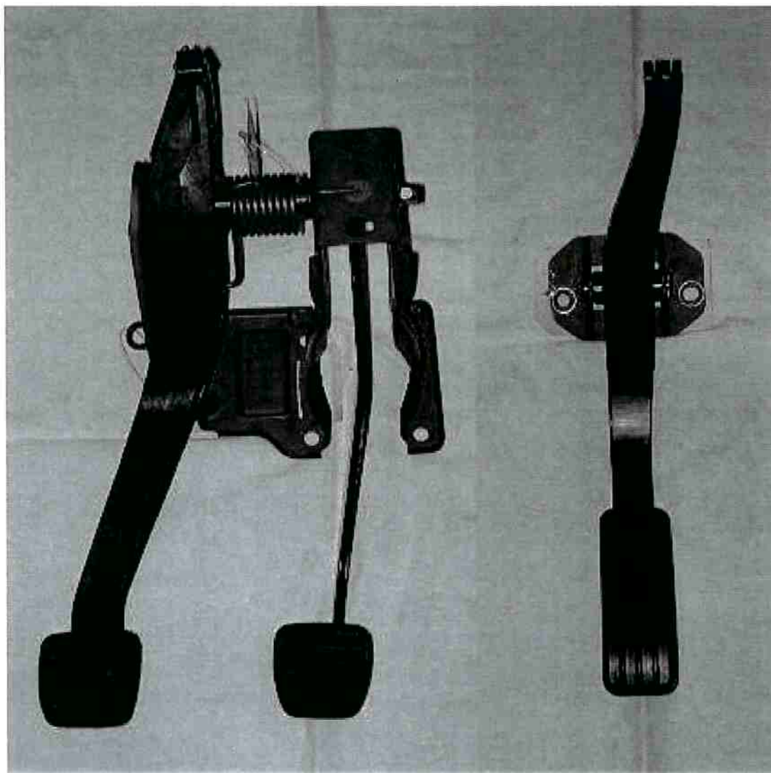
Figura 6 – Conjunto de pedais do veículo da concorrência montado.
