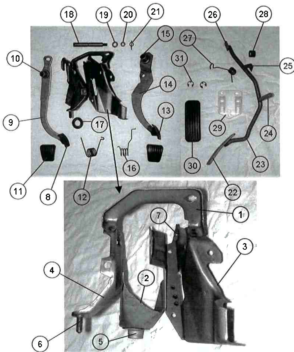
Figura 5 – Conjunto de pedais do veículo GMB desmontado.
