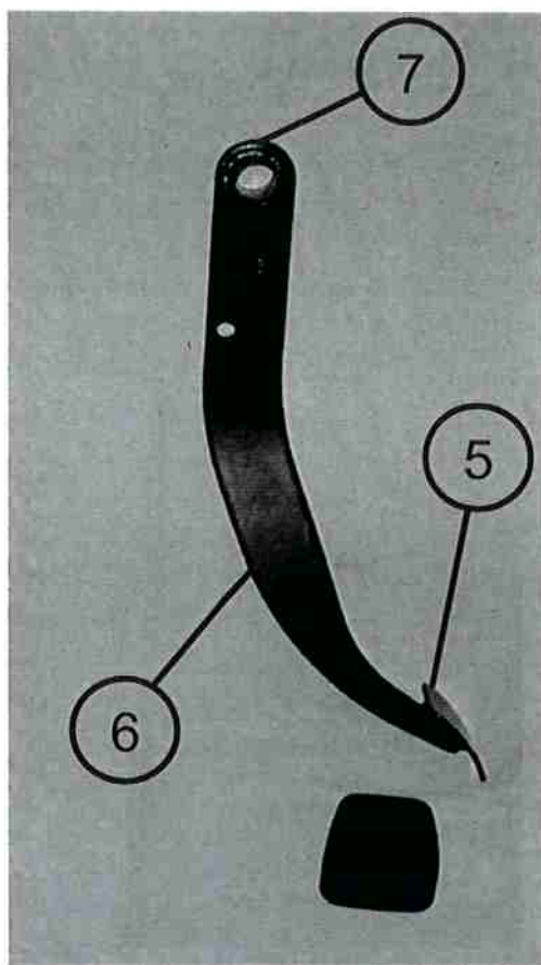
Figura 13 – Pedal do freio do veículo da concorrência.
