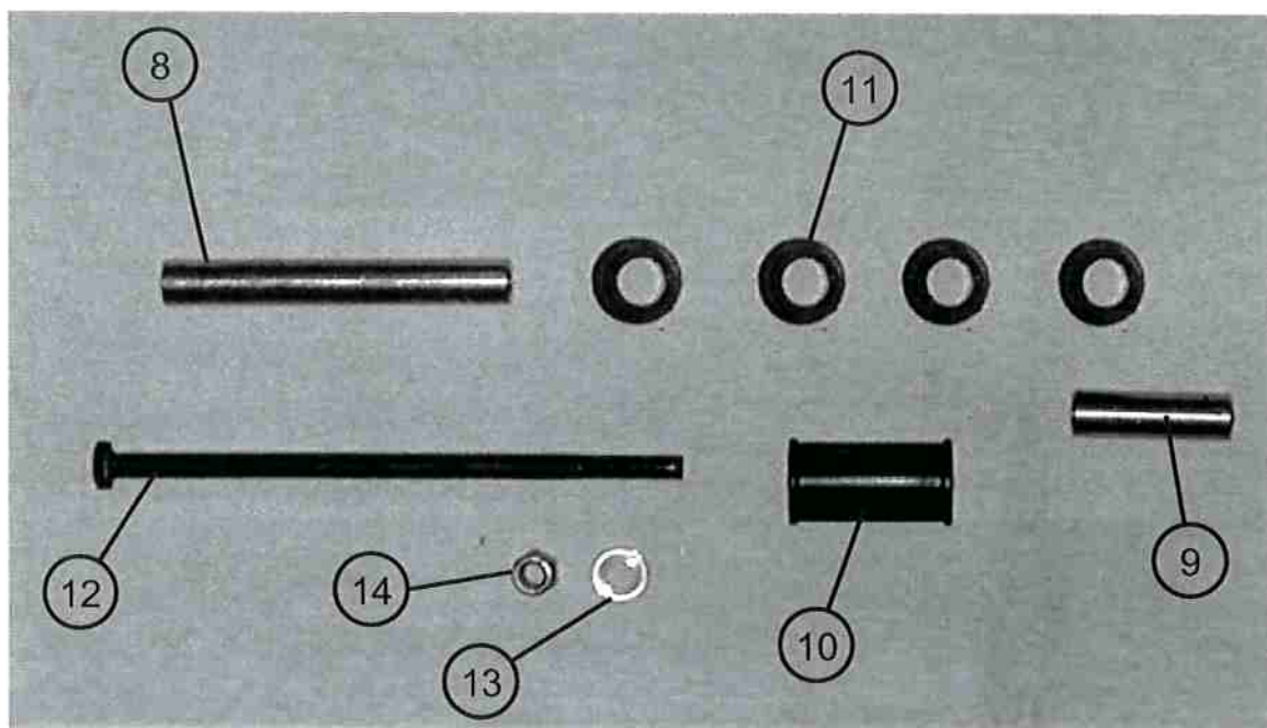
Figura 15 – Miscelâneas do veículo da concorrência.
