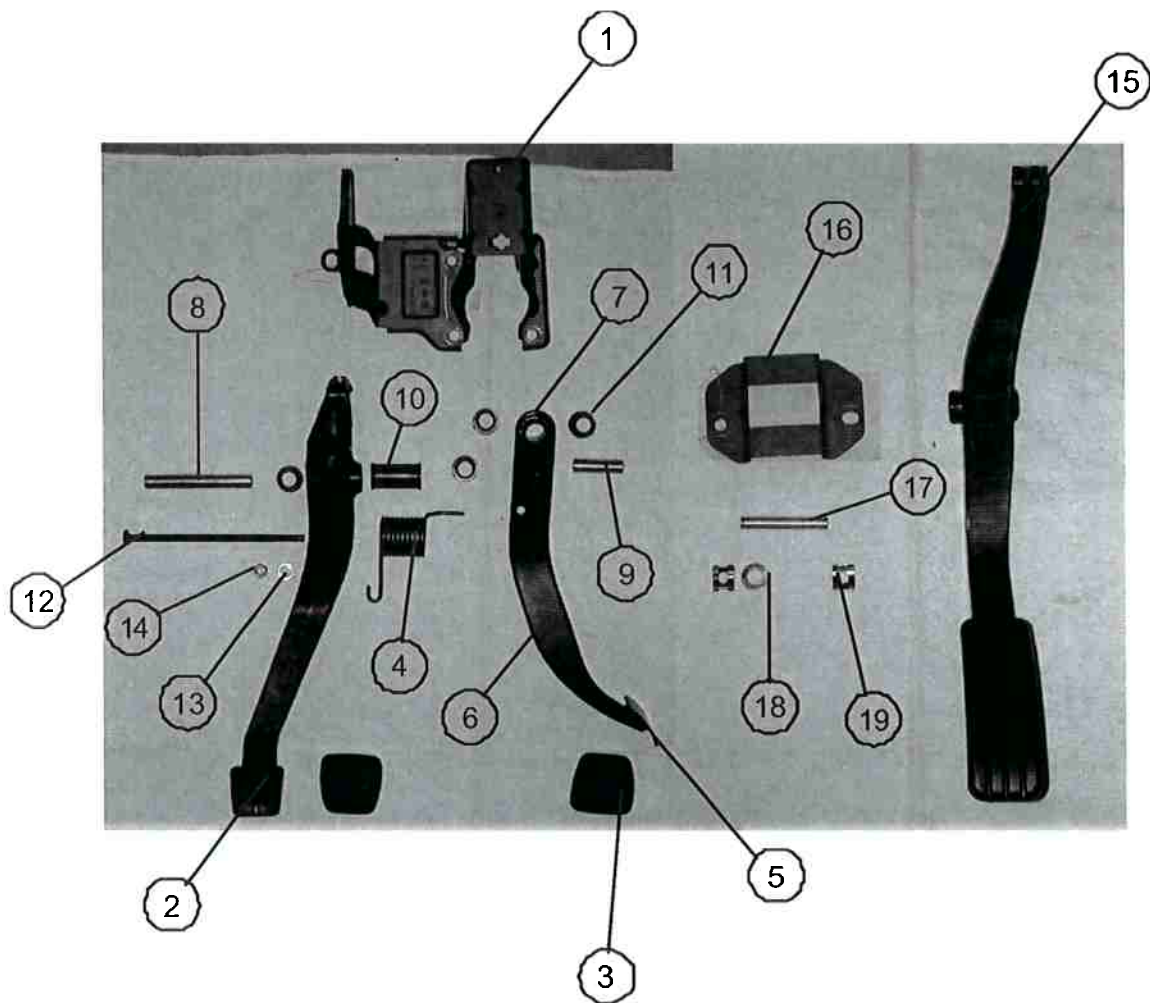
Figura 7 – Conjunto de pedais do veículo da concorrência desmontado.
