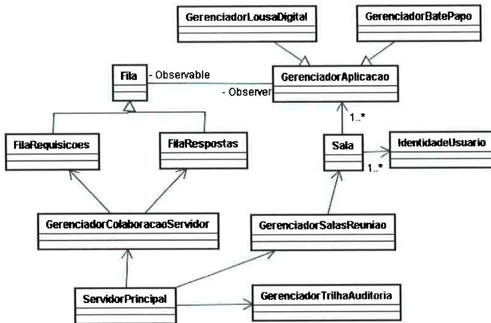
Figura 4-5 – Diagrama de classes do módulo servidor
