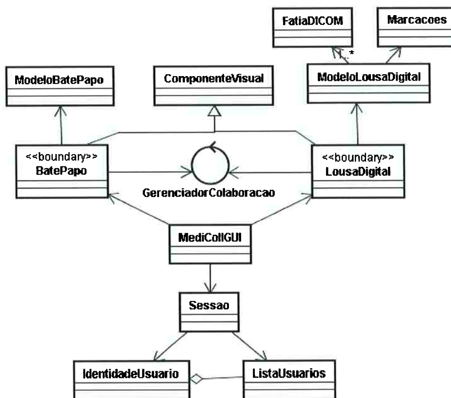
Figura 4-6 – Principais classes do módulo cliente
