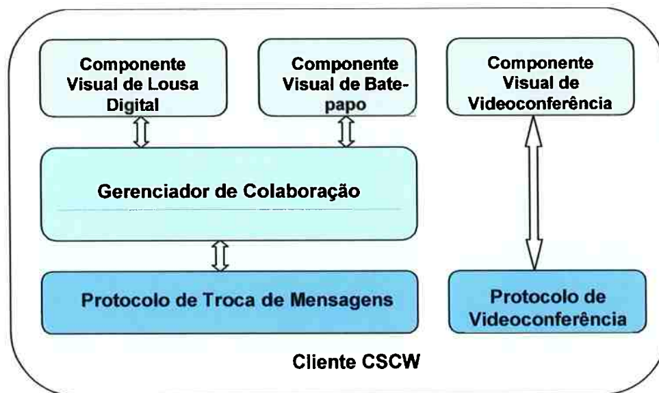
Figura 3-10 – Módulo Cliente da Aplicação
