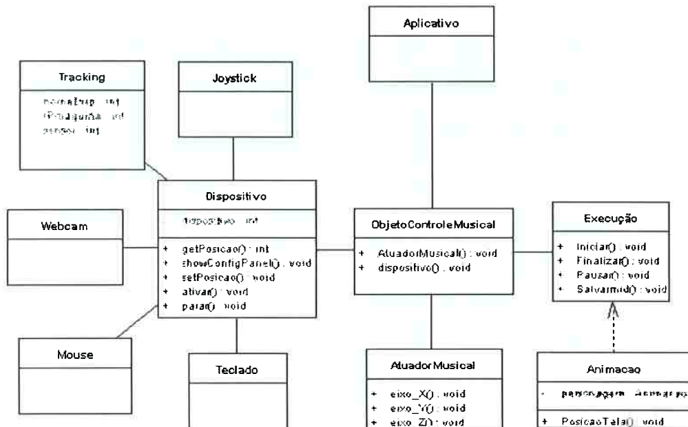
Figura 6.8: Modelo de classes de som do sistema MusandScene
