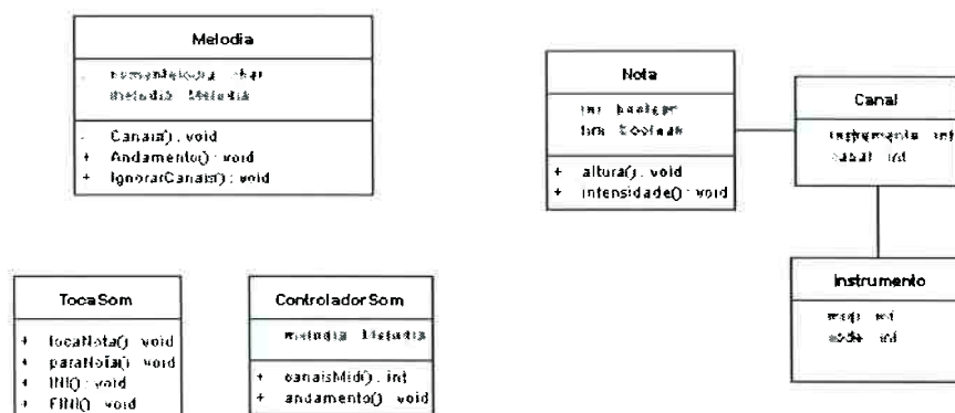
Figura 6.9: Modelo de classes do sistema MusandScene
