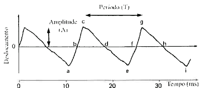
Figura 2.1: Gráfico de deslocamento temporal de uma corda Dó do violoncelo
