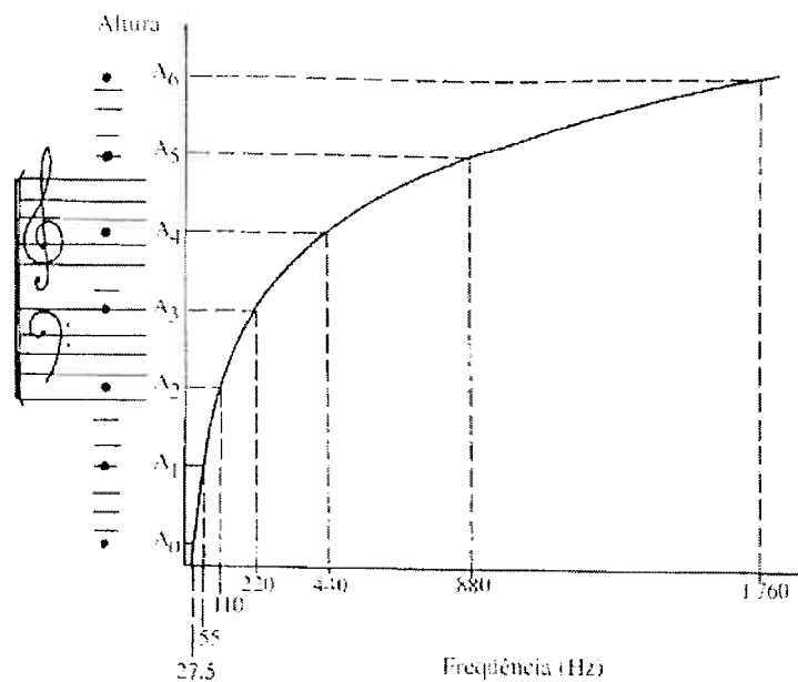
Figura 2.2: Relação entre alturas e frequências
