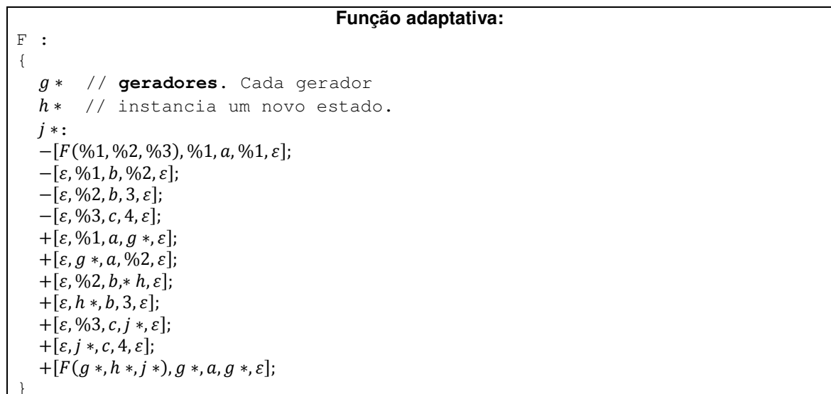
Figura 2.2 Função adaptativa F .
