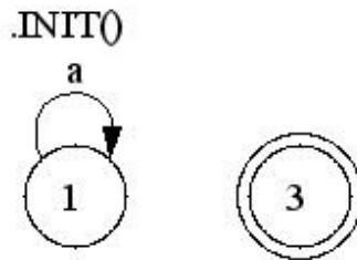
Figura 2.1 Autômato adaptativo que resolve a linguagem a^n b^n c^n . Configuração inicial.
