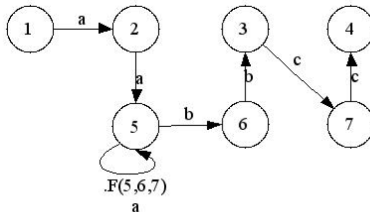
Figura 2.3 Autômato adaptativo que resolve a linguagem a^n b^n c^n . Configuração após a cadeia entrada aabbcc
