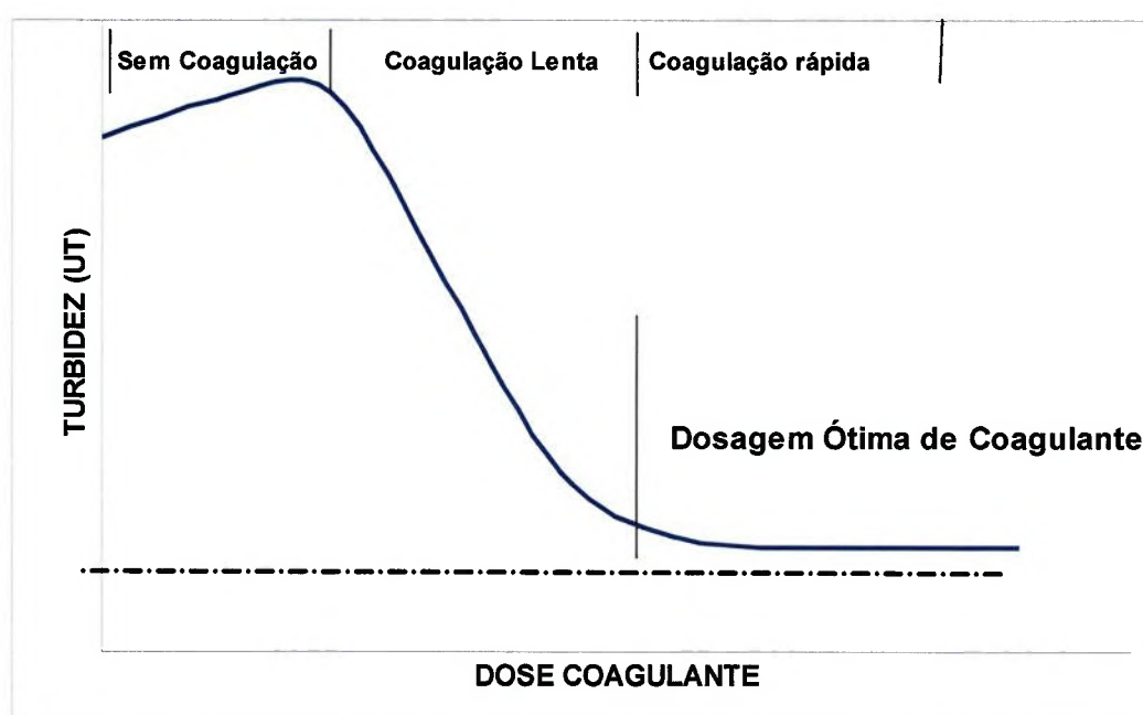
Fig. 2- Efeito da concentração de coagulante na turbidez
