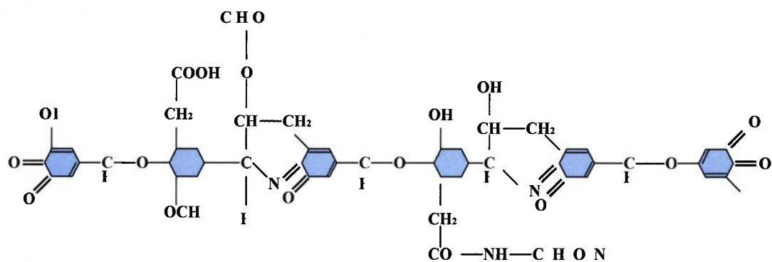
Fig. 6 - Modelo de molécula de ácido húmico
