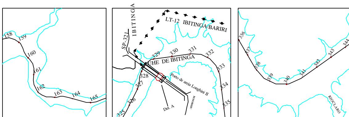
Figura B.34 – Raios de Curvatura dos Pontos Kilométricos 161-163, 331-333 e 338-340
