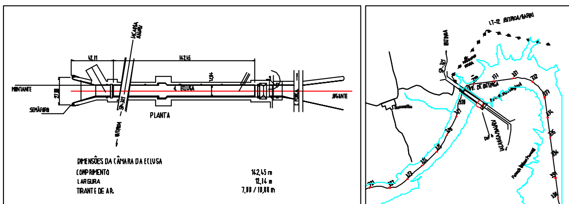
Figura B.25 - Eclusa de Ibitinga
