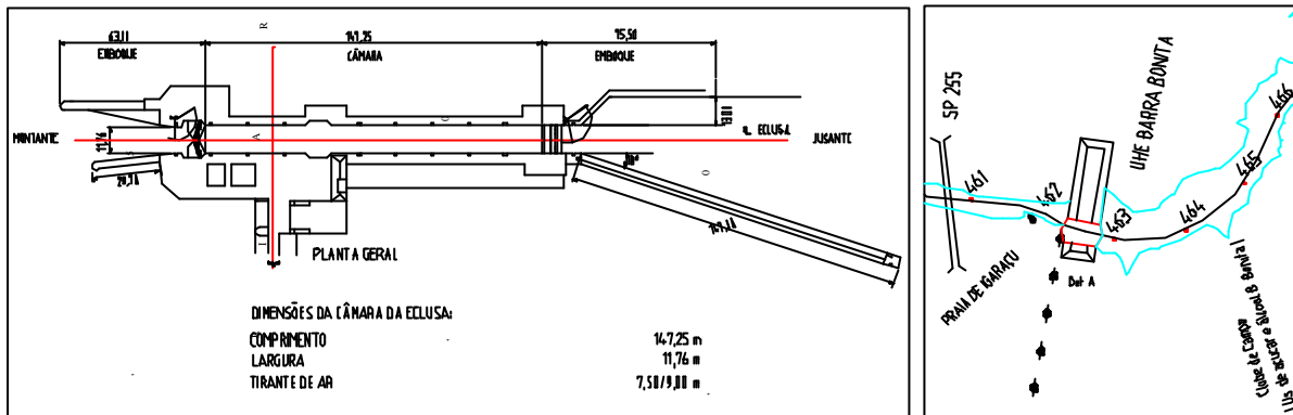
Figura B.23 - Eclusa de Barra Bonita
