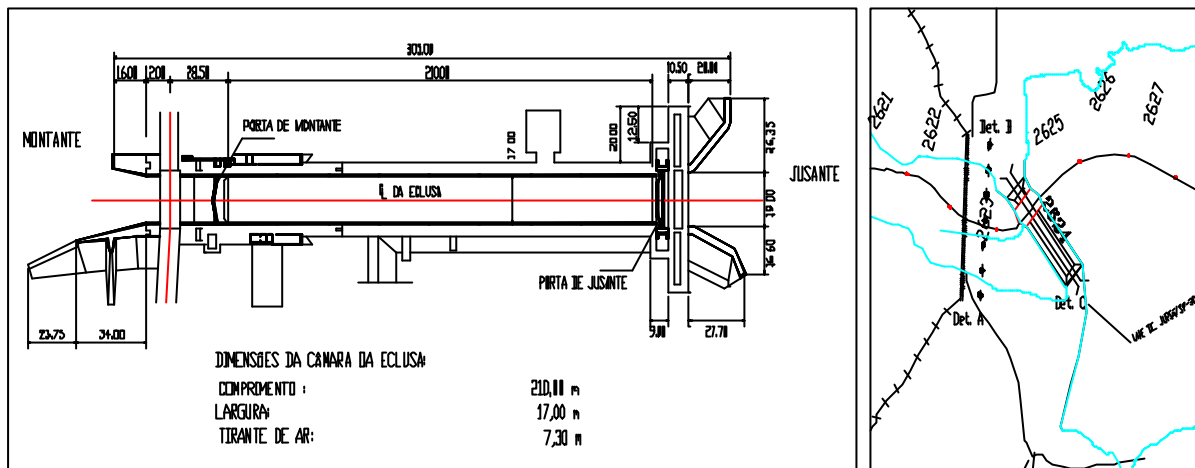
Figura B.30 - Eclusa de Jupia
