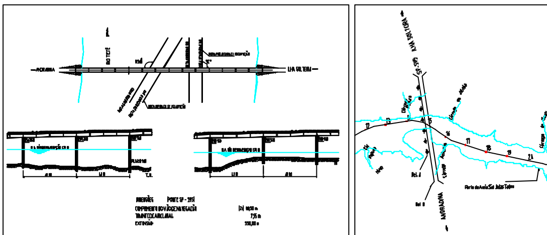
Figura B.10 - Ponte SP-595 (Ilha Solteira / Andradina)
