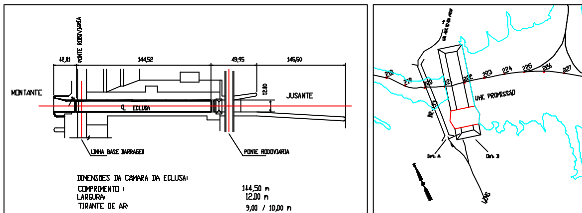
Figura B.26 - Eclusa de Promissão
