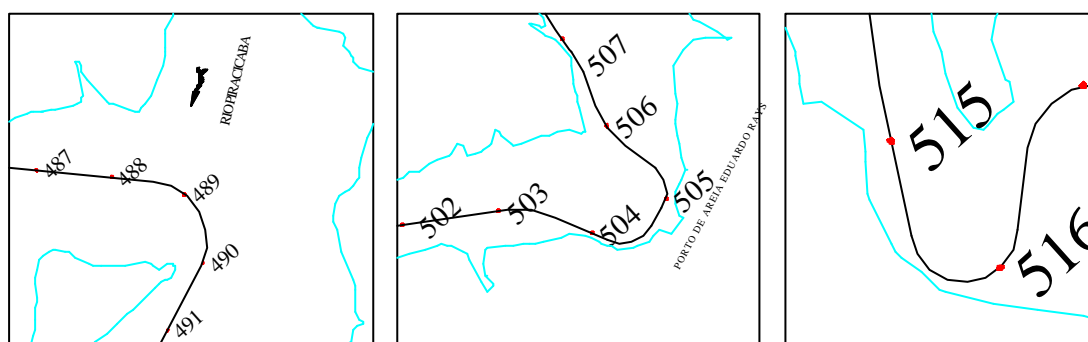
Figura B.38 – Raios de Curvatura dos Pontos Kilométricos 488-490, 504-505 e 515-516
