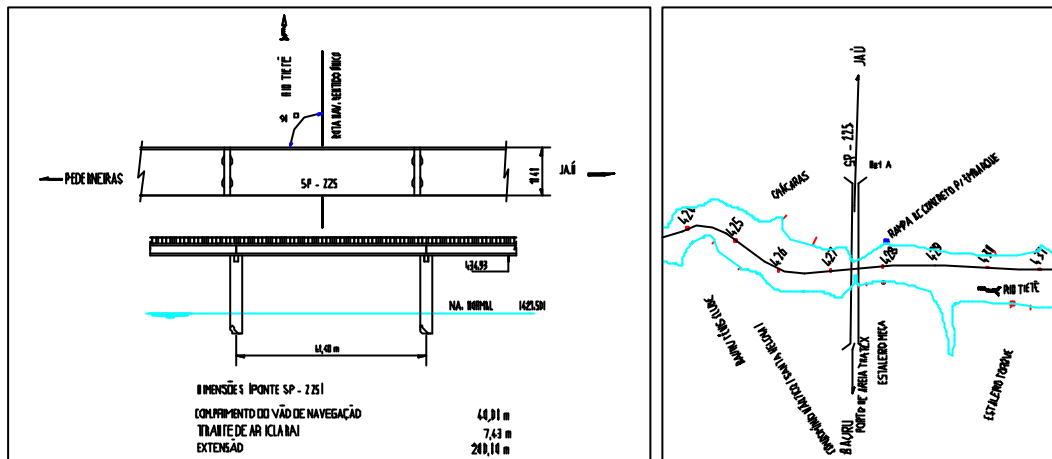
Figura B.6 - Ponte SP-225 (Pederneiras / Jaú)
