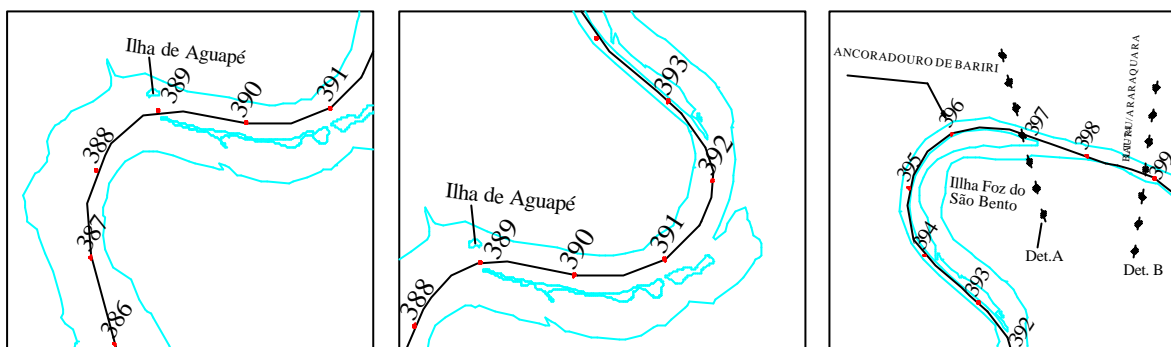
Figura B.36 – Raios de Curvatura dos Pontos Kilométricos 387-389, 391-392 e 394-396
