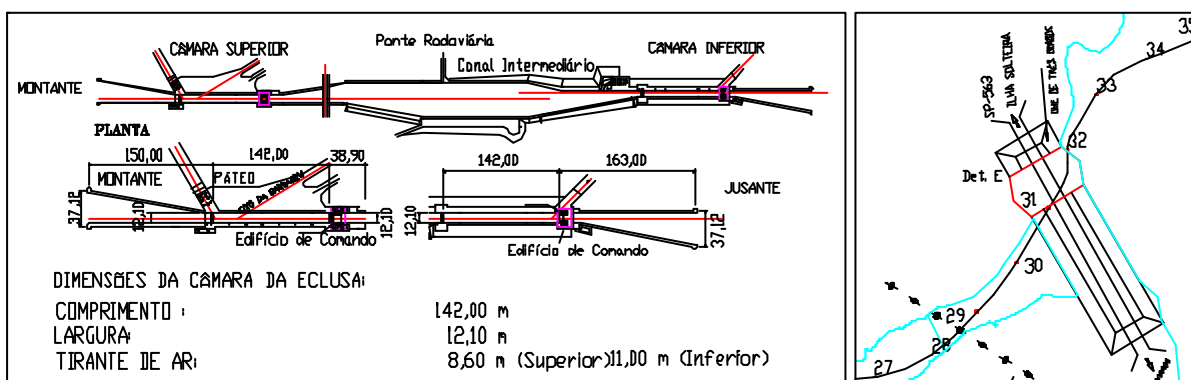
Figura B.28 - Eclusas de Três Irmãos
