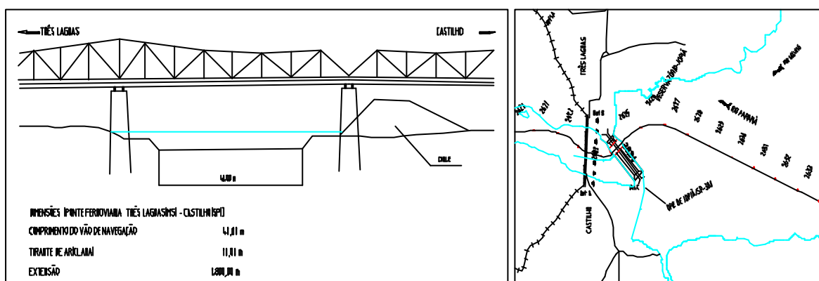
Figura B.19 - Ponte Ferroviária (Três Lagoas / Castilho)
