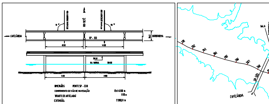
Figura B.4 - Ponte SP-333 (Cafelândia / Borborema)
