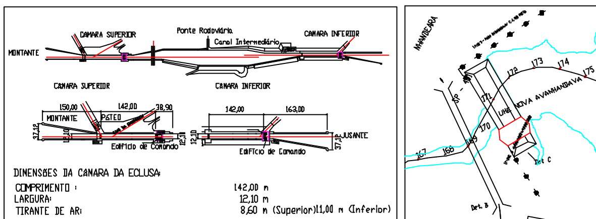
Figura B.27 - Eclusas de Nova Avanhandava
