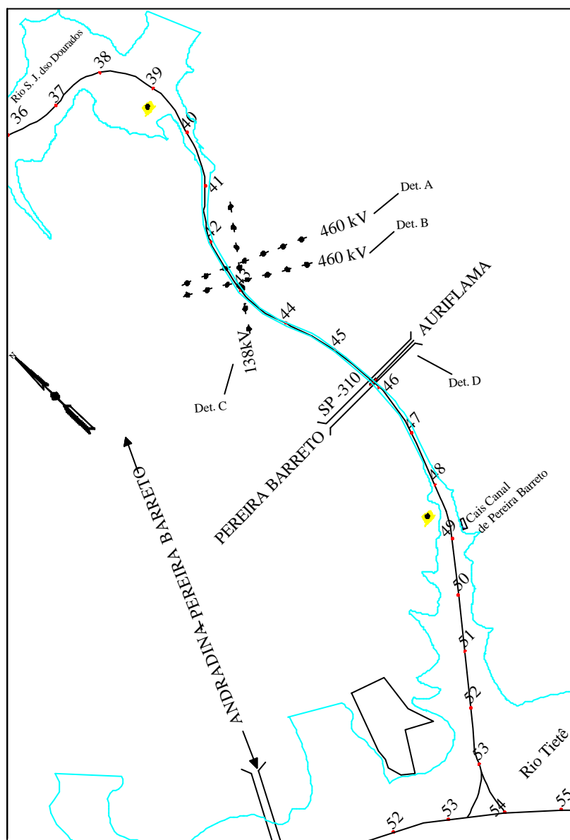
Figura B.49 – Canal de Pereira Barreto
