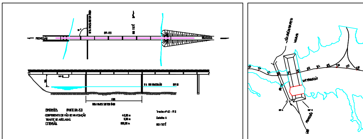
Figura B.5 - Ponte BR-153 (Promissão / Ubarana)
