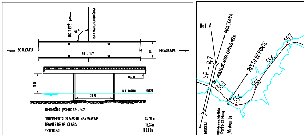
Figura B.9 - Ponte SP-147 (Botucatu / Piracicaba)
