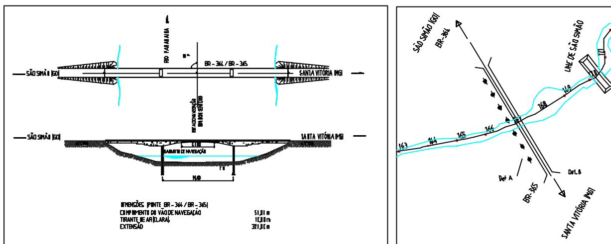
Figura B.21 - Ponte BR-365/BR-364 (Santa Vitória/São Simão)
