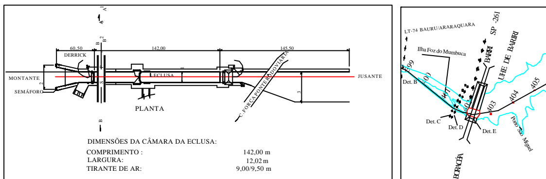
Figura B.24 - Eclusa de Bariri
