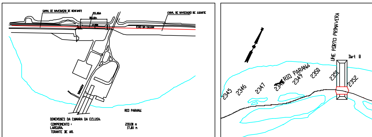
Figura B.31 - Eclusa de Primavera
