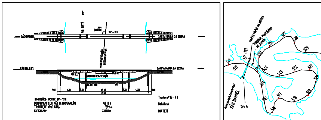
Figura B.7 - Ponte SP-191 (São Manuel / Santa Maria da Serra)
