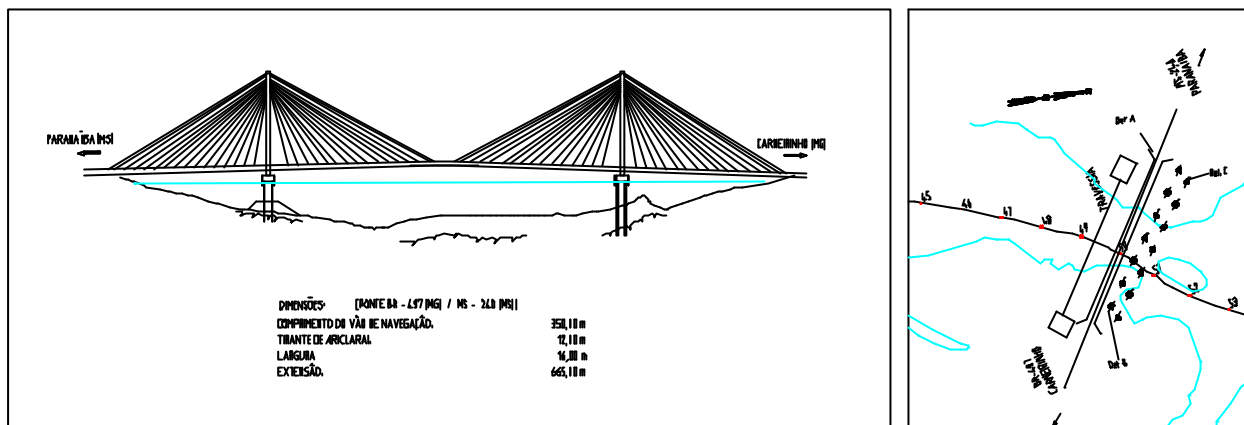
Figura B.20 - Ponte Br-497/Ms-240 (Paranaíba/Carneirinho)
