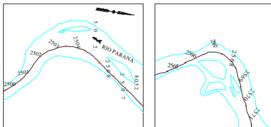
Figura B.46 – Raios de Curvatura dos Pontos Kilométricos 2501-2505 e 2566-2568
