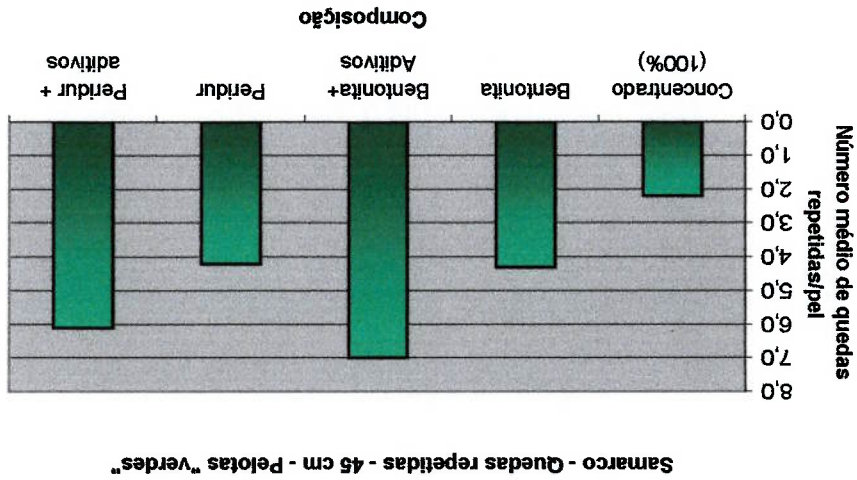
Figura 18 – Resultados de resistência a quedas a Concentrado Samarco
