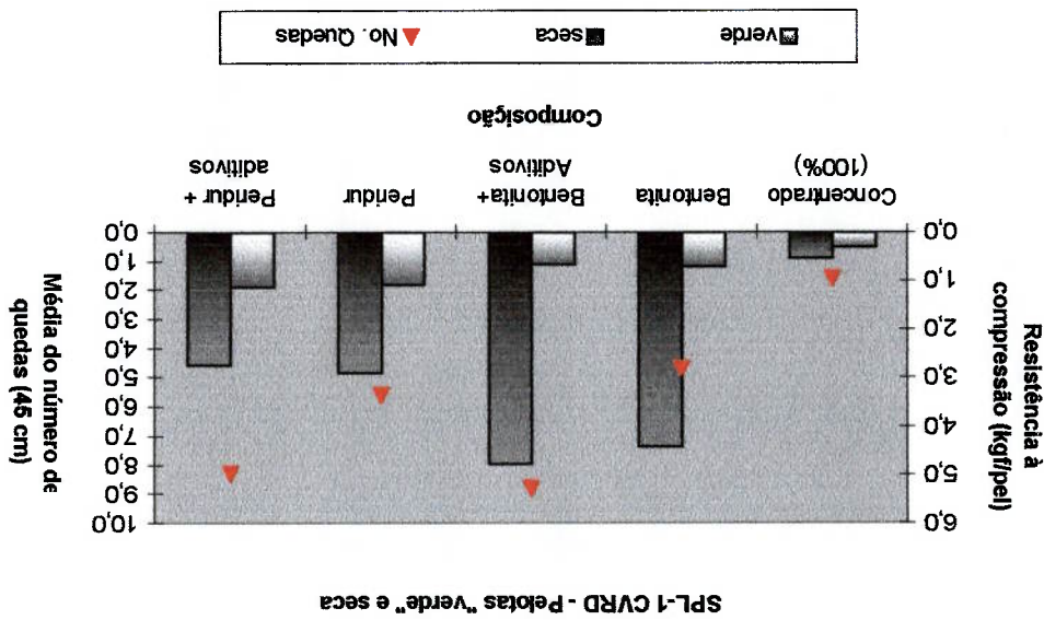
Figura 23 – Resultados obtidos com as pelotas “verde” e seca – Concentrado SPL-1
