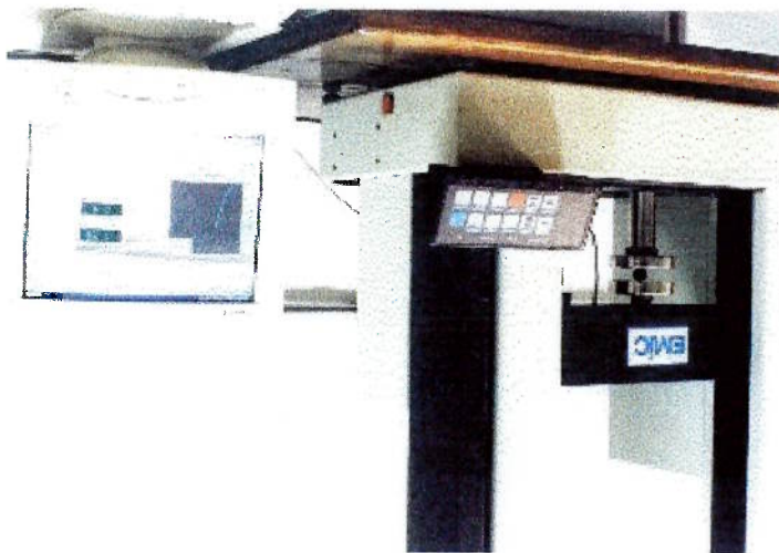
Figura 14 – Máquina Universal de Ensaios para ensaios de resistência à compressão
