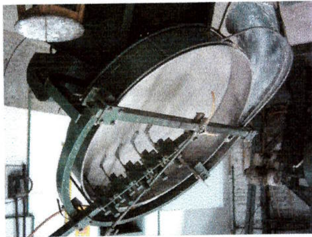
Figura 9 – Disco de pelotização utilizado nos ensaios
