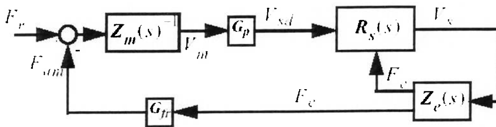
Fig.2.6 Medição direta de força(em Flemmer(1999))
