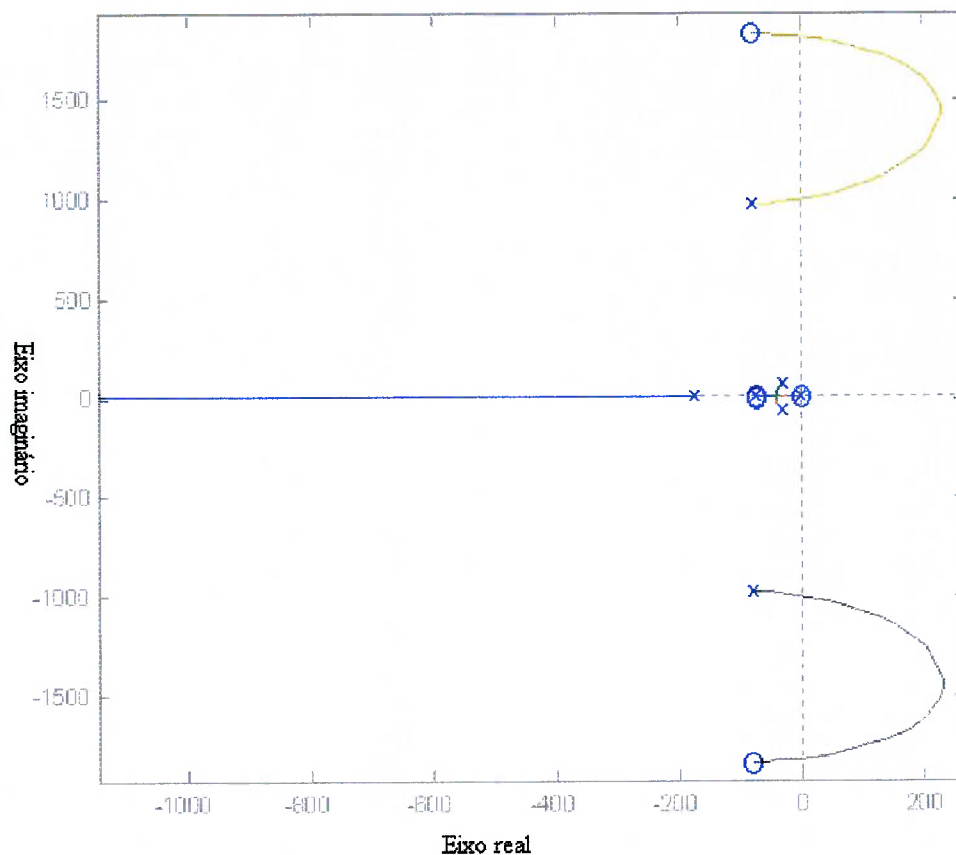
Fig.5.4 Lugar das raízes(medição direta de força com G_{fr} = 150, G_p = 1 )
