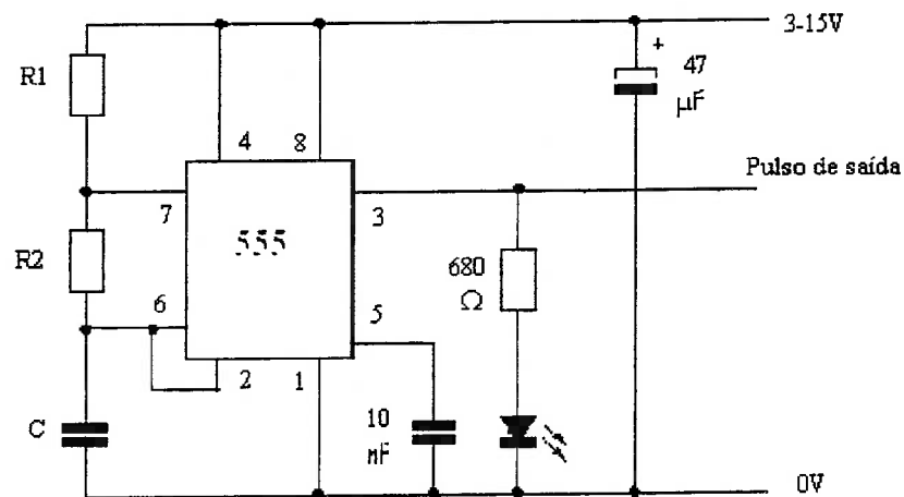
Fig.3.4 Circuito oscilador
