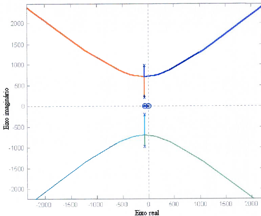
Fig.6.3 Lugar das raízes para o sistema G(s)
