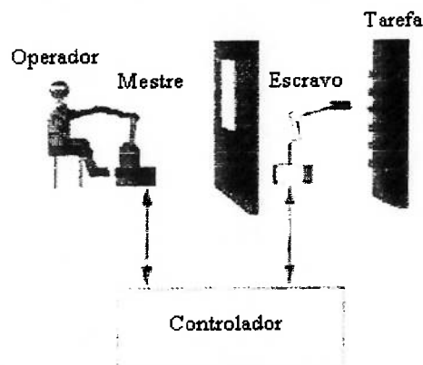
Fig.1.2 Sistema de teleoperação mestre-escravo(em Townsend et al,1999).
