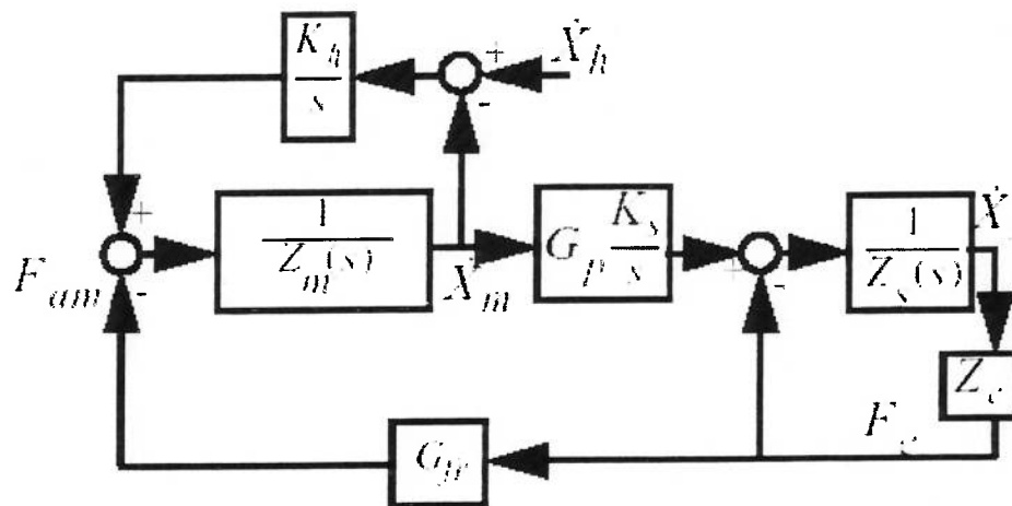
Fig.6.2 Medição direta de força(em Flemmer(1998))
