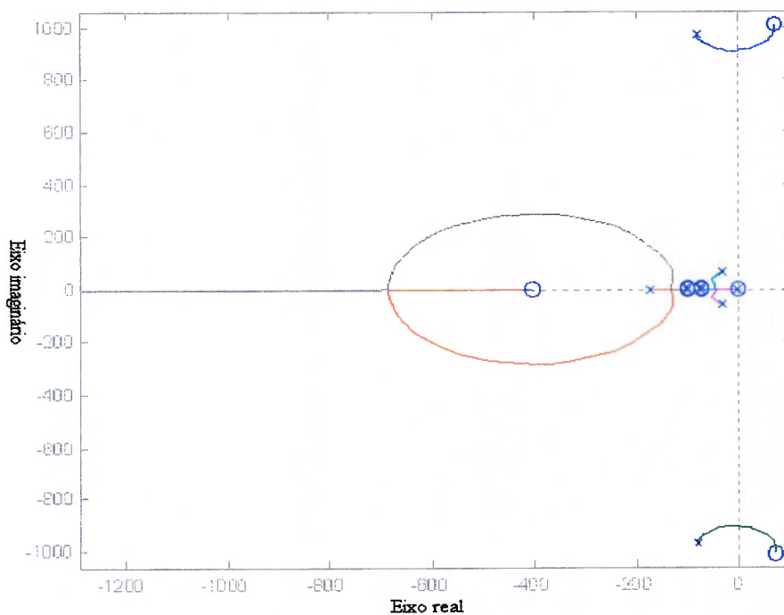
Fig.5.6 Lugar das raízes(medição direta modificada)
