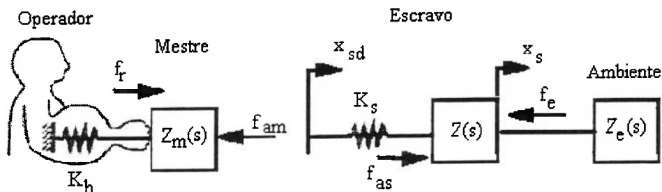
Fig.2.2 Modelagem do sistema
