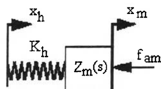
Fig.4.5 Modelo dinâmico (mestre e operador humano)
