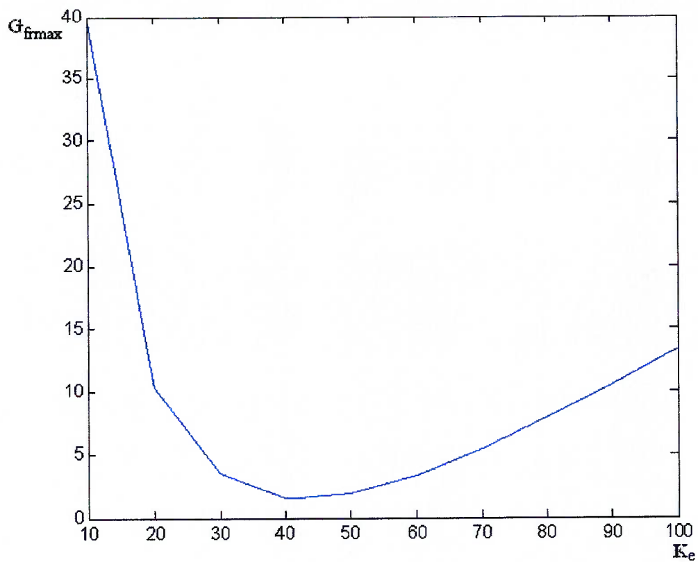
Fig.6.4 Gráfico G_{fr\max} versus K_e
