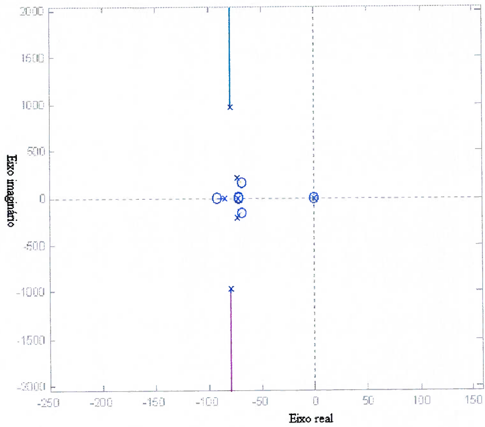
Fig.5.9 Lugar das raízes(erro de posição com Z_e = \frac{2}{s} )
