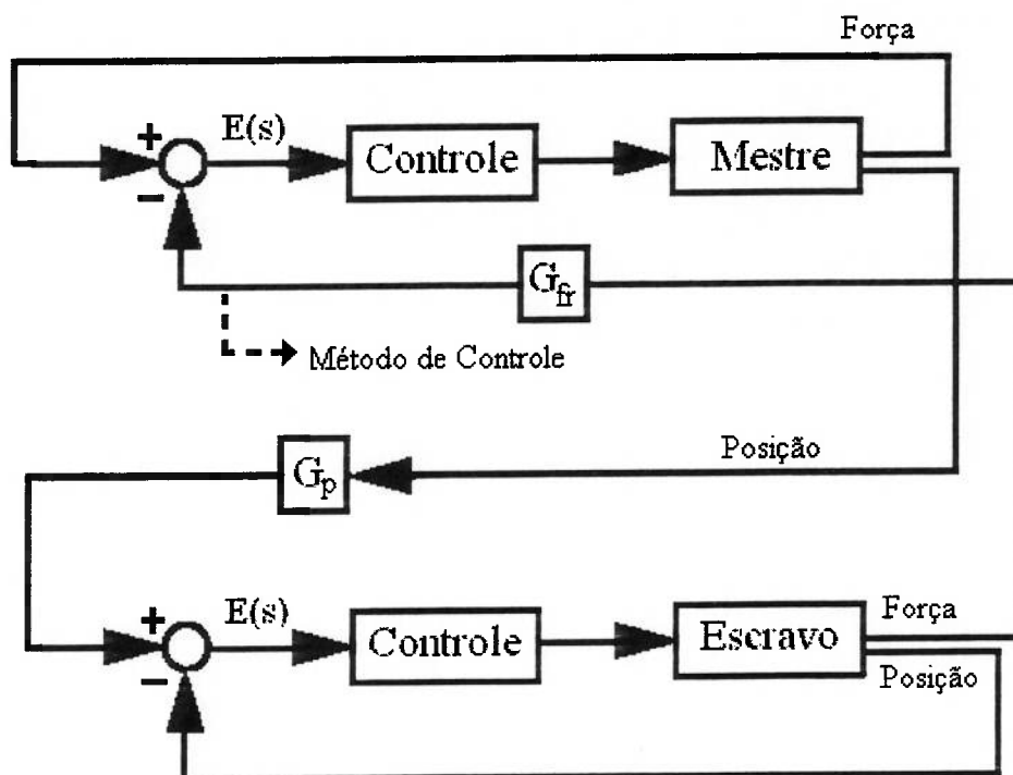
Fig.2.1 Estratégia de controle
