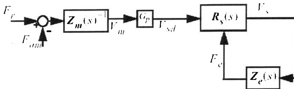
Fig.2.5 Modelo do sistema de teleoperação
