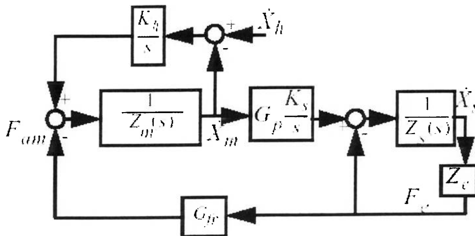
Fig.5.1 Medição direta de força (em Flemmer(1998))
