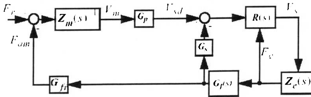
Fig.2.8 Medição direta modificada.(em Flemmer(1999))
