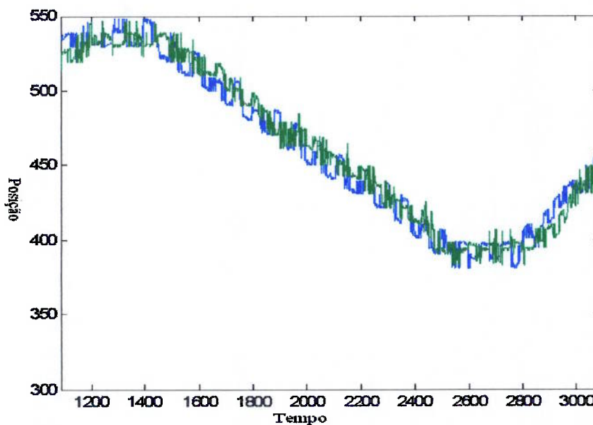
Fig.7.1 Comportamento genérico de um sistema de teleoperação utilizando motores com redução com mestre em azul e escravo em verde
