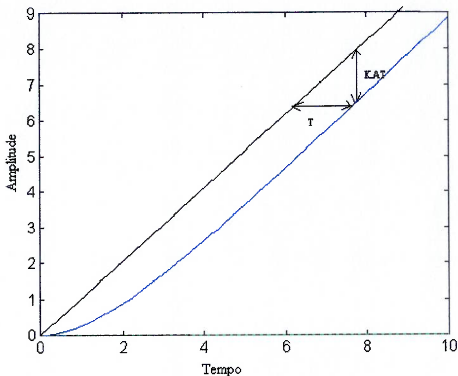
Fig.4.1 Determinação gráfica de K e T
