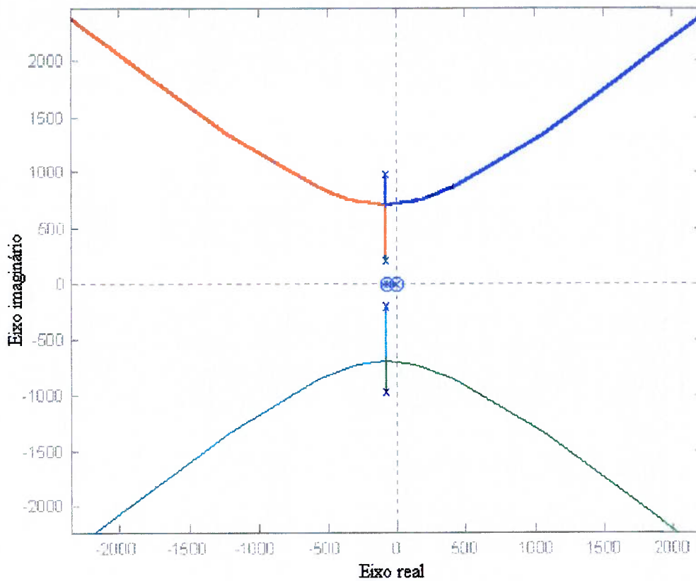
Fig.5.8 Lugar das raízes(medição direta com Z_e = \frac{2}{s} )
