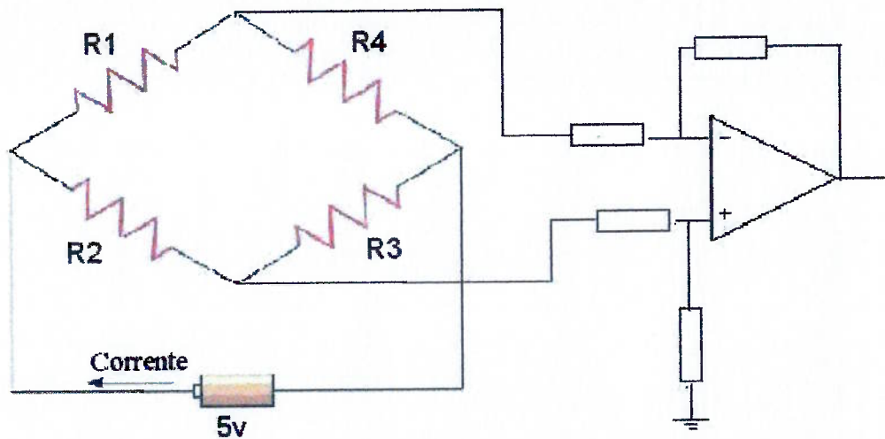
Fig.3.2 Ponte de Wheatstone e amplificador
