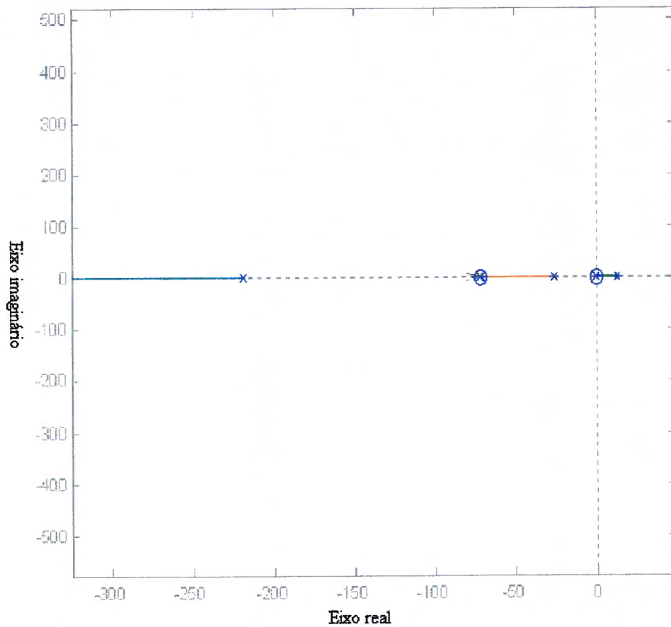
Fig.5.5 Lugar das raízes (erro de posição com G_{fr} = 150 e G_p = 1 )
