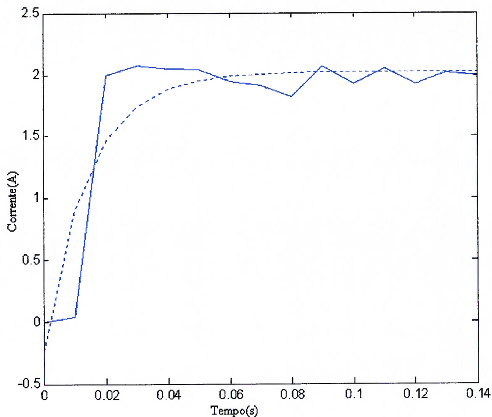
Fig.4.4 Resposta à entrada degrau
