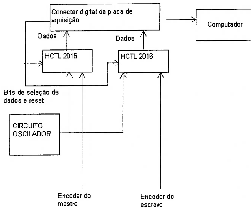
Fig.3.3 Circuito de interfaceamento dos encoders.
