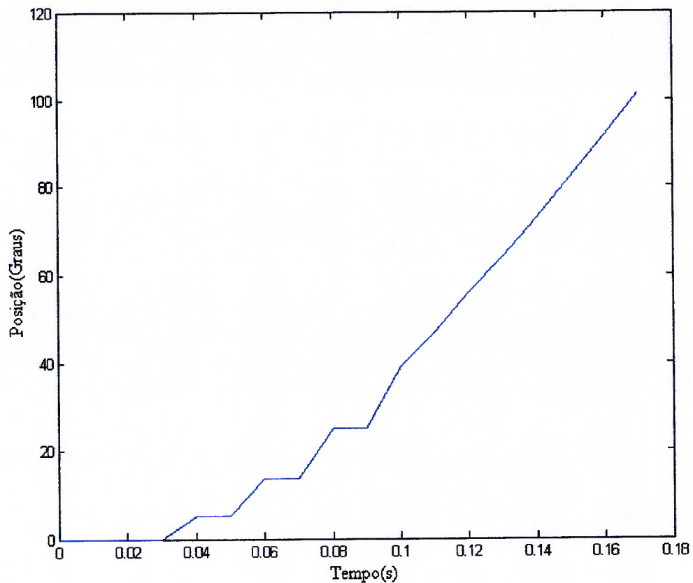
Fig.4.2 Resposta à entrada degrau
