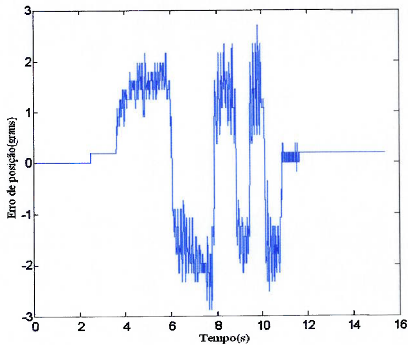
Fig.7.3 Erro de posição em graus
