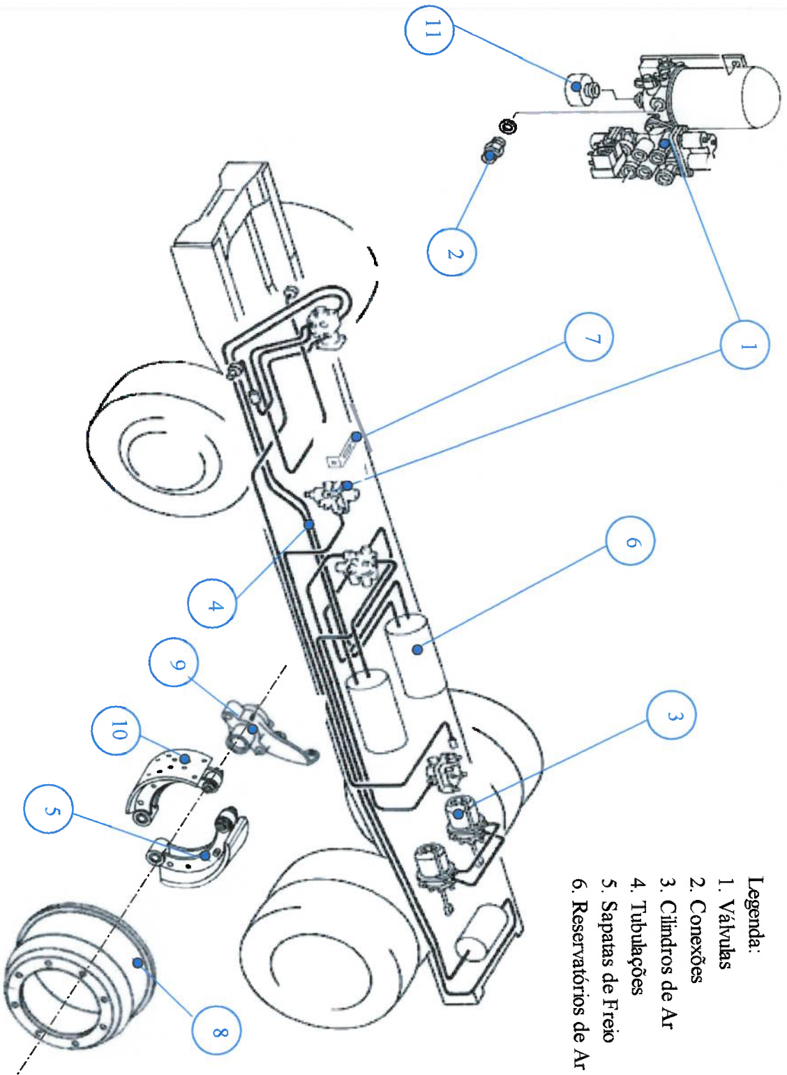
Figura 14. Esquema do Sistema de Freio a Ar acionado por Tambores.
