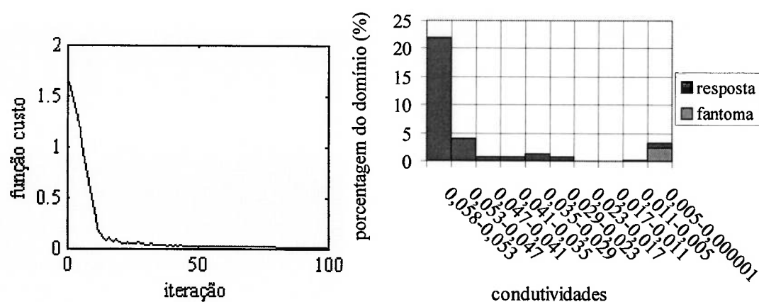
Figura 43 Curva de convergência e gráfico da porcentagem de elementos para cada faixa de valores das variáveis de projeto, ambos referentes à Figura 42. Há RS e restrição de 35% à variação das constantes de eletrodo. Valor mínimo: 0,009871.
