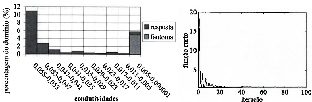
Figura 72 Curva de convergência e gráfico da porcentagem de elementos para cada faixa de valores das condutividades, ambos referentes à Figura 71. Valor mínimo: 0,628354.
