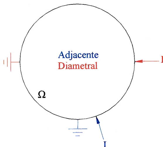
Figura 22 Padrões de excitação diametral e adjacente.
