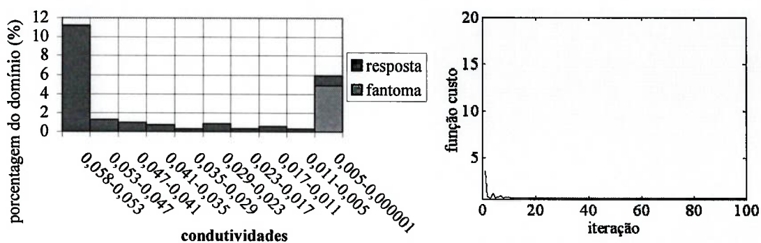
Figura 60 Curva de convergência e gráfico da porcentagem de elementos para cada faixa de valores das condutividades, ambos referentes à Figura 59. Valor mínimo: 0,615368.
