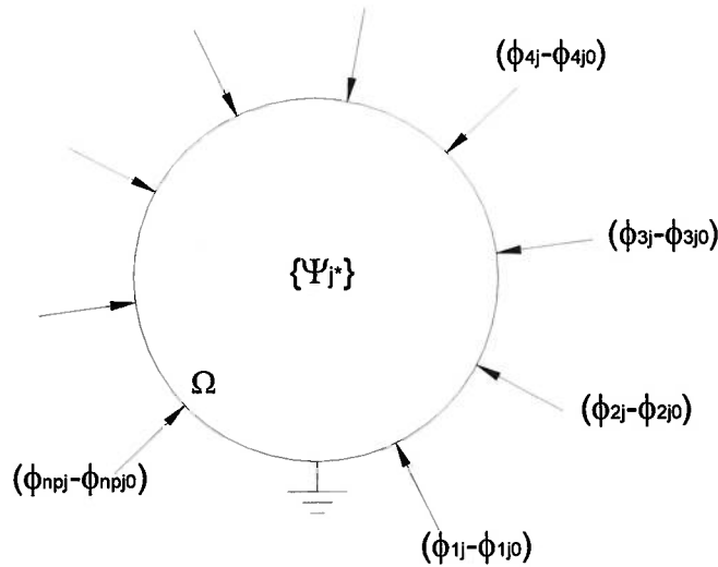
Figura 19 Aplicação de \{\Phi_j\} , com i de 1 a np , todas as correntes ao mesmo tempo. Obtém-se a distribuição \{\Psi_j^*\} .
