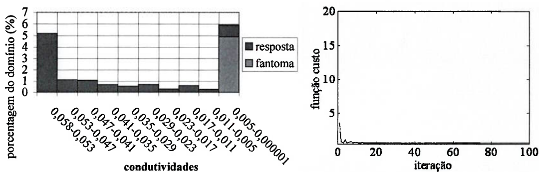
Figura 62 Curva de convergência e gráfico da porcentagem de elementos para cada faixa de valores das condutividades, ambos referentes à Figura 61. Valor mínimo: 0,615886.
