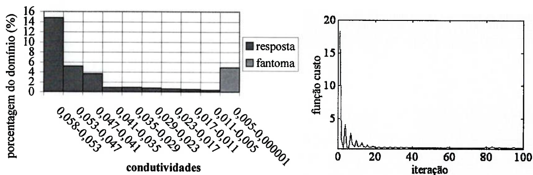
Figura 76 Curva de convergência e gráfico da porcentagem de elementos para cada faixa de valores das condutividades, ambos referentes à Figura 75. Valor mínimo: 0,728196.
