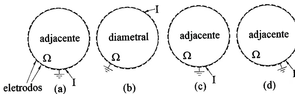
Figura 2 Os eletrodos são mostrados no contorno do domínio \Omega . (a) Padrão adjacente de excitação. (b) Padrão diametral de excitação. (c) e (d) Dois casos de carregamento diferentes para um mesmo padrão de excitação.
