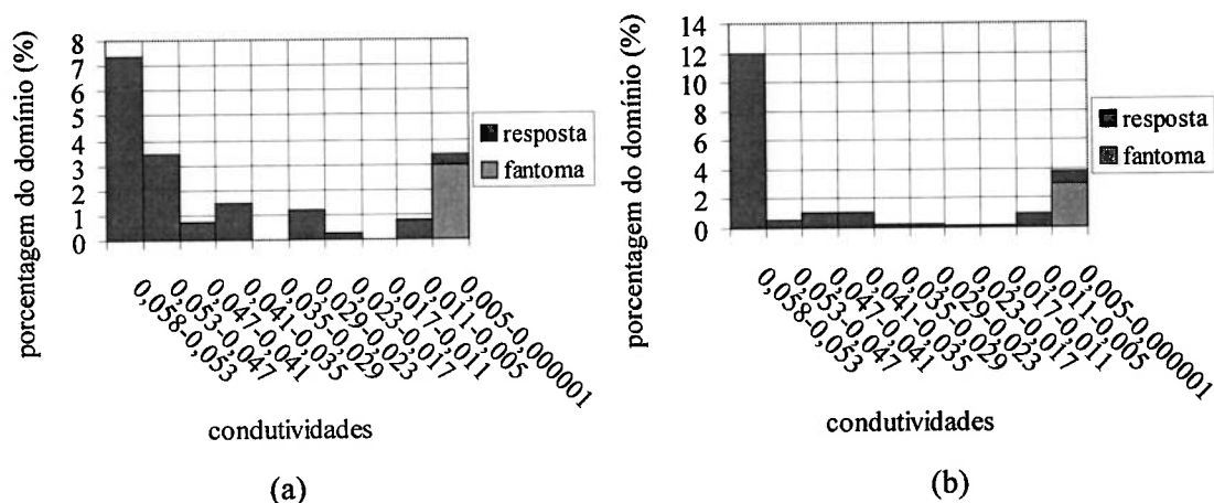
Figura 30 Gráficos da porcentagem de elementos para cada faixa de valores das variáveis de projeto. (a) Referente à Figura 21. (b) Referente à Figura 22.
