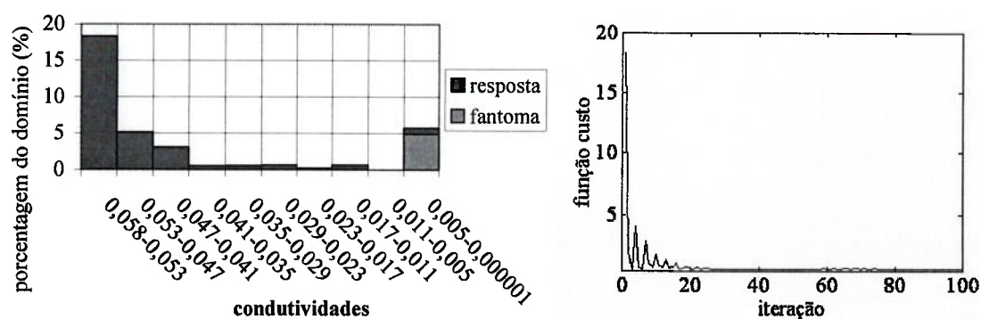
Figura 74 Curva de convergência e gráfico da porcentagem de elementos para cada faixa de valores das condutividades, ambos referentes à Figura 73. Valor mínimo: 0,647476.
