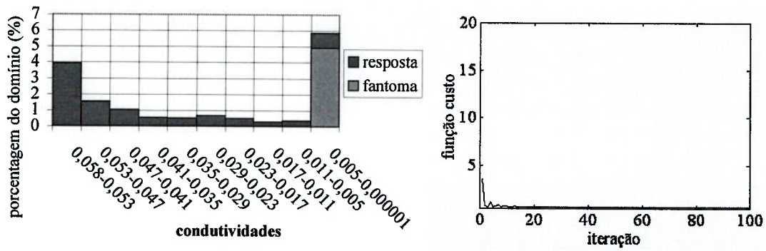
Figura 64 Curva de convergência e gráfico da porcentagem de elementos para cada faixa de valores das condutividades, ambos referentes à Figura 63. Valor mínimo: 0,616282.
