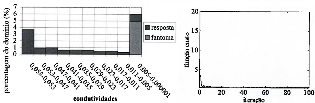
Figura 80 Curva de convergência e gráfico da porcentagem de elementos para cada faixa de valores das condutividades, ambos referentes à Figura 79. Valor mínimo: 0,618546.
