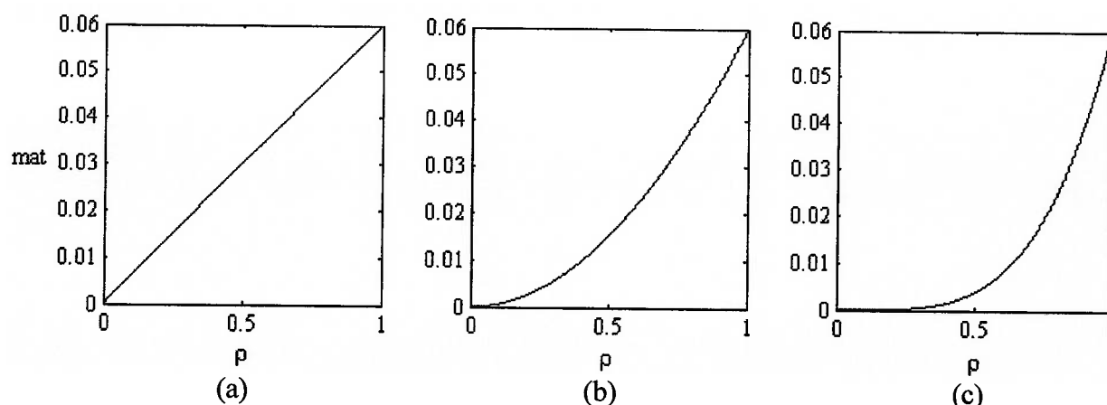
Figura 10 Gráficos de mat \times \rho para diferentes valores de p . Os valores de mat_A e mat_B usados foram 0,000001 e 0,06, respectivamente. (a) p=1 . (b) p=2 . (c) p=4 .
