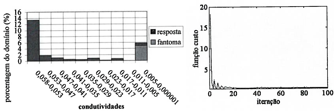
Figura 93 Curva de convergência e gráfico da porcentagem de elementos para cada faixa de valores das condutividades, ambos referentes à Figura 92. Valor mínimo: 0,617844.
