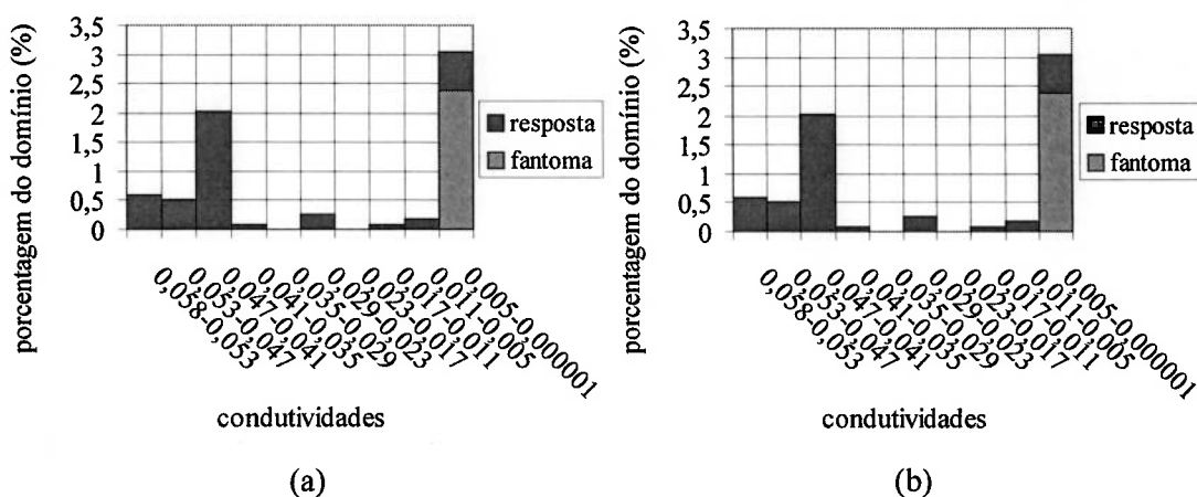
Figura 41 Gráficos da porcentagem de elementos para cada faixa de valores das variáveis de projeto. (a) Referente à Figura 38. (b) Referente à Figura 39.
