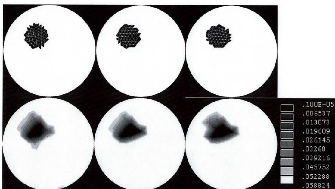
Figura 59 “Fantoma” numérico e resposta encontrada. Neste caso, p=1 e o raio do filtro é 0,005m.
