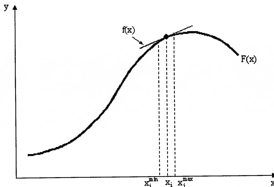
Figura 16 Função não linear F(x) e sua linearização f(x) em torno de x_i . O índice i indica a i -ésima iteração.
