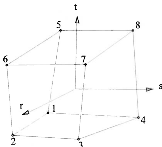
Figura 4 Elemento finito hexaédrico e suas coordenadas locais. As coordenadas variam de -1 a 1 .
