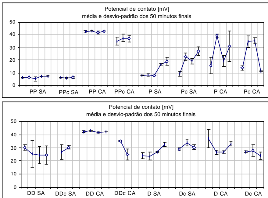
Valores médios do potencial de contato, resultante dos ensaios oscilatórios (gráfico superior) e rotativos (gráfico inferior).
