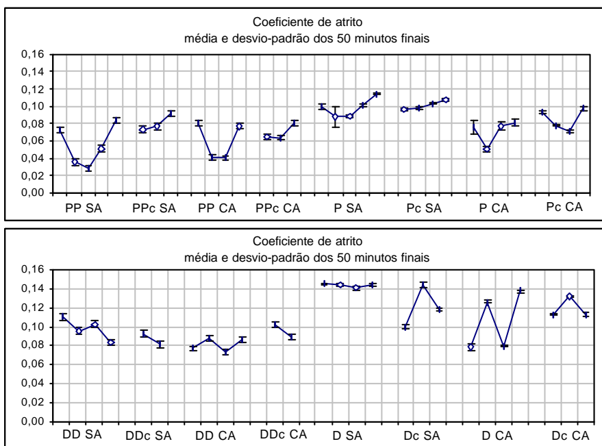
Valores médios do coeficiente de atrito, resultante dos ensaios oscilatórios (gráfico superior) e rotativos (gráfico inferior).
