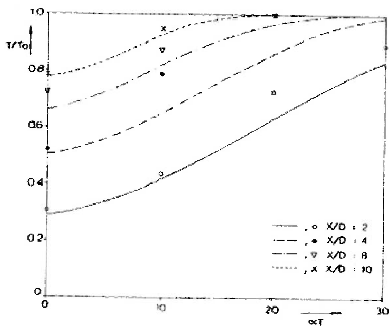
Figura 3.19b – Degradação dos propulsores quando submetidos a interferência, em função do ângulo de azimute (extraído de DIJK, AALBERS, 2001).
