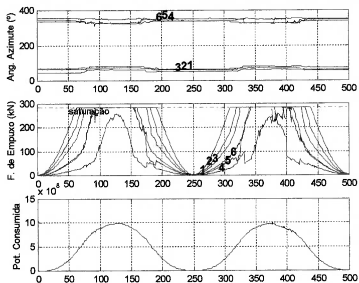
Figura 4.8 – Ângulos de azimute, forças comandadas e potência consumida para a aplicação senoidal.
