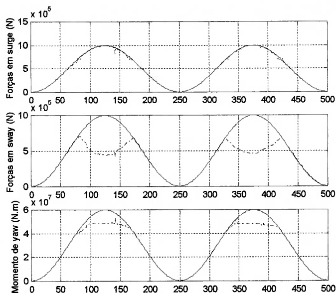
Figura 4.9 – Diferenças de forças comandadas e produzidas considerando a força senoidal.
