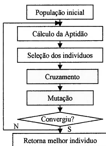
Figura 3.12 – Fluxograma representativo das etapas do SGA.
