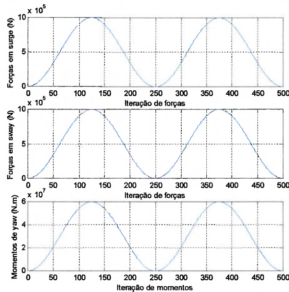
Figura 4.3 – Representação da variação de forças comandadas senoidalmente, em um único sentido.
