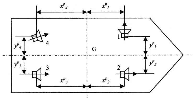
Figura 3.4 – Distribuição dos propulsores no casco da embarcação
