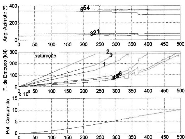
Figura 4.6 – Ângulos de azimute, forças comandadas e potência consumida para uma variação linear de forças usando algoritmos genéticos binários.
