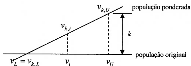
Figura 3.16 – Aplicação dos fatores de ponderação ao Grupo 1.
