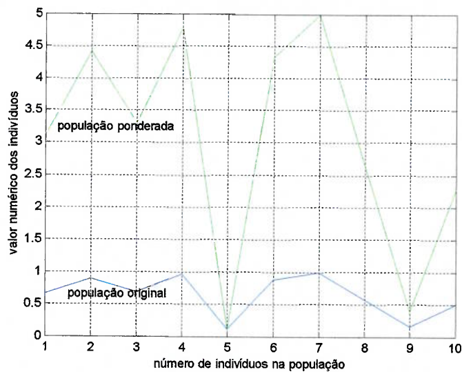
Figura 3.17 – Aplicação do fator de ponderação k = 5 a uma população com 10 indivíduos normalizada.
