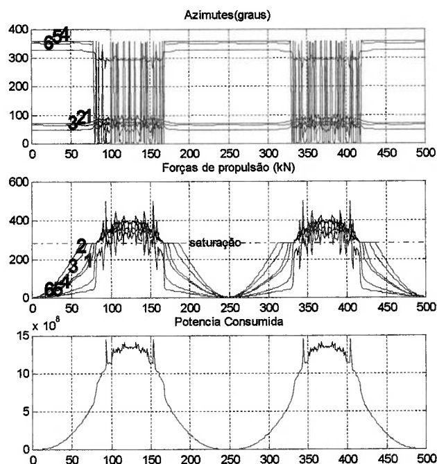
Figura 4.16– Ângulos de azimute, forças de empuxo e potência consumida par a forma senoidal do método SQP.
