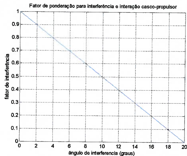
Figura 3.18 – Fator de ponderação k_{prop} proporcional ao ângulo de interferência e de incidência sobre o casco, respectivamente.
