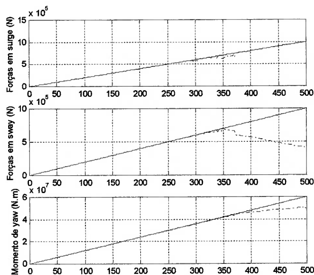
Figura 4.7 – Forças comandadas e produzidas, para a forma linear com algoritmos genéticos binários.
