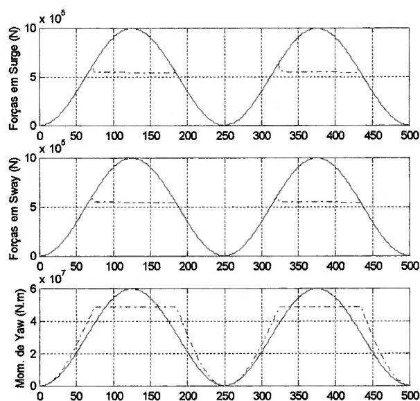
Figura 4.13 – Forças comandadas e produzidas, para a forma senoidal com algoritmos genéticos reais.
