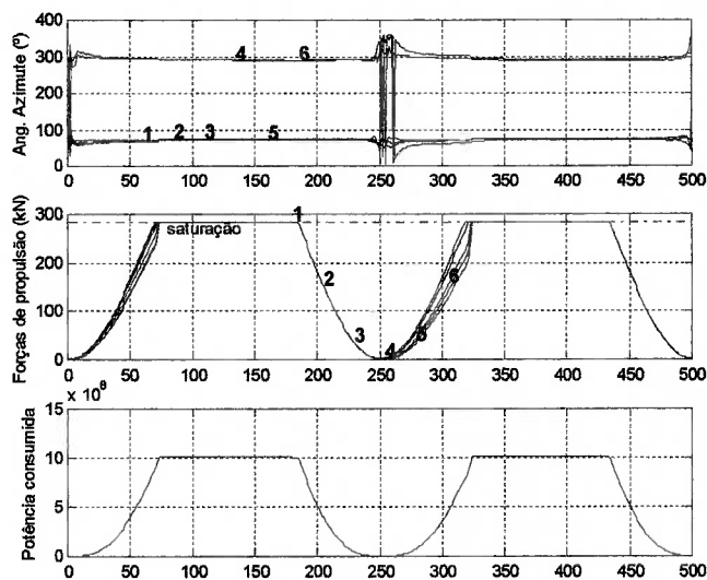
Figura 4.12 – Ângulos de azimute, forças comandadas e potência consumida para uma variação senoidal de forças usando algoritmos genéticos reais.
