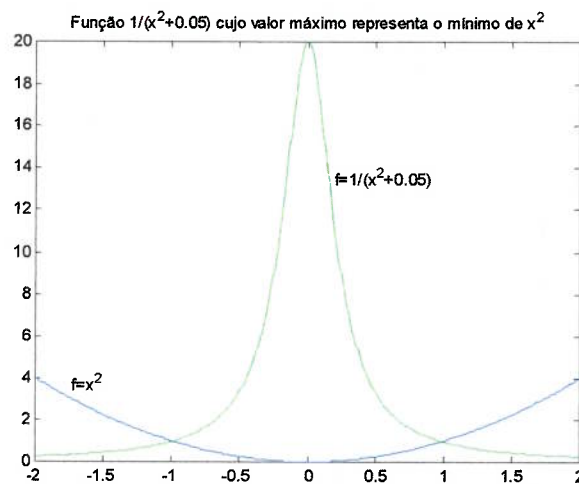
Figura 3.13 – Representação de uma função quadrática normal e transformada. A função transformada permite a determinação do valor mínimo da função original através do seu valor máximo.
