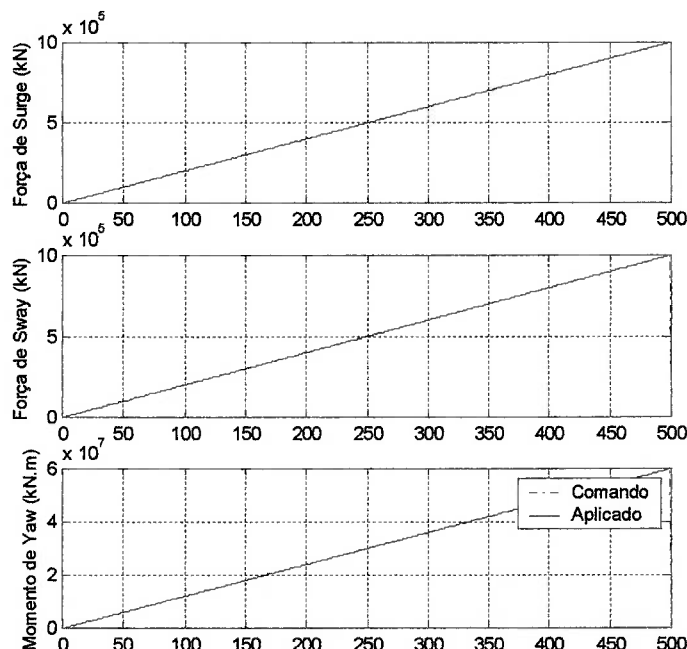
Figura 4.15– Forças comandadas e produzidas, para a forma linear usando SQP.
