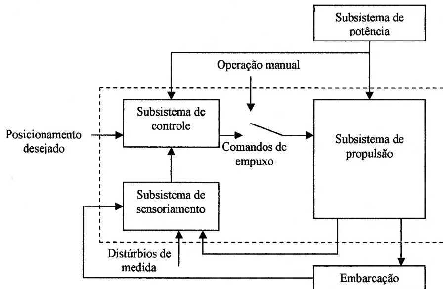
Figura 1.4 – Estrutura Básica do controle da embarcação (extraído em partes de HAMAMATSU, 2002; TANNURI, 2002 e DONHA, 1989).
