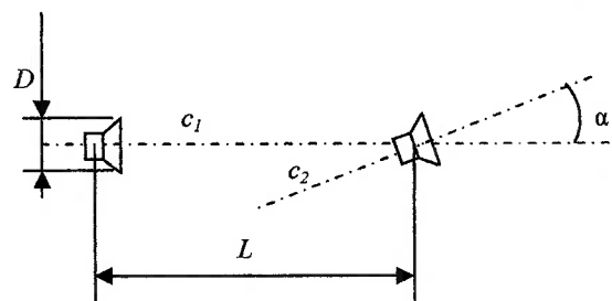
Figura 3.6– Interferência entre dois propulsores. O ângulo \alpha é o ângulo de interferência entre eles, obtido pelas linhas de ação c_1 e c_2
