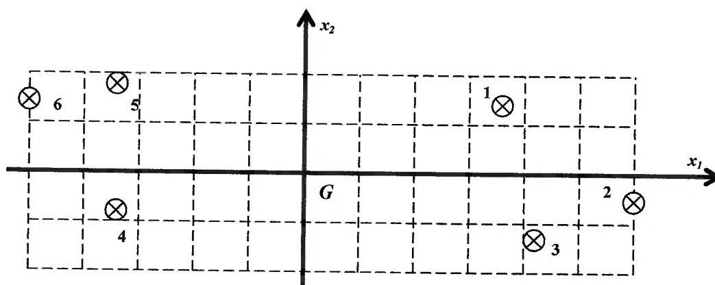
Figura 4.1 – Disposição dos propulsores no casco da barçaça BGL1 (extraída e adaptada de TANNURI, 2002).
