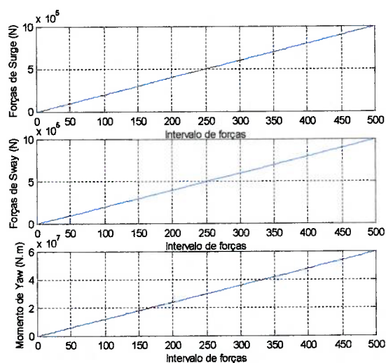
Figura 4.2 – Representação da variação de forças comandadas linearmente.
