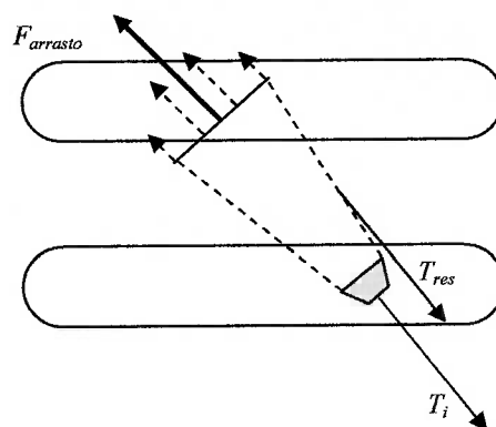
Figura 3.11 – Interação casco-propulsor (extraída e adaptada de SINDING; ANDERSEN, 1998)
