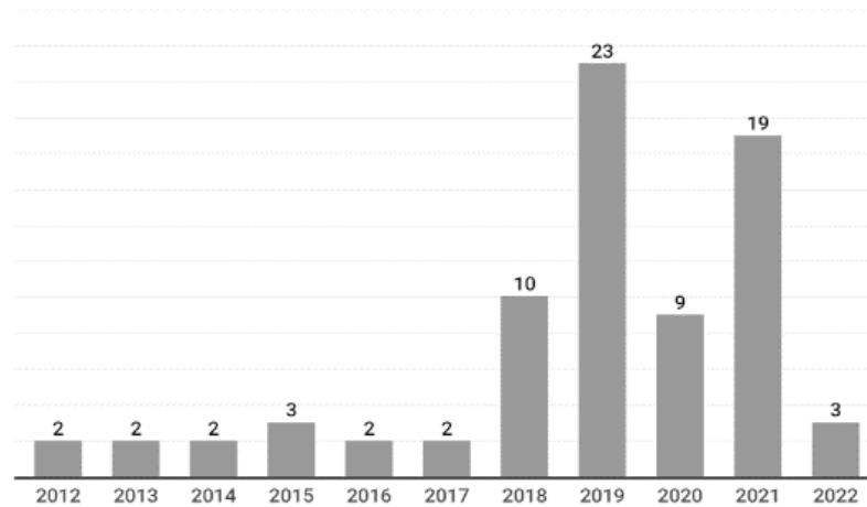
Gráfico 1 - Gráfico com a distribuição das publicações por ano
