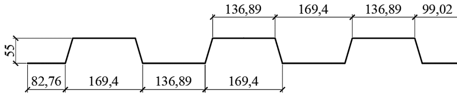
Figura 7.2 – Seção transversal da fôrma de aço linearizada
