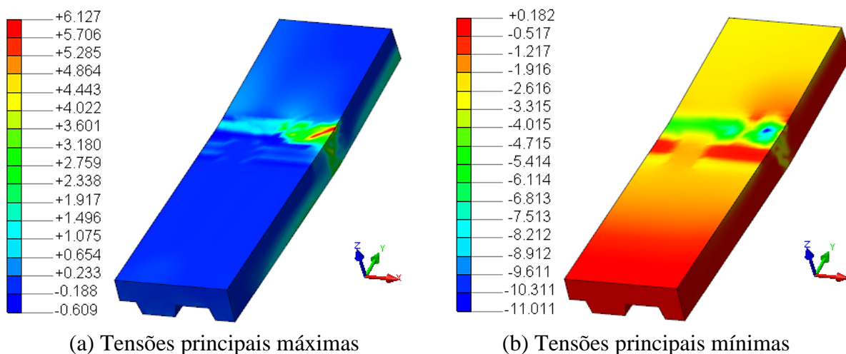
Figura 7.39 – Tensões principais no concreto do modelo numérico inicial da laje mista com os parâmetros de interface do modelo numérico do ensaio slip-block
