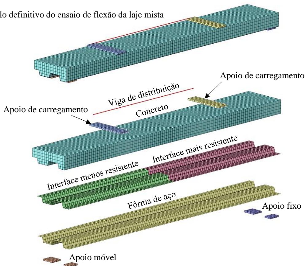
Figura 7.52 – Estrutura do modelo numérico do ensaio de flexão da laje mista
