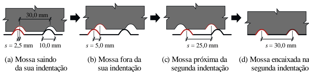
Figura 6.17 – Processo de deslizamento do concreto em relação à moisa da fôrma de aço
