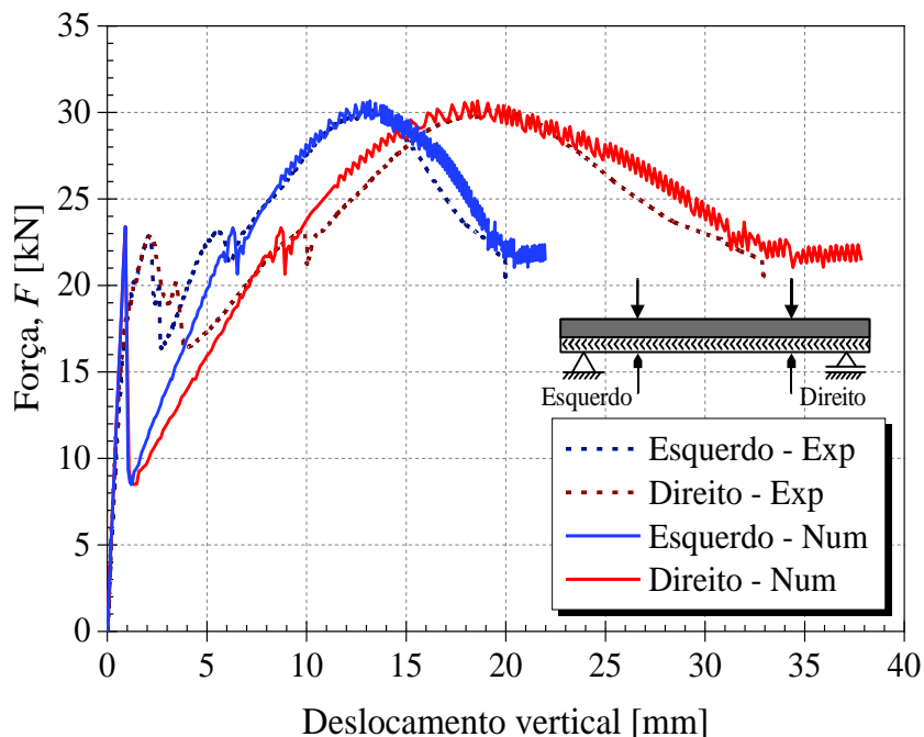
Figura 7.58 – Gráficos da Força versus Deslocamento vertical das seções localizadas abaixo do carregamento aplicado – modelo numérico definitivo – Laje 1
