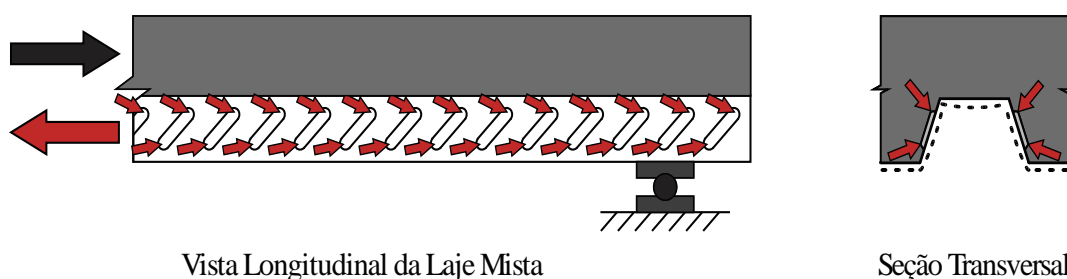
Figura 2.14 – Esquema do mecanismo de resistência ao deslizamento longitudinal
