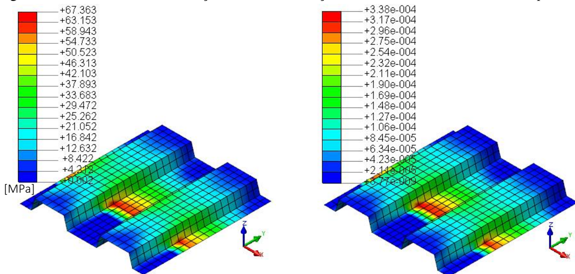
(a) Tensão de Von Mises
