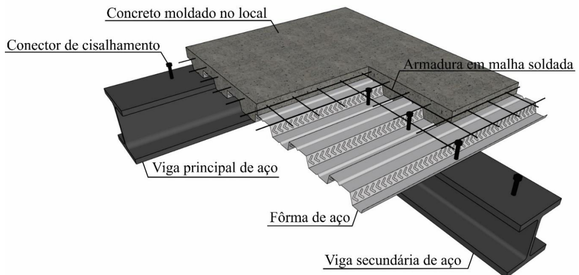
Figura 1.1 – Exemplo da estrutura de um piso misto
