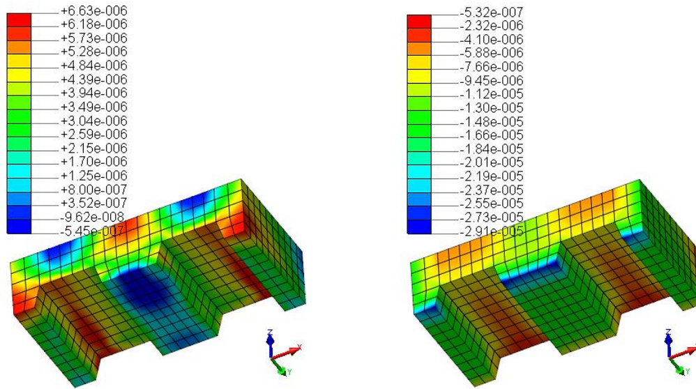
(a) Tensões principais máximas
