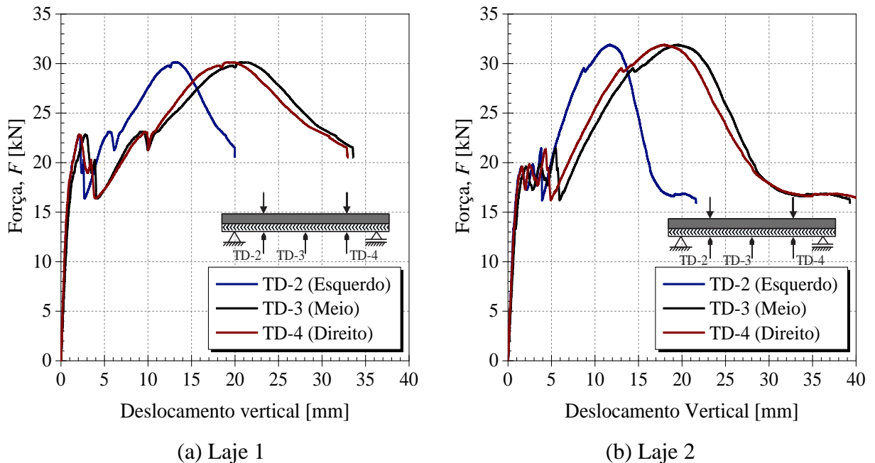
Figura 6.29 – Gráficos da Força versus Deslocamento vertical nos três pontos de medição
