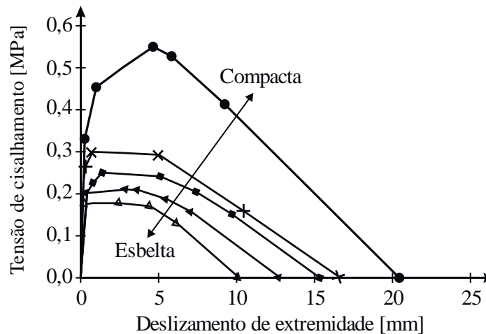
Figura 4.19 – Gráfico da tensão de cisalhamento longitudinal versus deslizamento para os resultados de Abdullah (2004)
