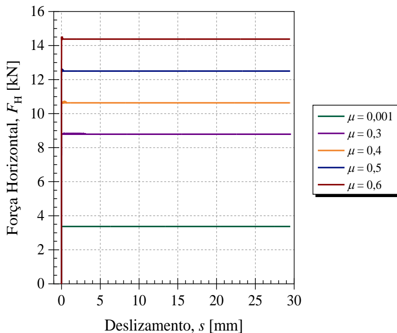
Figura 7.12 – Gráfico de F_H versus s do modelo numérico do ensaio slip-block – análise de \mu
