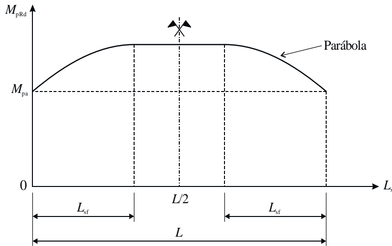
Figura 5.8 – Curva típica M_{Rd} versus L_x para Método da Interação Parcial
