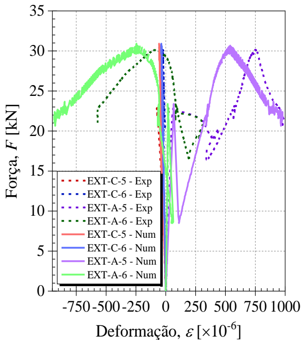
(c) Gráfico da Força versus Deformação específica dos materiais – Seção C-C
