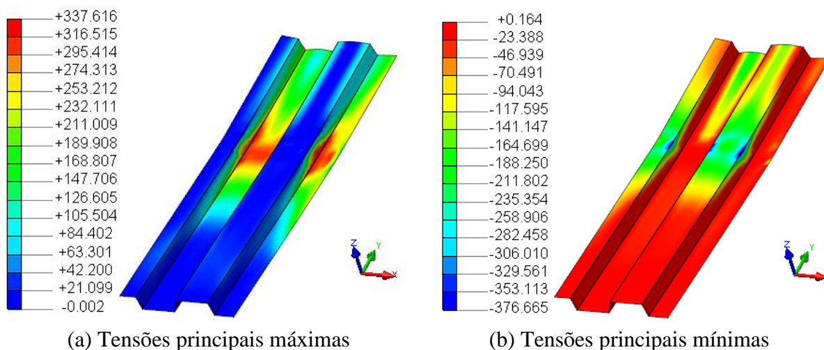
Figura 7.40 – Tensões principais na fôrma de aço do modelo numérico inicial da laje mista com os parâmetros de interface do modelo numérico do ensaio slip-block
