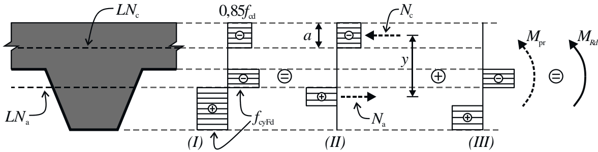
Figura 5.4 – Distribuição de tensões de momento fletor positivo em uma seção qualquer da laje mista empregando o Método da Interação Parcial
