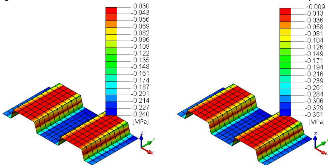
(a) Tensão normal à interface
