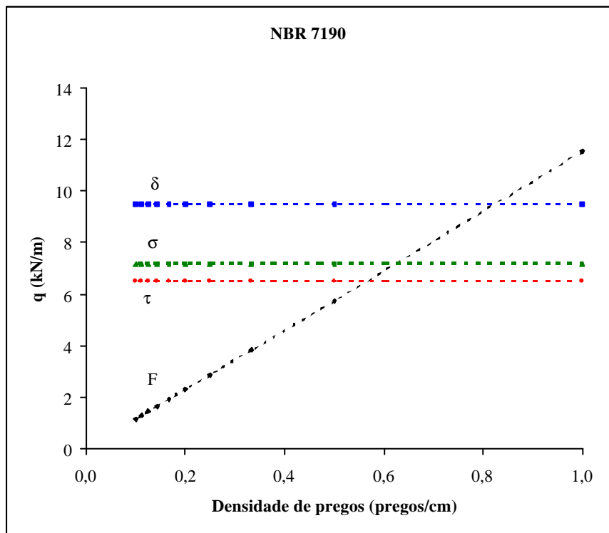
Figura 75 – Valor máximo de carregamento permanente distribuído em função da taxa de conectores – Viga Tipo 1
