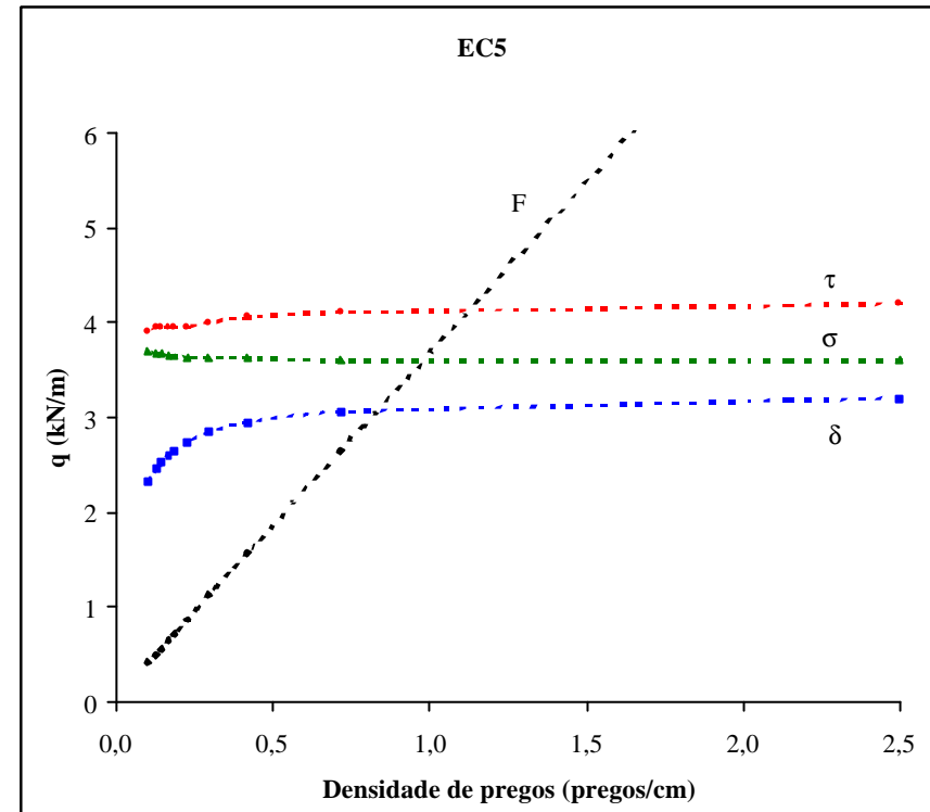
Figura 76 – Valor máximo de carregamento permanente distribuído em função da taxa de conectores – Viga Tipo 2
