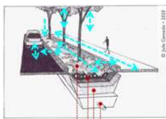
Canal Raso com lados levemente inclinados Terra para Plantio Solo de Bio Retenção Tubulação
