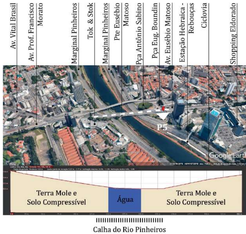
Figura 15: Perfil de Elevação 5: Ponte Eusébio Matoso.
