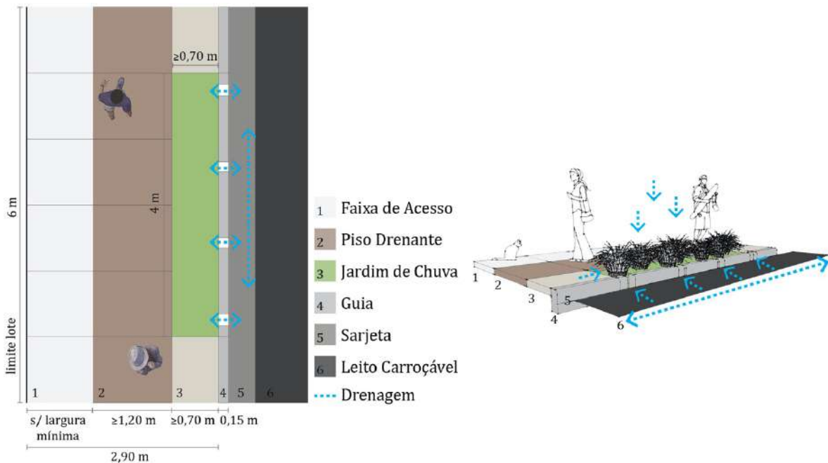
Croqui 19: Jardim de Chuva Organização das Calçadas
