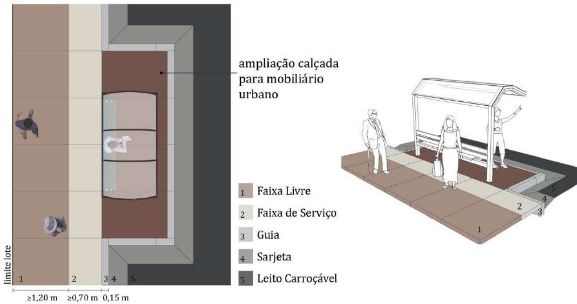
Croqui 17: Ampliação Calçada – Mobiliário Organização das Calçadas Referência: Decreto nº 58611/2019 - Prefeitura do Município de São Paulo (2018) Croqui e Adaptação: Sarah Bezerra Suassuna (2020)
