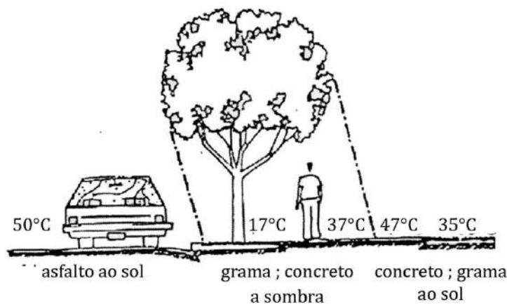
Figura 5: Temperaturas superficiais de diferentes tipos de piso do ambiente urbano.
