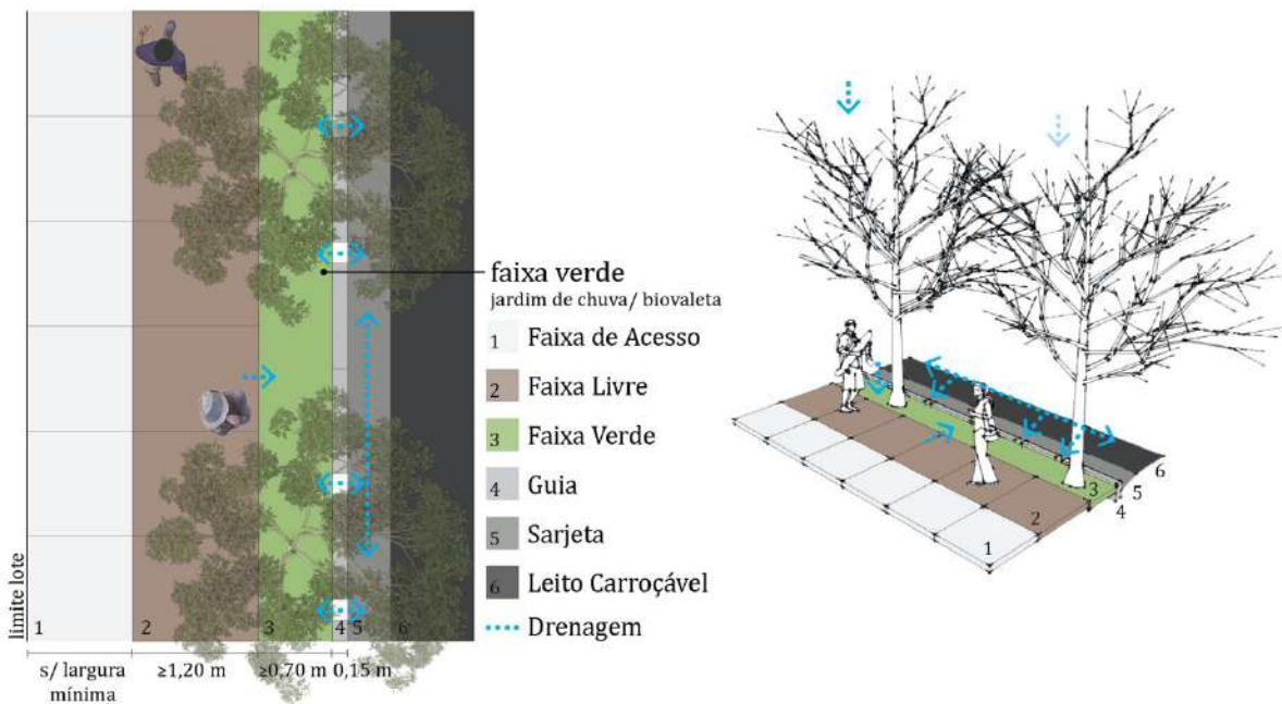
Croqui 18: Calçadas Verdes Organização das Calçadas Referência: Decreto nº 58611/2019 - Prefeitura do Município de São Paulo (2018) Croqui e Adaptação: Sarah Bezerra Suassuna (2020)
