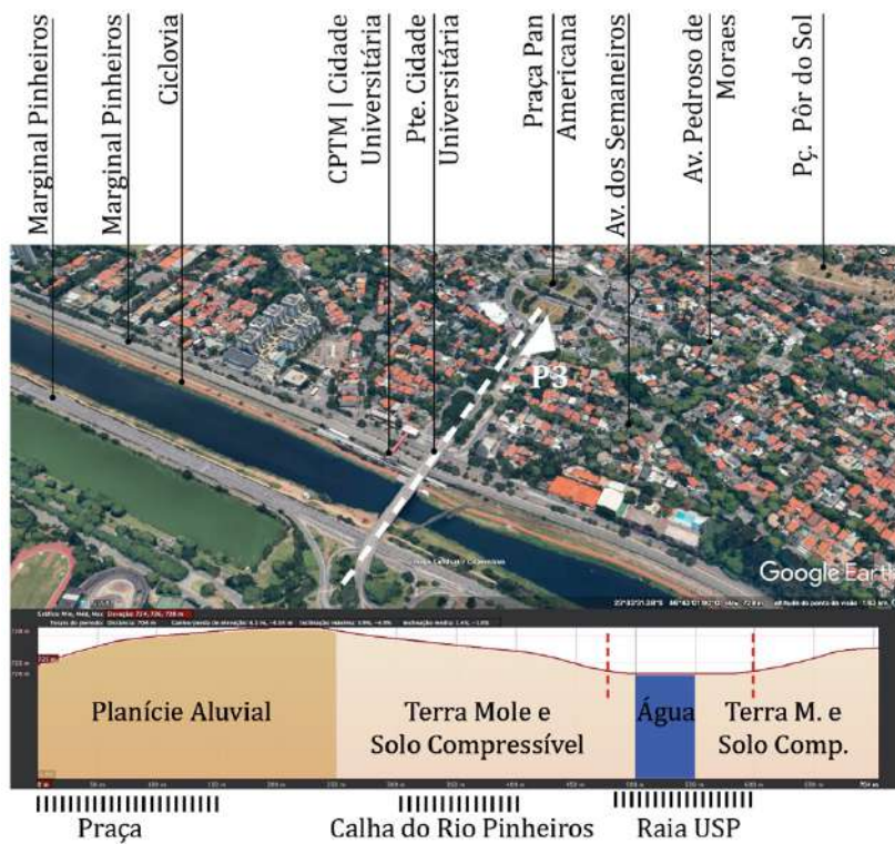
Figura 13: Perfil de Elevação 3: Ponte Cidade Universitária
