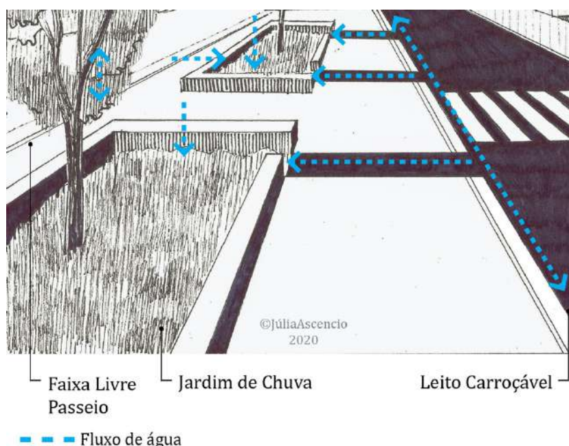
Croqui 1: Jardins de Chuva Tipologias de Elementos de Infraestrutura Verde e Azul Referência: The South Side Green. Infrastructure Charrette Croqui e Adaptação: Júlia Ascencio Cansado (2020)
