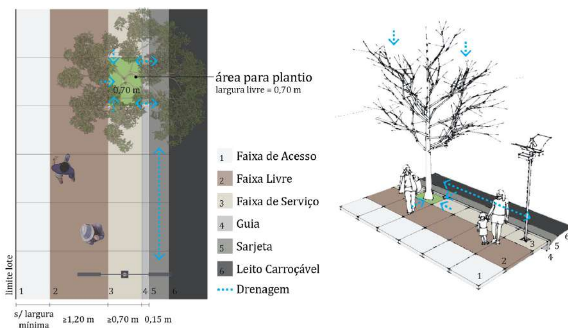
Croqui 16: Faixa de Serviço Organização das Calçadas
