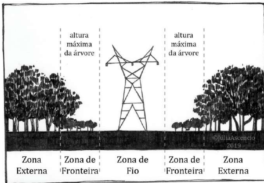
Croqui 11: Corredores Arborizados Amplos Padrão de Distribuição de Árvores em Meio Urbano Referência: Sacramento Municipal Utility District Croqui e Adaptação: Júlia Ascencio Cansado (2019)
