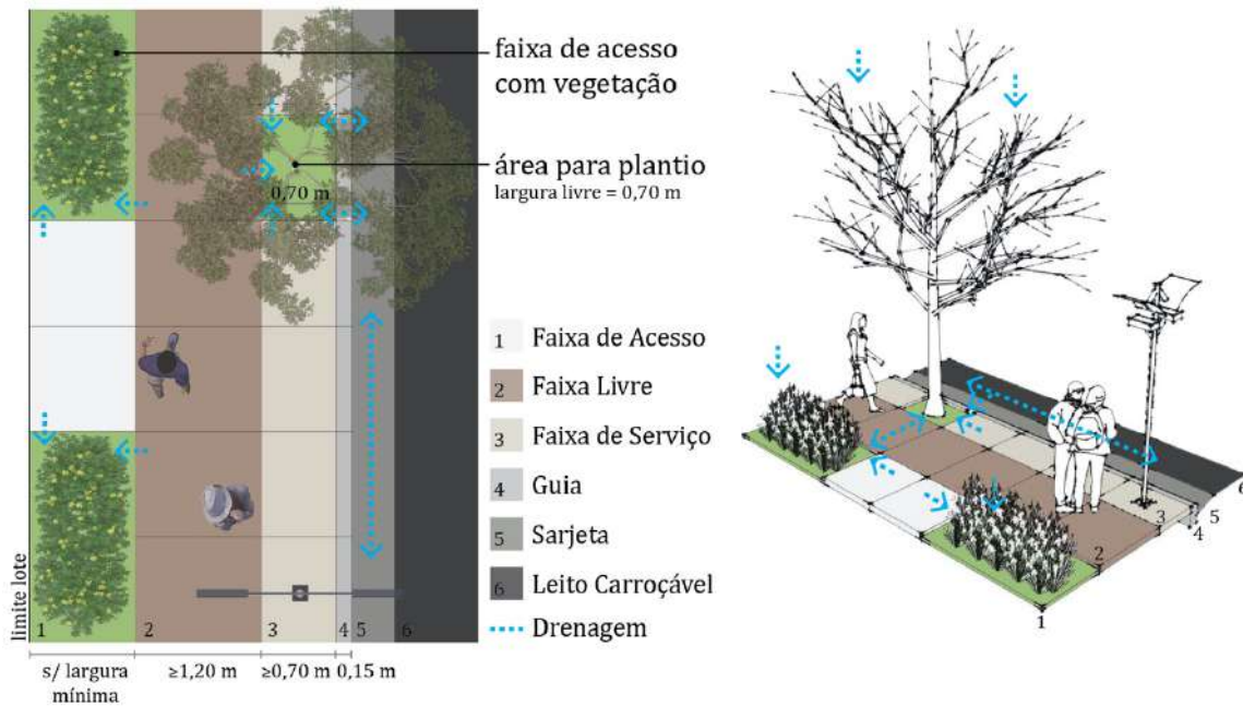
Croqui 15: Faixa de Acesso com Vegetação Organização das Calçadas Referência: nº 58611/2019 - Prefeitura do Município de São Paulo (2018) Croqui e Adaptação: Sarah Bezerra Suassuna (2020)
