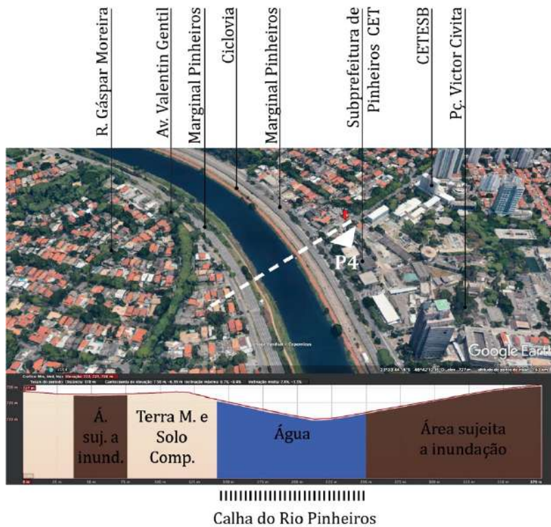
Figura 14: Perfil de Elevação 4: CET – Pinheiros
