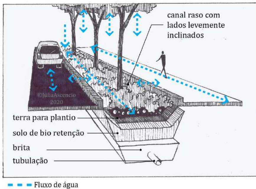
Croqui 2: Biovaletas Tipologias de Elementos de Infraestrutura Verde e Azul Referência: (BRANKOVIC, 2019) Croqui e Adaptação: Júlia Ascencio Cansado (2020)
