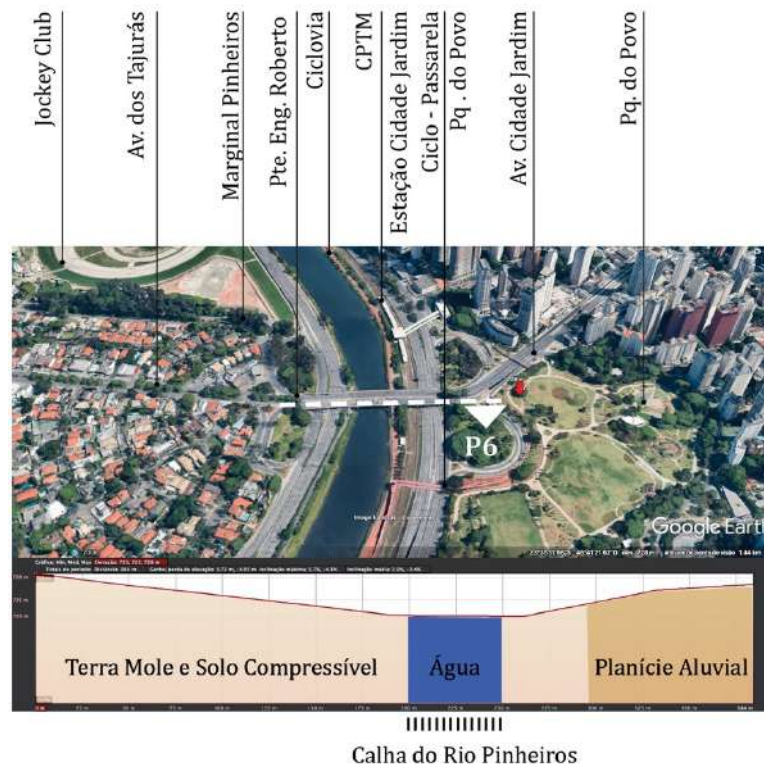
Figura 16: Perfil de Elevação 6: Ponte Engenheiro Roberto Rossi Zuccolo.
