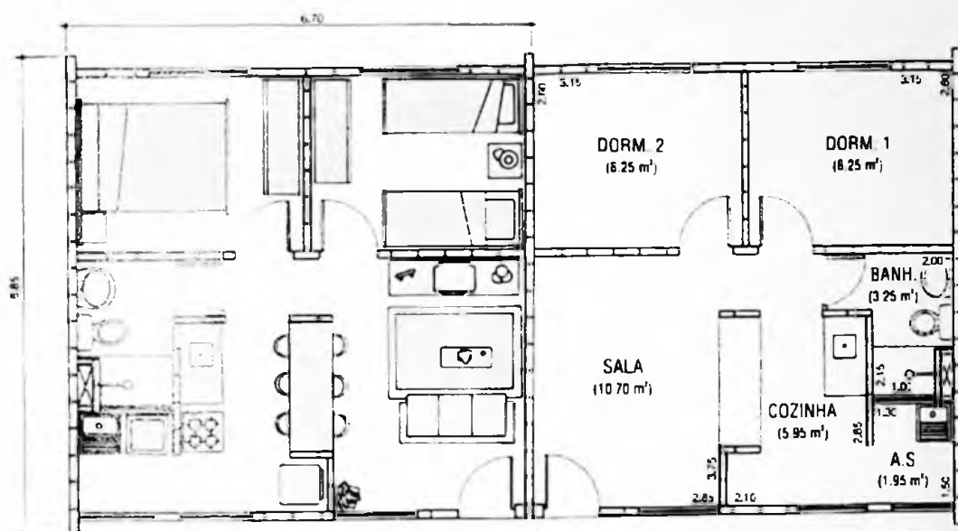
PLANTA TIPO
