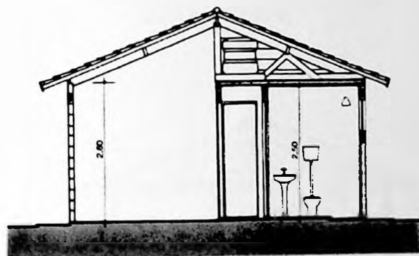
CORTE
