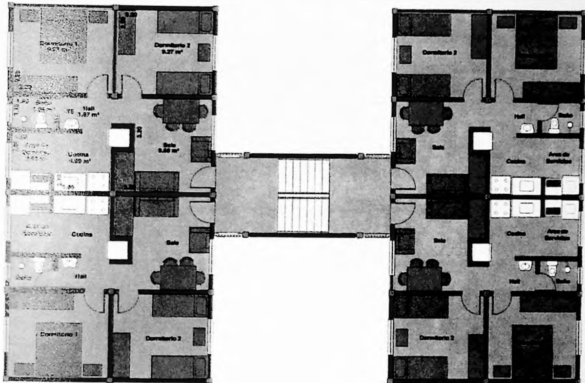
Planta típica
