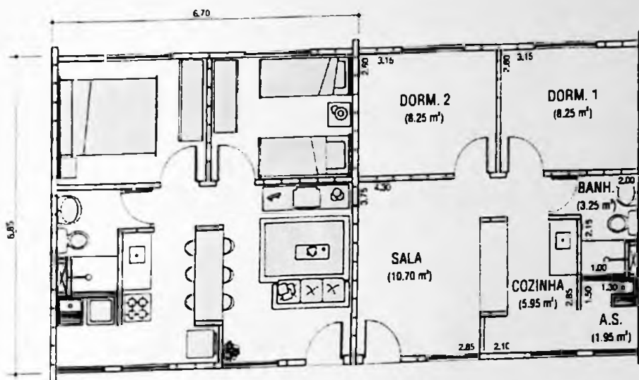
PLANTA TIPO
