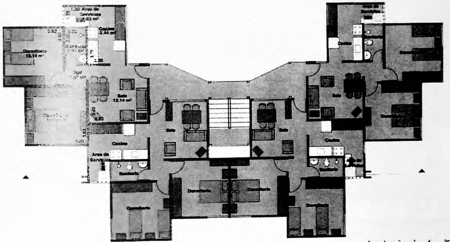
Planta tipo
