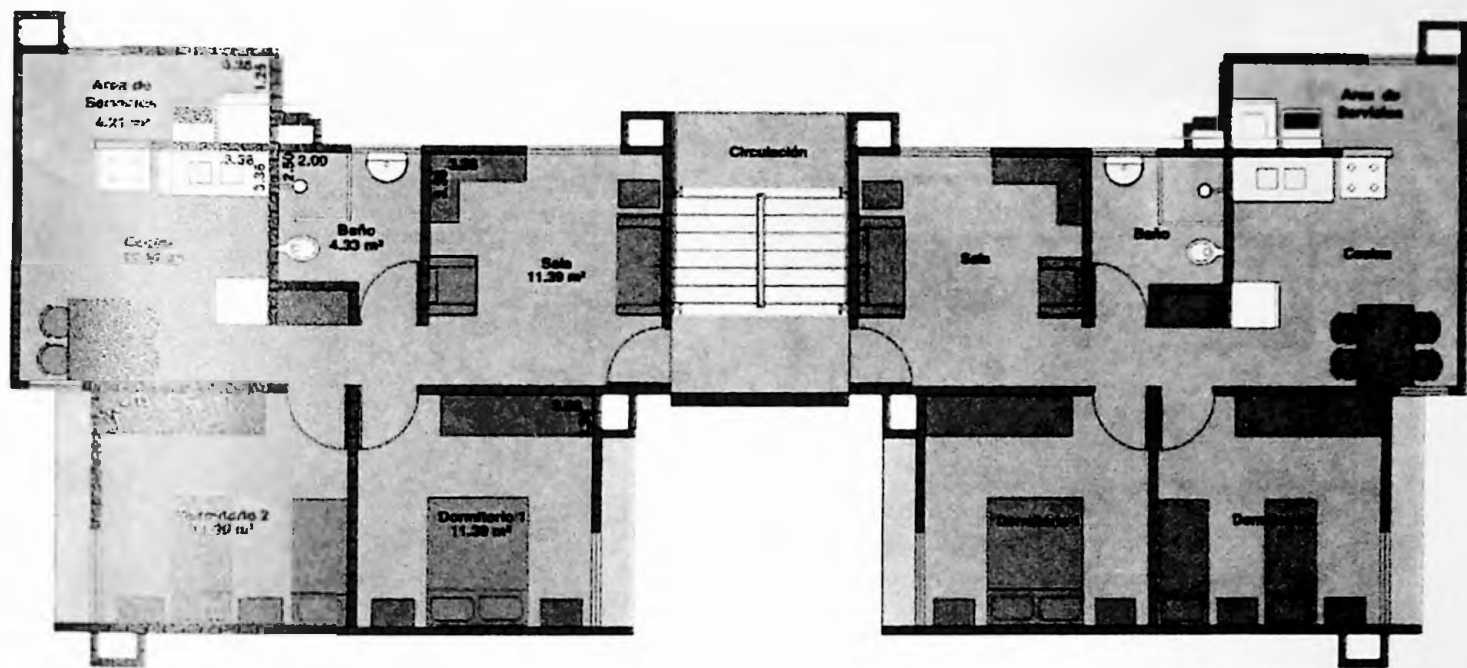
Planta tipo
