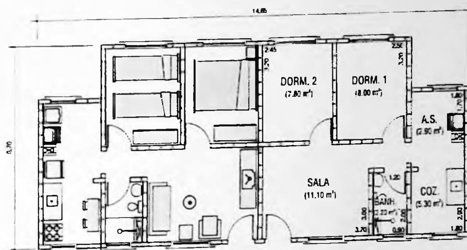
PLANTA TIPO
