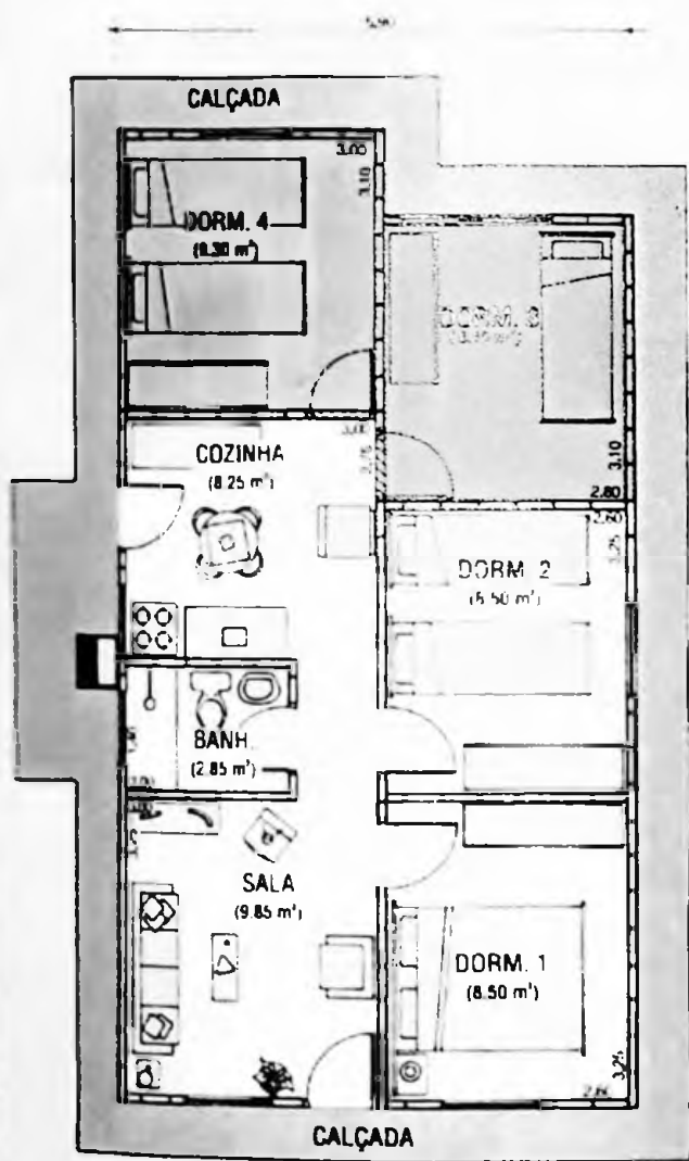
PLANTA
