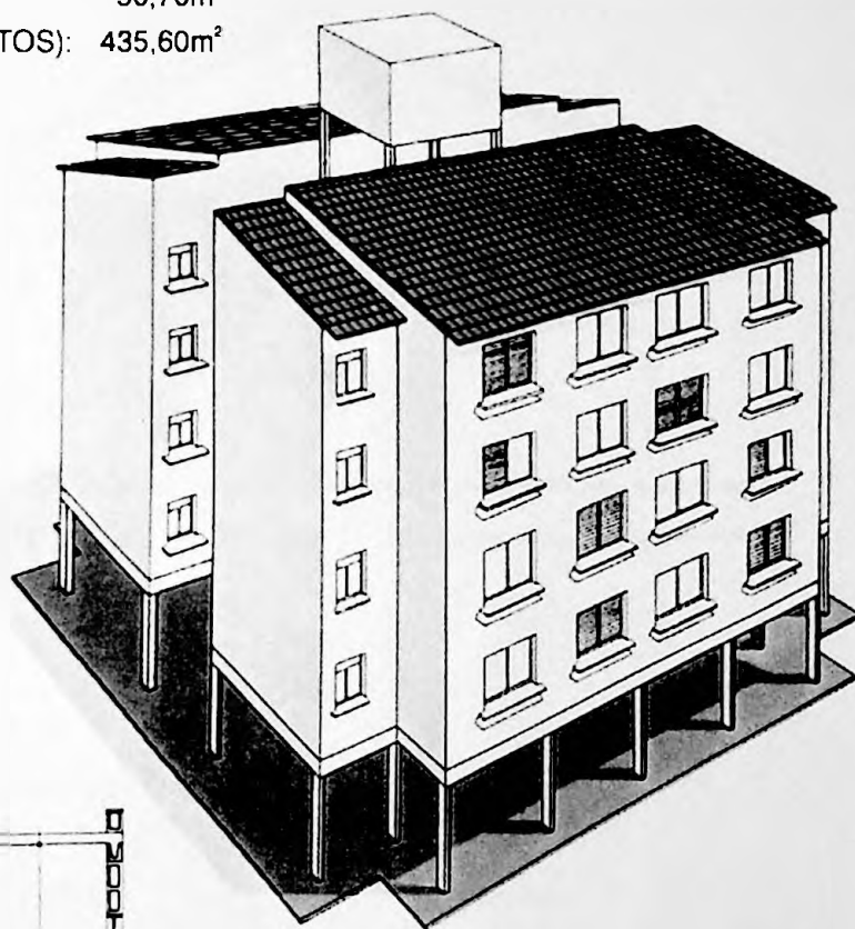
ELEVAÇÃO EM PERSPECTIVA
