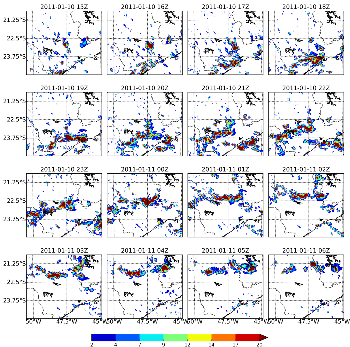
Figura 3.29: Precipitação acumulada em uma hora, em mm, para a simulação NG8UV a partir de 1500 UTC do dia 10/01/2011 até 0600 UTC do dia 11/01/2011.
