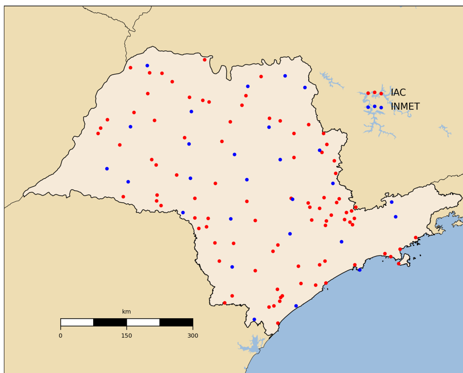
Figura 2.1: Distribuição espacial das estações de superfície utilizadas na análise de Cressman. Em vermelho são indicadas as estações pertencentes ao Instituto Agrônomo de Campinas (IAC) e em azul as estações automáticas pertencentes ao Instituto Nacional de Meteorologia (INMET).
