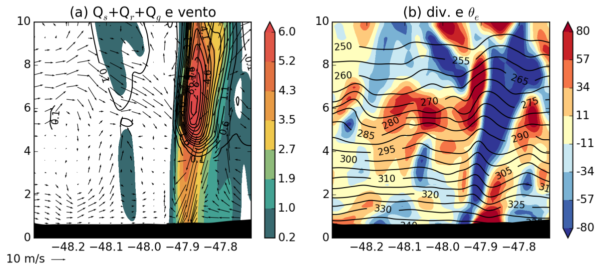
Figura 3.41: Corte vertical DD' entre 23,21^\circ\text{S}/48,29^\circ\text{W} e 23,83^\circ\text{S}/47,72^\circ\text{W} às 1920 UTC do dia 10/01/2011. O eixo x se refere a longitude em graus, enquanto que o eixo y é a altura em km (a) Conteúdo total de hidrometeoros precipitantes ( Q ), dado pela soma da razão de mistura em \text{g kg}^{-1} de neve ( Q_s ), chuva ( Q_r ) e graupel ( Q_g ) (sombreado), razão de mistura das espécies de gelo (contornos) e vento paralelo ao corte vertical (vetores); (b) Divergência horizontal de massa ( 10^{-5} \text{ s}^{-1} ) e temperatura potencial equivalente ( \theta_e ) em K.
