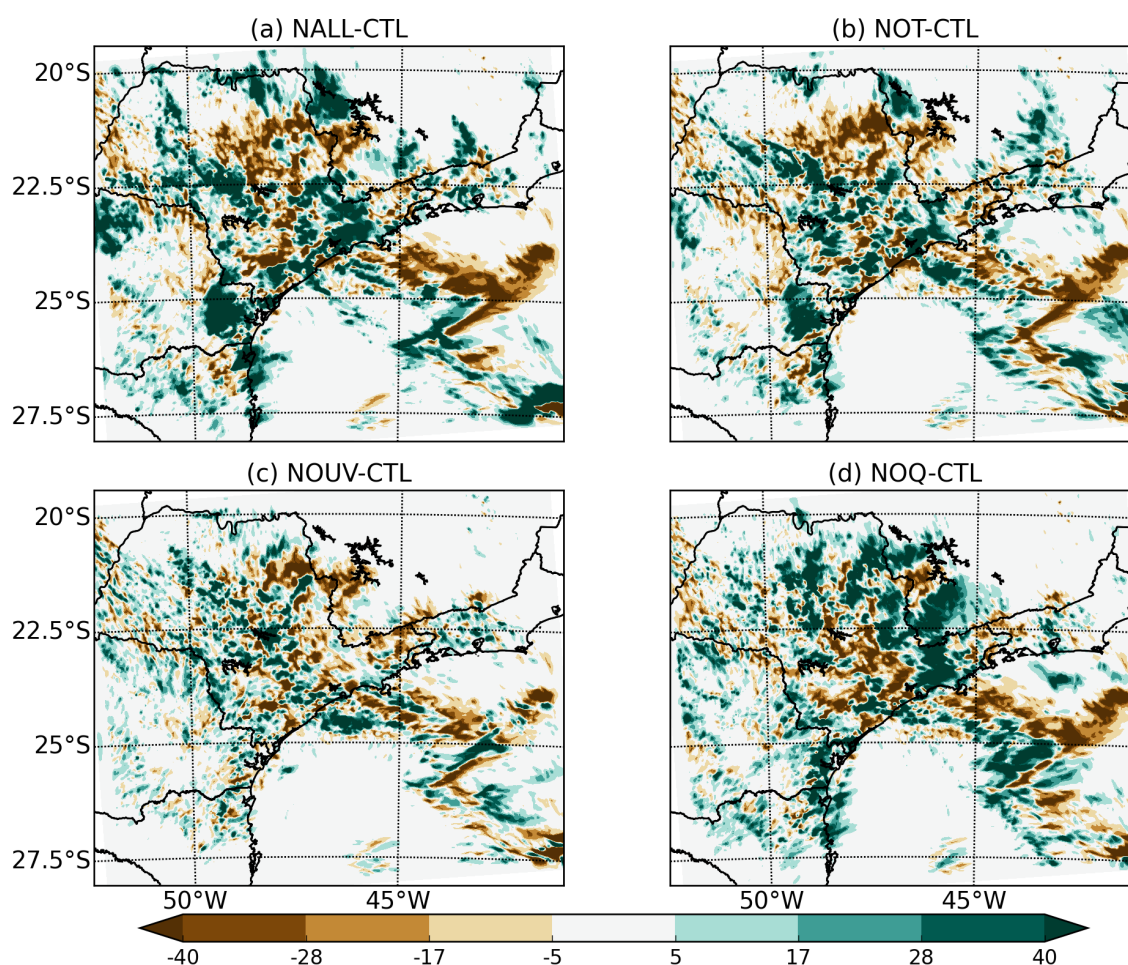
Figura 3.20: Diferença entre os experimentos com assimilação de dados e a simulação controle para a precipitação acumulada entre às 1800 UTC do dia 10 e às 0600 UTC do dia 11 de janeiro de 2011 para: (a) NALL-CTL; (b) NOT-CTL; (c) NOUV-CTL; (d) NOQ-CTL.
