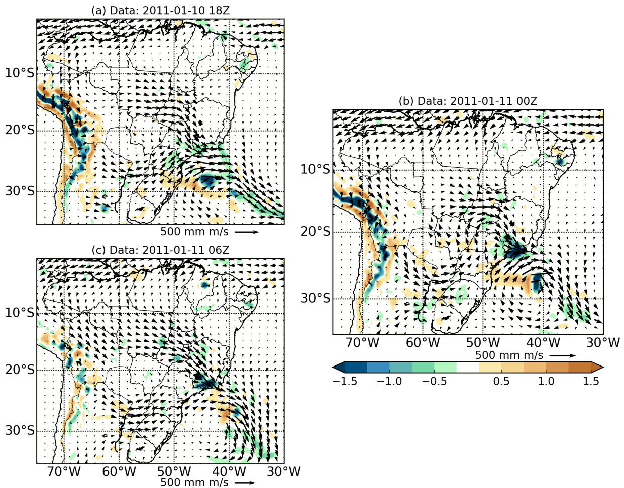
Figura 3.3: Transporte de umidade integrado verticalmente entre 850 hPa e 500 hPa ( \vec{Q} ) (vetores) e divergente de \vec{Q} ( \nabla \cdot \vec{Q} ) ( 10^{-3} \text{ mm s}^{-1} ) (sombreado) calculado com a análise do GFS de 0,5^\circ , para (a): Dia 10/01/2011 às 1800 UTC; (b) Dia 11/01/2011 à 0000 UTC; (c) Dia 11/01/2011 às 0600 UTC.
