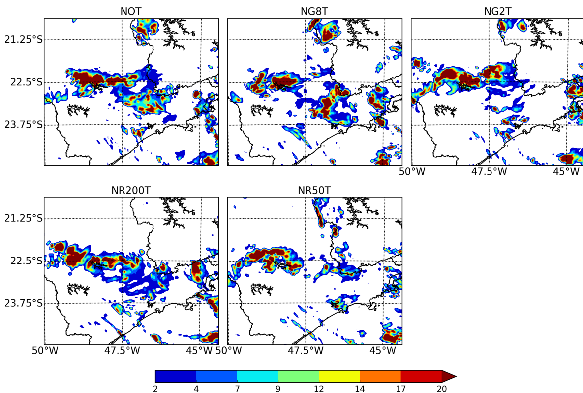
Figura 3.30: Precipitação acumulada entre 2300 UTC do dia 10/01/2011 e 0000 UTC do dia 11/01/2011, em mm, para as simulações NOT, NG8T, NG2T, NR200T e NR50T.
