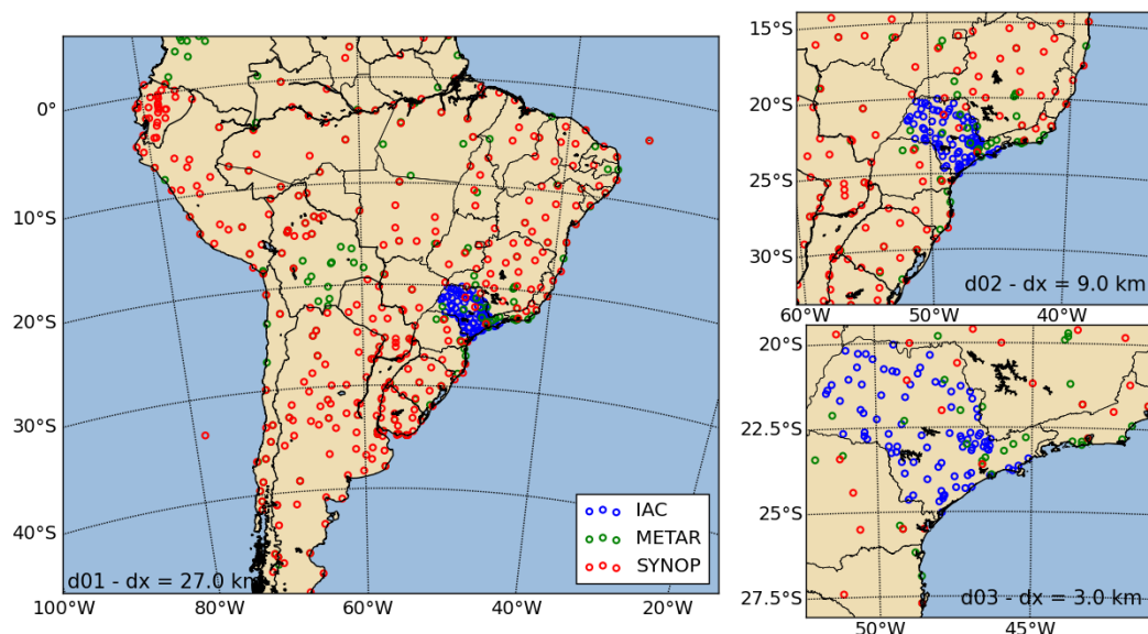
Figura 2.3: Distribuição espacial das observações de superfície assimiladas nos experimentos em cada um dos três domínios utilizados (d01, d02, d03).
