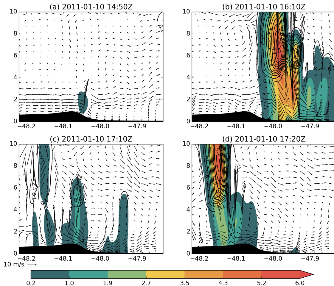
Figura 3.39: Corte vertical CC' entre 23,89^{\circ}\text{S}/48,22^{\circ}\text{W} e 24,56^{\circ}\text{S}/47,83^{\circ}\text{W} com o conteúdo total de hidrometeoros precipitantes ( Q ), dado pela soma da razão de mistura em \text{g kg}^{-1} de neve ( Q_s ), chuva ( Q_r ) e graupel ( Q_g ) (sombreado), razão de mistura das espécies de gelo (contornos) e vento paralelo ao corte vertical (vetores). O eixo x se refere a longitude em graus, enquanto que o eixo y é a altura em km às (a) 1450 UTC do dia 10/01/2011; (b) 1610 UTC do dia 10/01/2011; (c) 1710 UTC do dia 10/01/2011; (d) 1720 UTC do dia 10/01/2011.
