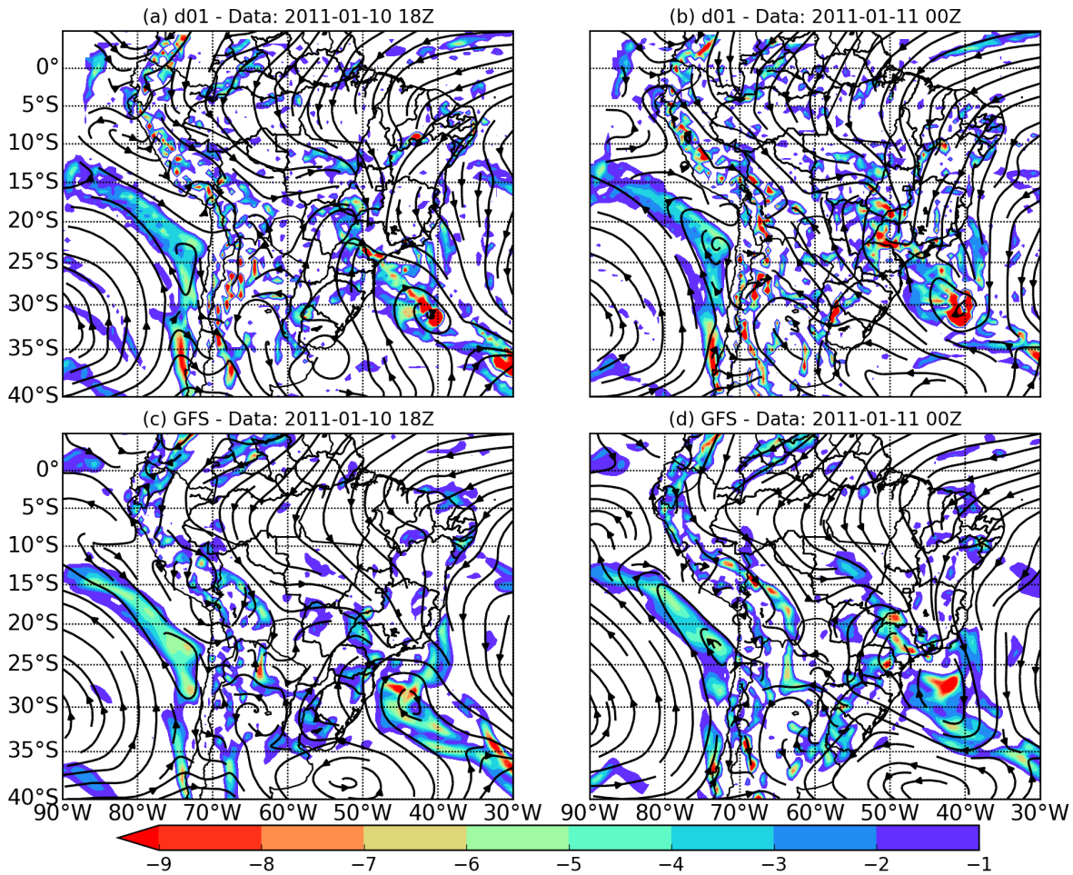
Figura 3.10: Linhas de corrente em 850 hPa e vorticidade relativa ( 10^{-5} \text{ s}^{-1} ), obtidos com os dados da simulação controle para o domínio d01 para o dia 10/01/2011 às 1800 UTC (a) e dia 11/01/2011 à 0000 UTC (b). As figuras (c) e (d) são similares a (a) e (b), porém para a análise do GFS de 0,5°.
