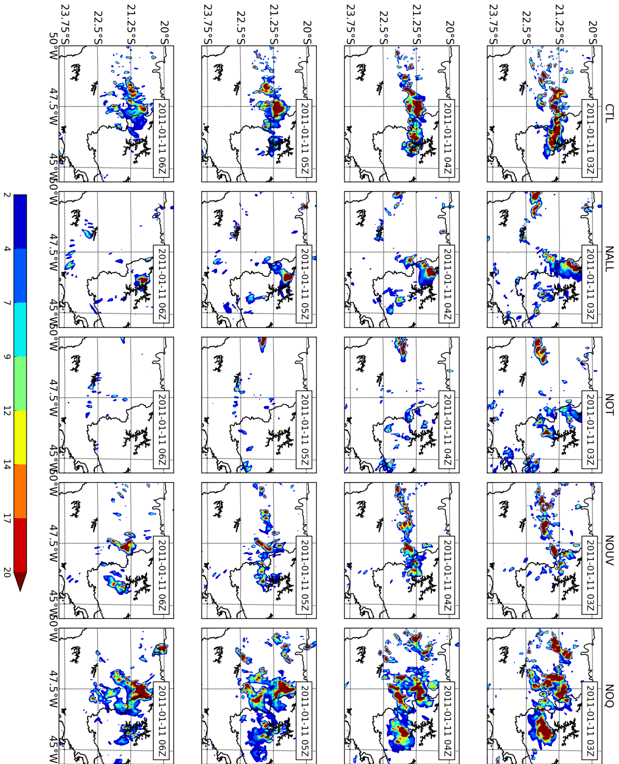
Figura 3.26: Precipitação acumulada em uma hora, em mm, para a simulação CTL, NALL, NOT, NOUV e NOQ entre 0300 e 0600 UTC do dia 11/01/2011.
