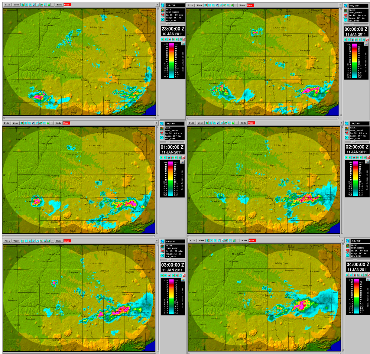
Figura 3.15: Precipitação acumulada em uma hora, em mm, pelas estimativas dos radares de Bauru e Presidente Prudente entre 2300 UTC do dia 10/01/2011 e 0400 UTC do dia 11/01/2011.
