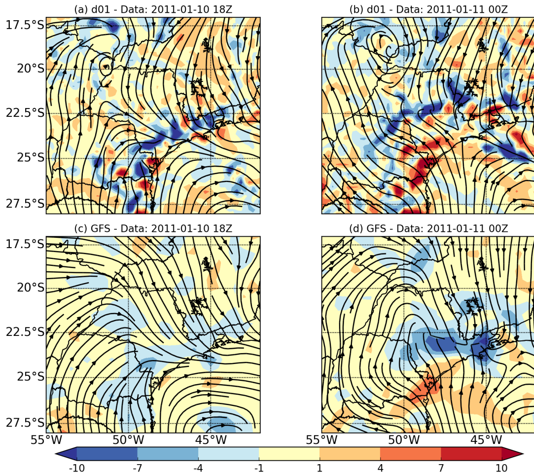
Figura 3.11: Linhas de corrente em 850 hPa e divergência de massa ( 10^{-5} \text{ s}^{-1} ), obtidos com os dados da simulação controle para o domínio d01 para o dia 10/01/2011 às 1800 UTC (a) e dia 11/01/2011 à 0000 UTC (b). As figuras (c) e (d) são similares a (a) e (b), porém para a análise do GFS de 0,5^\circ .
