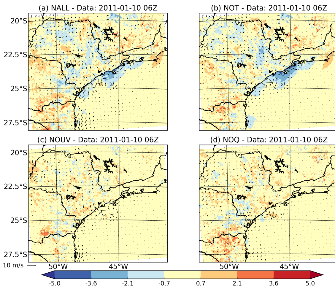
Figura 3.18: Diferença média no domínio d03 entre a temperatura a 2 metros (sombreado) e o vento a 10 metros da superfície (vetores) às 0600 UTC do dia 10/01/2015 para: (a) NALL-CTL; (b) NOT-CTL; (c) NOUV-CTL; (d) NOQ-CTL.
