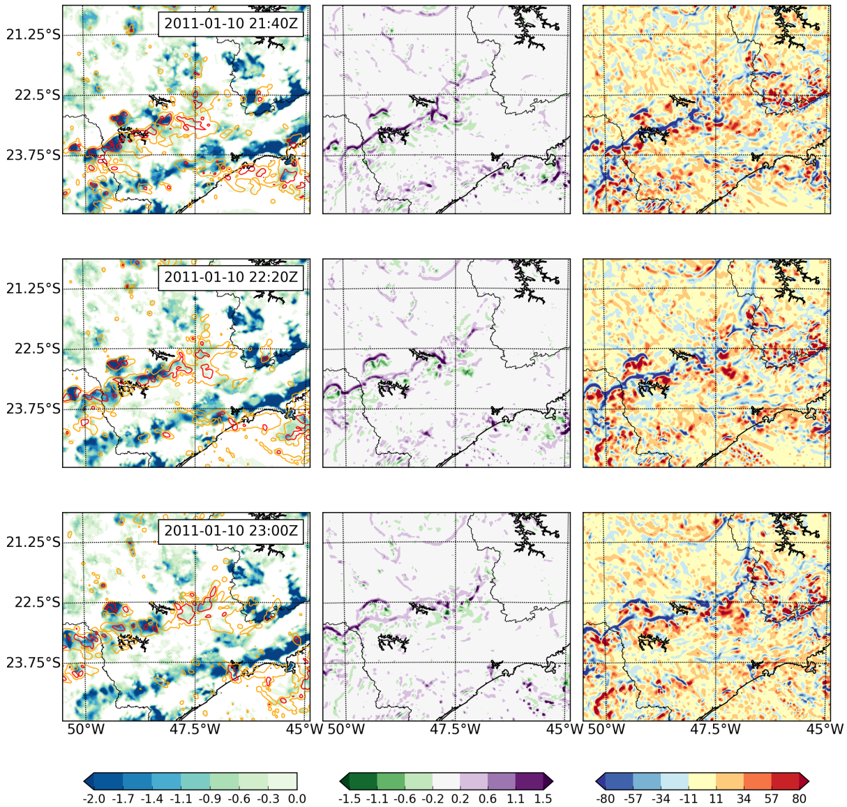
Figura 3.44: A coluna da esquerda representa a anomalia da temperatura em ^{\circ}\text{C} a 2 metros (sombreado) ( T'_{2m} ) e taxa de precipitação em \text{mm hora}^{-1} que excede 1 e 20 \text{ mm hora}^{-1} em contornos laranja e vermelho, respectivamente; a coluna do meio apresenta a velocidade vertical a 1,2 km de altura em \text{m s}^{-1} ; a coluna da direita indica a divergência calculada a 1,2 km de altura ( 10^{-5} \text{ s}^{-1} ). Esses campos são representados para o dia 10/01/2011 às 2140 UTC, 2220 UTC e 2300 UTC.
