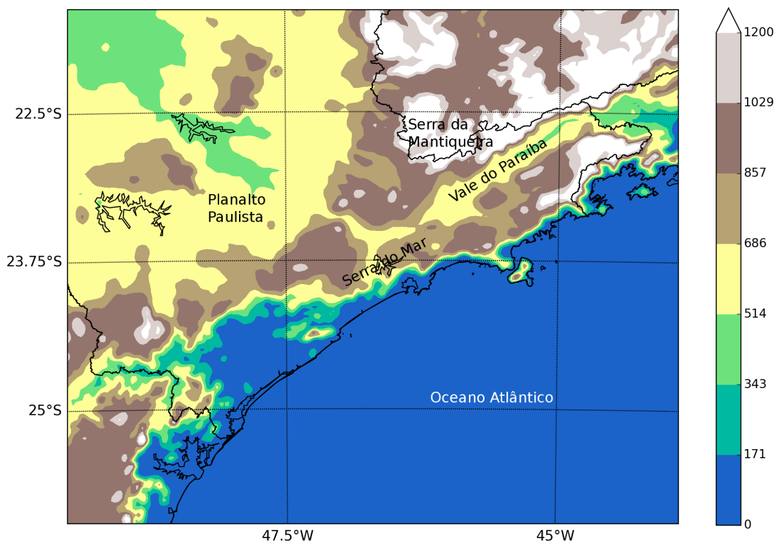
Figura 1.4: Altura topográfica em metros, com destaque para as principais regiões.
