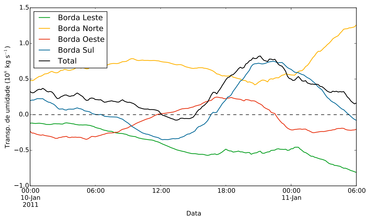
Figura 3.34: Transporte de umidade integrado verticalmente entre 850 e 500 hPa calculado com a simulação NG8UV através das bordas Oeste, Norte, Leste e Sul do subdomínio delimitado pelas coordenadas 25^{\circ}\text{S}/50^{\circ}\text{W} e 21^{\circ}\text{S}/44^{\circ}\text{W} ( 10^8 \text{ kg s}^{-1} ). Valores positivos indicam que há umidade entrando no subdomínio e valores negativos que há umidade saindo do subdomínio.
