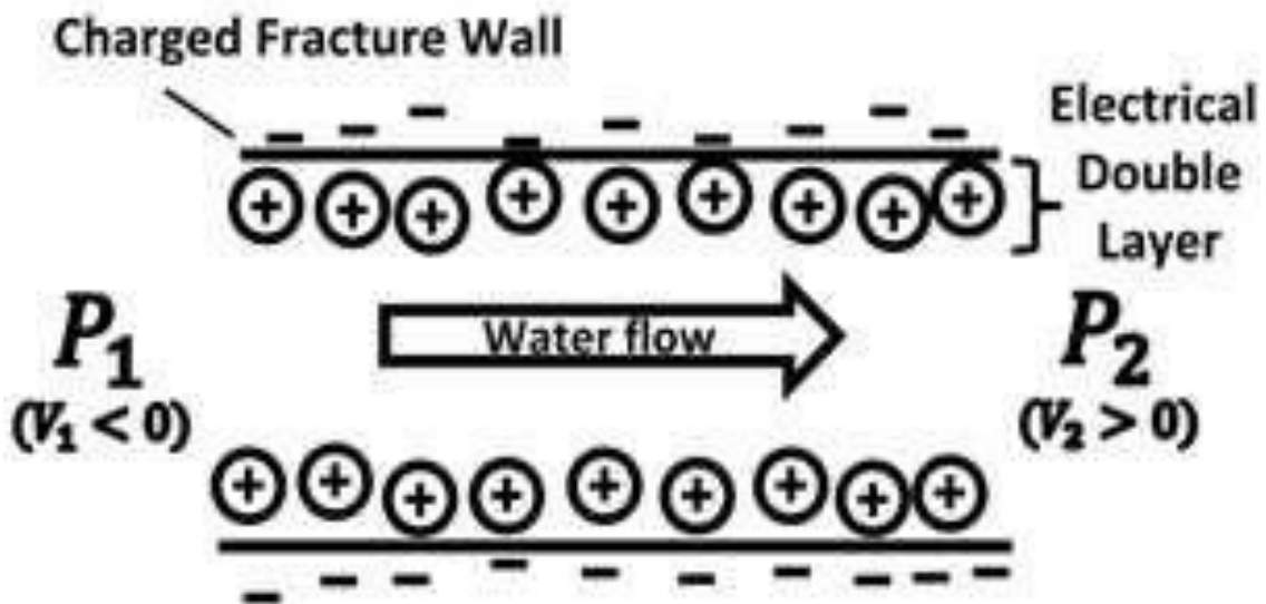
Figura 3.4 – Esquema simplificado para um modelo de fratura com a presença da dupla camada elétrica formada próxima à interface entre as paredes da fratura na presença de um eletrólito. Nessa situação, um fluxo se estabelece da esquerda para a direita correspondendo a um gradiente de pressão P_1 > P_2 nas extremidades da fratura (adaptado de Kowalski et al., 2020).
