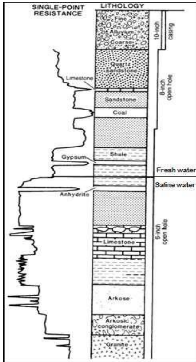
Figura 2.4 – Perfil esquemático com diversas unidades litológicas e variações do diâmetro do poço, assim como a curva representando a resposta relativa de acordo com essas mudanças ao utilizar a perfilagem SPR (Adaptado de Keys, 1990).
