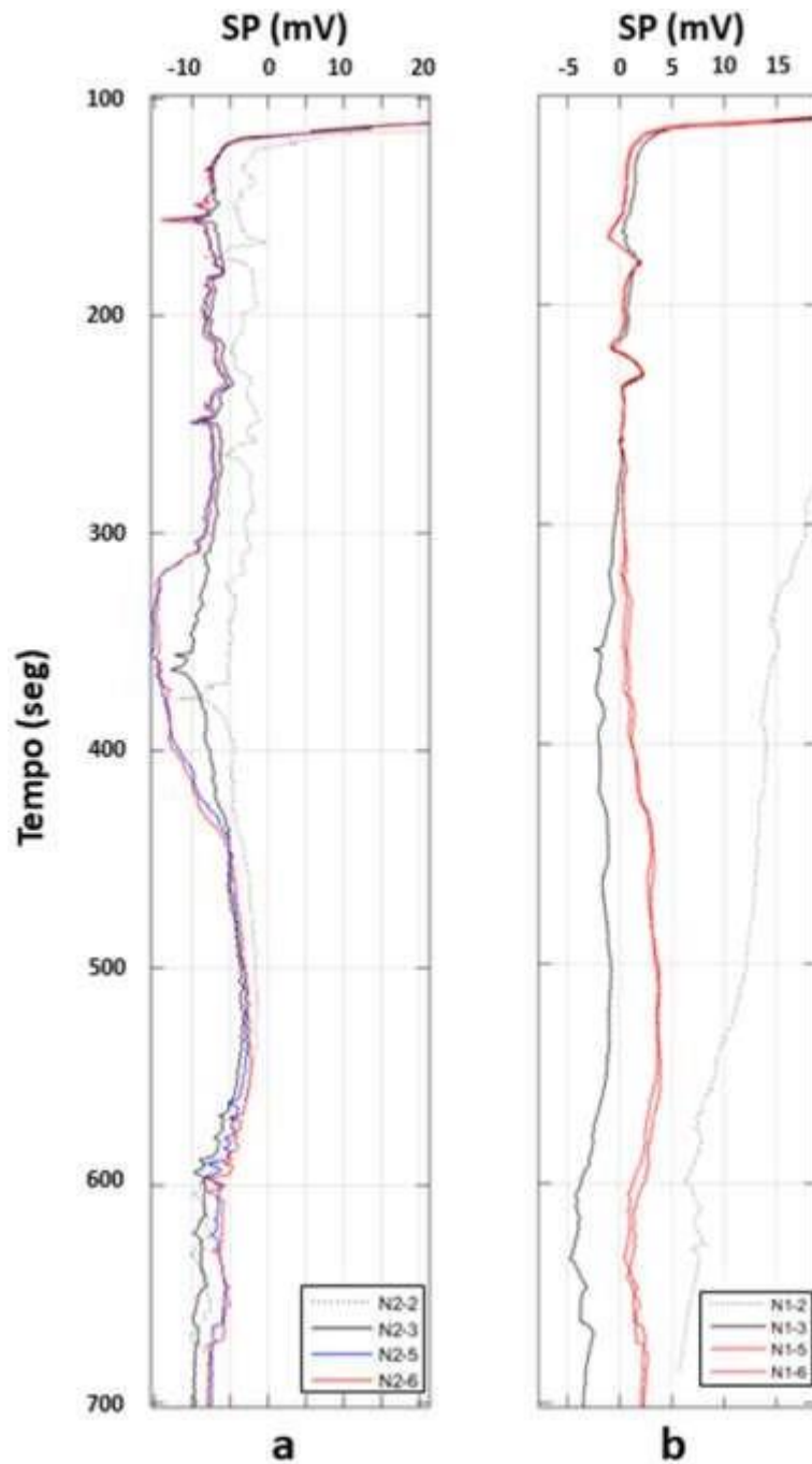
Figura 4.3 – Perfis de potencial espontâneo pelo tempo obtidos com sonda utilizando eletrodos Pb-PbCl utilizando os espaçamentos longo ( a , N2 - 100 cm) e curto ( b , N1 - 50 cm) entre os eletrodos de medida. As corridas 2 e 3, em ambos os arranjos, são realizadas em situação ambiente, enquanto as medidas 5 e 6 foram realizadas após rebaixamento do nível de água no poço e durante sua recuperação.
