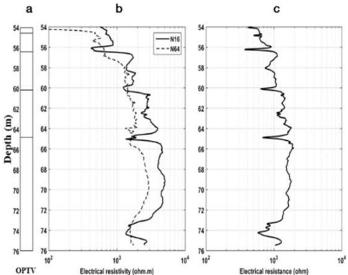
Figura 4.9 - Perfis obtidos no poço P2 do SCGR do IAG/USP. (a) Representação das fraturas com aberturas aparentes mais expressivas, da ordem de centímetros, nas profundidades de 54, 56, 60 e 65 metros, identificadas no perfil ótico. (b) Perfis de eletrorresistividade normal com espaçamento de 16" (linha sólida) e 64" (linha tracejada). (c) Perfil de resistência pontual (Adaptado de Kowalski, 2017).
