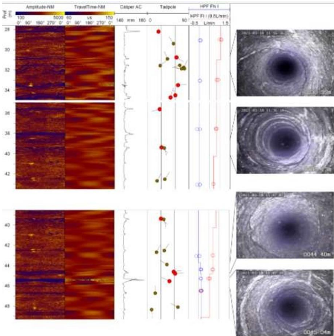
Figura 6.11 – Correspondência em profundidade entre as imagens obtidas com a câmera de inspeção, os perfis de imagem acústica e as medidas de fluxo vertical em condições ambiente e induzido, para os quatro intervalos de maior variação no fluxo, identificados pela sonda flowmeter.
