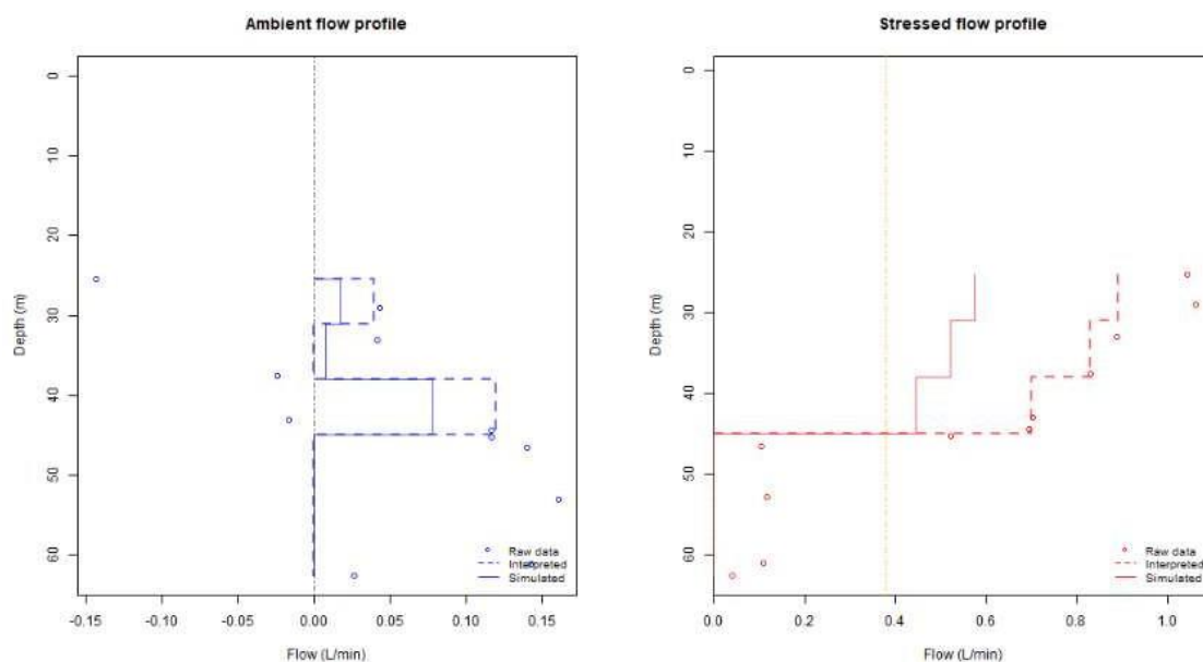
Figura 6.13 – Perfis obtidos pela perfilagem heat pulse em condições ambiente (azul) e durante bombeamento constante (vermelho) no poço P1. Os círculos indicam o fluxo medido, enquanto a linha contínua e tracejada representam o modelo simulado e interpretado, respectivamente.
