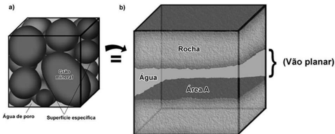
Figura 5.3 - Esquema representativo da equivalência entre as superfícies específicas de uma amostra porosa e das interfaces geradas por uma fratura.
