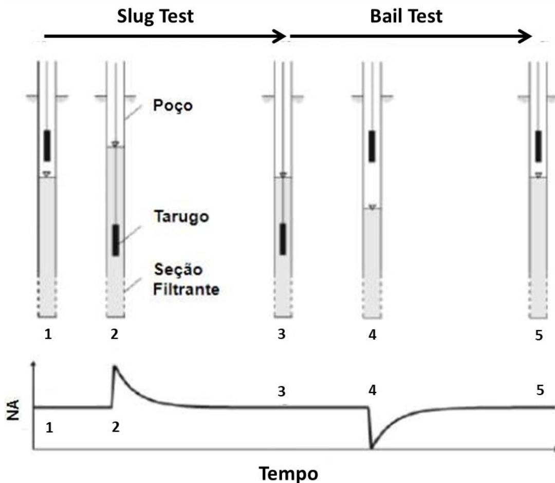
Figura 2.10 - Representação esquemática de um teste slug-bail. (1) Situação ambiente, indicando nível estático do poço. (2) Um tarugo sólido é inserido “instantaneamente” na água do poço elevando o NA. (3) O nível estático é recuperado após um período de tempo. (4) Retira-se “instantaneamente” o tarugo de dentro do poço, causando um rebaixamento do nível de água. (5) Após um novo período de tempo o nível estático é recuperado. As medidas de controle do nível de água no poço durante o levantamento podem ser feitas de maneira manual ou automatizada (Adaptado de Clark, 2003).
