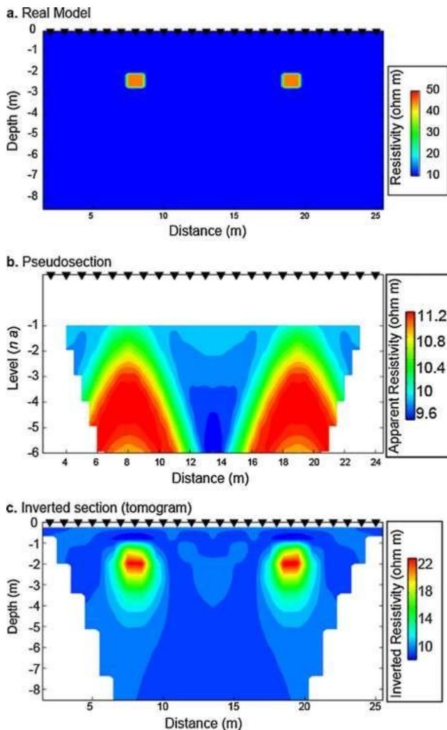
Figura 2.1 - Exemplo de inversão utilizando uma abordagem determinística e com vínculos de suavização. (a) Distribuição real da resistividade elétrica. (b) Pseudosseção obtida em função do arranjo dos eletrodos (triângulos em superfície). (c) Seção de resistividade elétrica invertida. (Revil et al., 2012).
