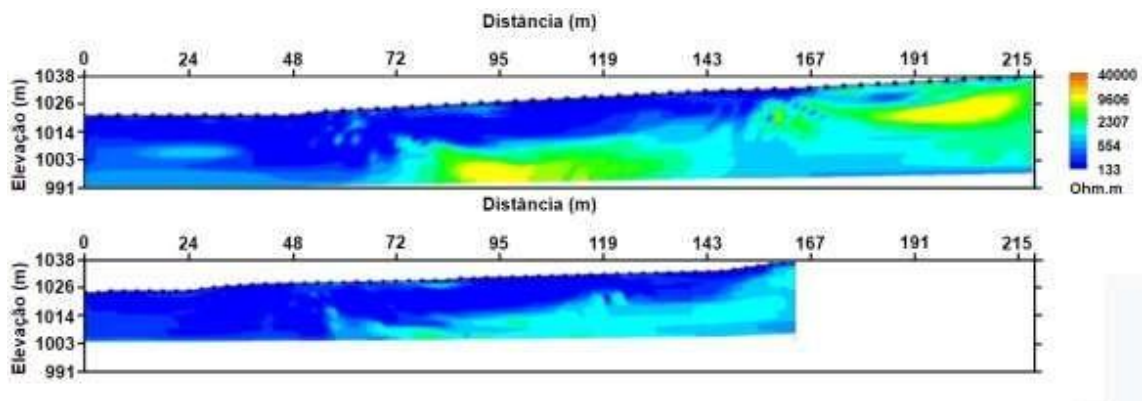
Figura 6.5 – Comparação entre as linhas ERT 02 (topo) e ERT 01 (base) com espaçamento entre os eletrodos de 3 e 4 metros, respectivamente. Foi necessário aumentar o espaçamento para atingir as unidades geoeletricas mais profundas e planejar as profundidades de cada um dos três poços que foram perfurados.
