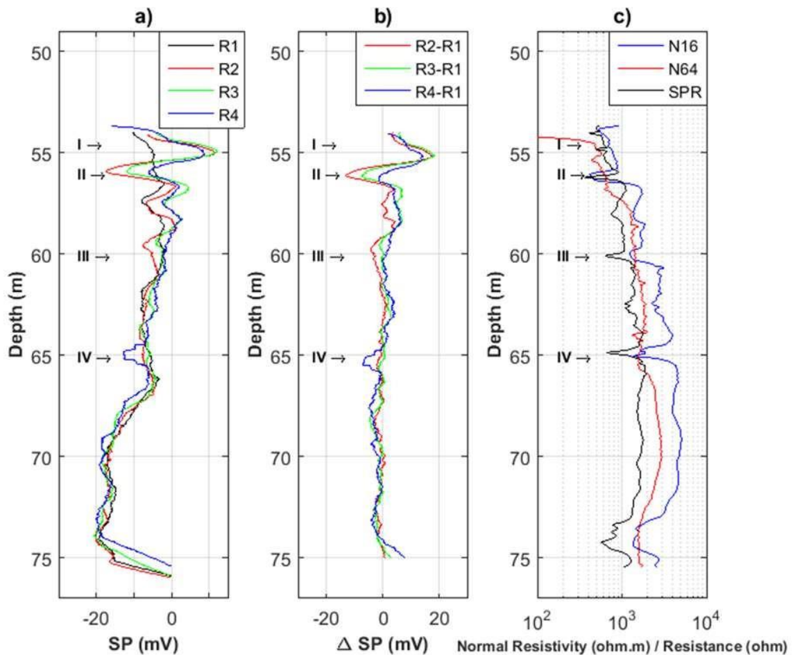
Figura 4.10 - Perfis elétricos obtidos no poço P2 do SCGR do IAG/USP. (a) Perfilagem do potencial espontâneo utilizando o espaçamento longo (100 cm) durante a subida. R1 indica a curva relacionada à situação ambiente, enquanto as curvas R2, R3 e R4 foram obtidas sequencialmente durante a recuperação
