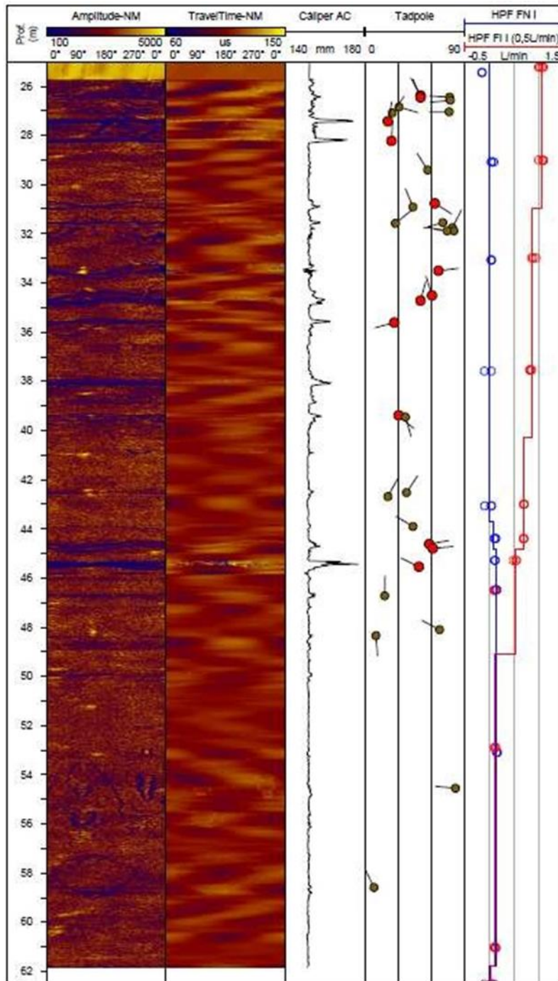
Figura 6.10 – Medidas heat pulse em condições de fluxo ambiente (linha azul) e induzido (linha vermelha), sendo as profundidades dos pontos de medida definidas pelo perfil de imageamento acústico. As medidas de fluxo induzido foram realizadas com bombeamento constante de aproximadamente 2 l/min e com um nível dinâmicode 4.4 m.
