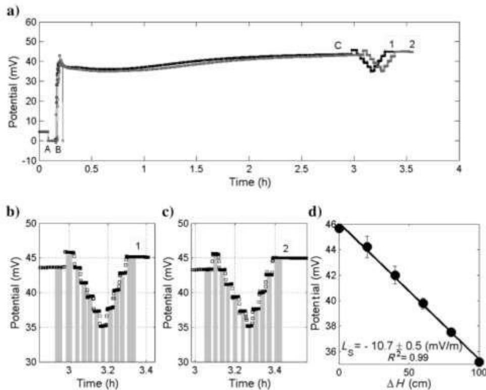
Figura 5.1 - Resultados experimentais obtidos em escala de laboratório ao simular uma perfilagem do potencial espontâneo (Mendonça et al., 2012). (a) Evolução das medidas do sinal SP após a substituição do eletrólito (ponto B) e mudanças em degraus de 20cm no gradiente hidráulico (ponto C), enquanto as medidas entre A e B foram monitoradas até atingir-se a estabilização do sinal. As curvas 1 e 2 representam medidas realizadas em dias consecutivos do potencial de origem eletrocinética, sendo apresentadas ampliadas em (b) e (c) , respectivamente. (d) Cálculo do parâmetro de acoplamento eletrocinético L_s a partir da relação linear entre o potencial elétrico e a altura da coluna de água.
