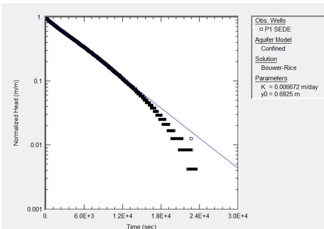
Figura 6.12 - Monitoramento do nível de água durante teste slug no poço P1. O cilindro de Nylon foi retirado após 6 horas desde o início do monitoramento. Para a estimativa de transmissividade do poço, ajustou-se linearmente os pontos do início do levantamento.
