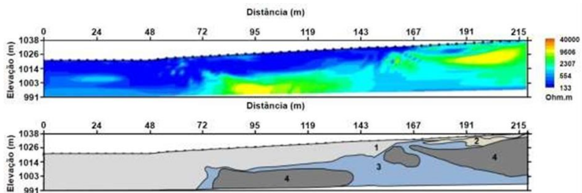
Figura 6.6 – Perfil ERT 02 próximo à nascente N9 onde foram identificadas as seguintes unidades: 1 – solo superficial com presença vegetação e raízes; 2 – solo mais seco com menor presença de matéria orgânica; 3 – Zona alterada; 4 – Rochas cristalinas.
