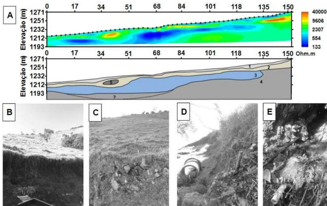
Figura 6.3 – Interpretação da seção ERT 06 e registros fotográficos dos afloramentos na vizinhança da nascente N15. (A) Perfil da distribuição de resistividade elétrica em subsuperfície e perfil interpretativo das unidades geoeletricas: 1 - Solo superficial com valores de condutividade associados à presença de raízes e vegetação; 2 - Solo seco com menor teor de matéria orgânica; 3 - Zona alterada, aumento da umidade com a profundidade até atingir a saturação; 4 - Rochas cristalinas; 5 - Matacão; (?) Profundidade até a rocha sã, ou camada 4, não atingida. (B) Solo superficial; (C) Fragmentos de rochas presentes na zona alterada; (D) Blocos de rochas presentes na zona alterada; (E) Nascente N15 entre fragmentos de rochas.
