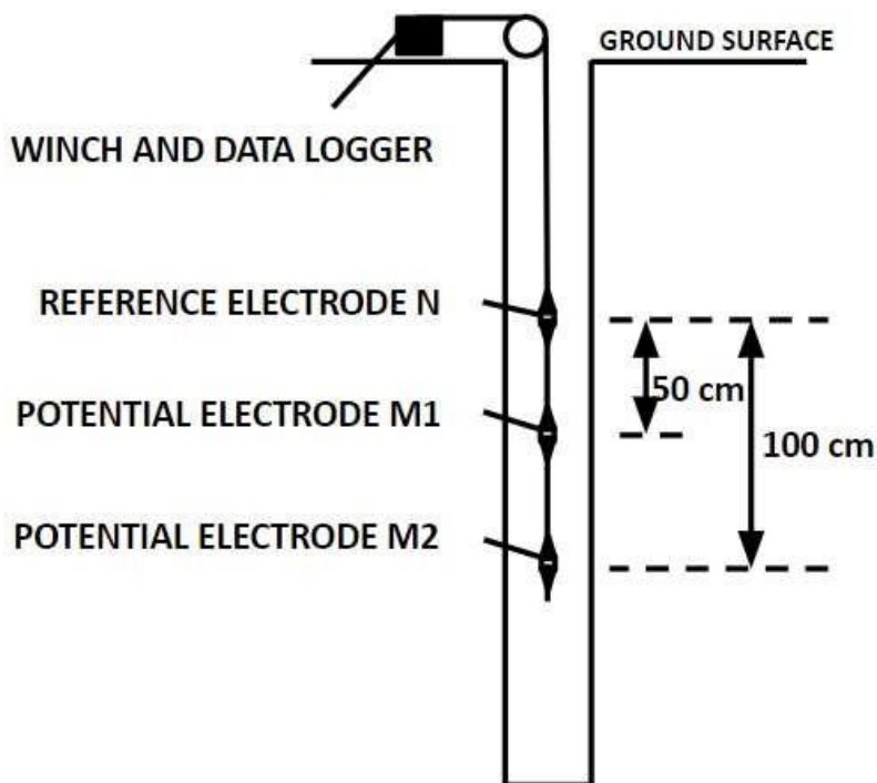
Figura 3.2 – Esquema ilustrativo da sonda utilizada na perfilagem geofísica do potencial espontâneo utilizando o espaçamento curto e longo, 50 e 100 cm respectivamente, entre os eletrodos de potencial e referência. Os eletrodos utilizados são feitos de chumbo e foram tratados com hipoclorito de sódio para evitar efeitos de polarização em suas superfícies. Na superfície do terreno fica a unidade contendo um voltímetro de alta impedância para realizar as medições, um sistema para registro e armazenamento dos dados, além do transdutor de giros para identificar as profundidades de cada medida.
