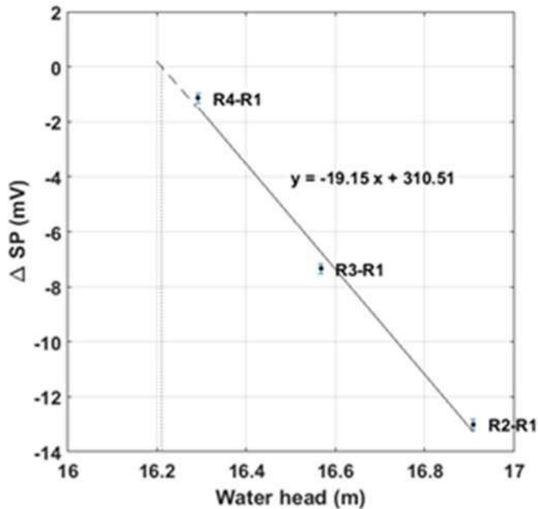
Figura 4.11 - Diferenças do potencial espontâneo obtidos no poço P2 na profundidade de 56 metros, utilizando o espaçamento longo durante a descida da sonda, em relação ao potencial medido em situação ambiente. Foi realizado um ajuste linear para determinar o valor em que o potencial é nulo, neste caso 16.2 m, correspondendo ao valor de pressão aplicado sobre a fratura (Kowalski et al., 2020).
