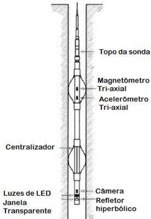
Figura 2.5 – Esquema de sonda utilizada na perfilagem ótica para imageamento da parede do poço. Os centralizadores são compostos por materiais não magnéticos para evitar distorções na orientação da sonda com base nos sensores magnéticos (Adaptado de Wild et al., 2002).
