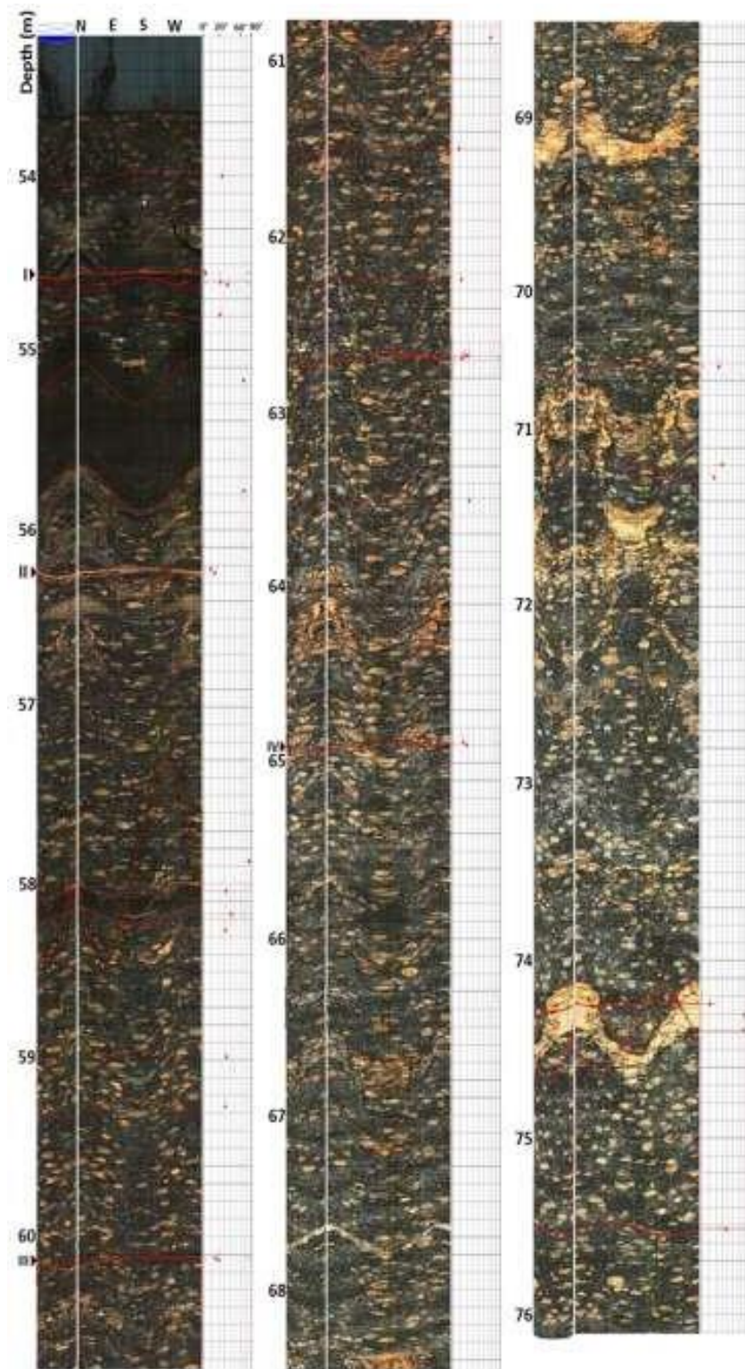
Figura 4.8 - Perfil ótico no intervalo aberto do poço P2 localizado no SCGR do IAG/USP. As linhas vermelhas indicam a localização de fraturas, enquanto os alfinetes indicam a orientação e inclinação das estruturas identificadas. As fraturas que apresentaram abertura aparente da ordem de 1 cm ou mais (apenas 4) estão indicadas pelos números I a IV na figura.
