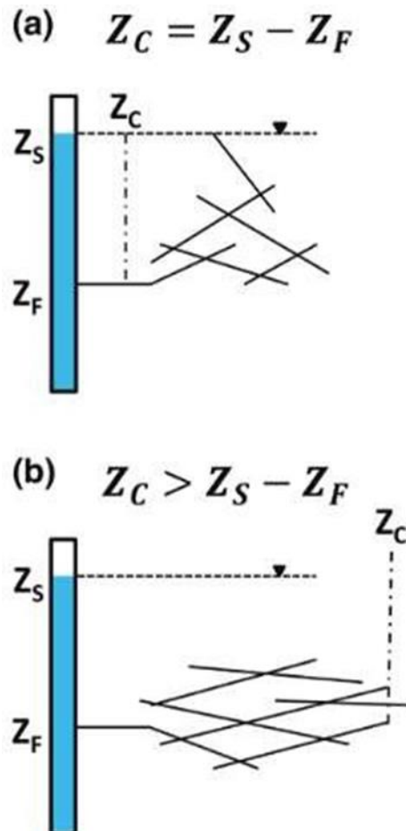
Figura 3.5 - Esquema conceitual descrevendo dois modelos para fraturas interceptadas por um poço e conectadas a um sistema aquífero livre (a) e confinado (b). Z_S e Z_C indicam o nível estático e a carga hidráulica associada ao potencial nulo, respectivamente, enquanto Z_F indica a profundidade do nível de fratura.
