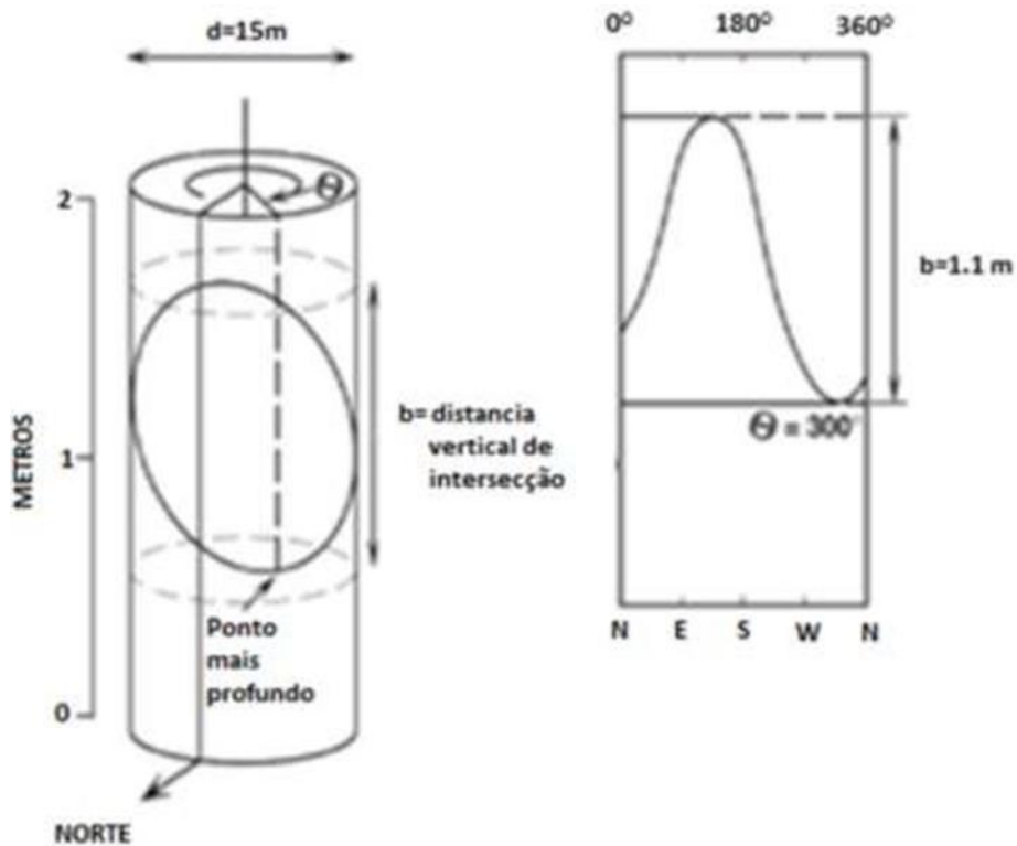
Figura 2.6 – Representação de uma fratura interceptada pelo poço e sua projeção planificada. b representa a distância vertical entre os pontos que interceptam a fratura, \theta é o ângulo que define a orientação da fratura e d o diâmetro do poço (Adaptado de Paillet & Ellefsen, 2005).
