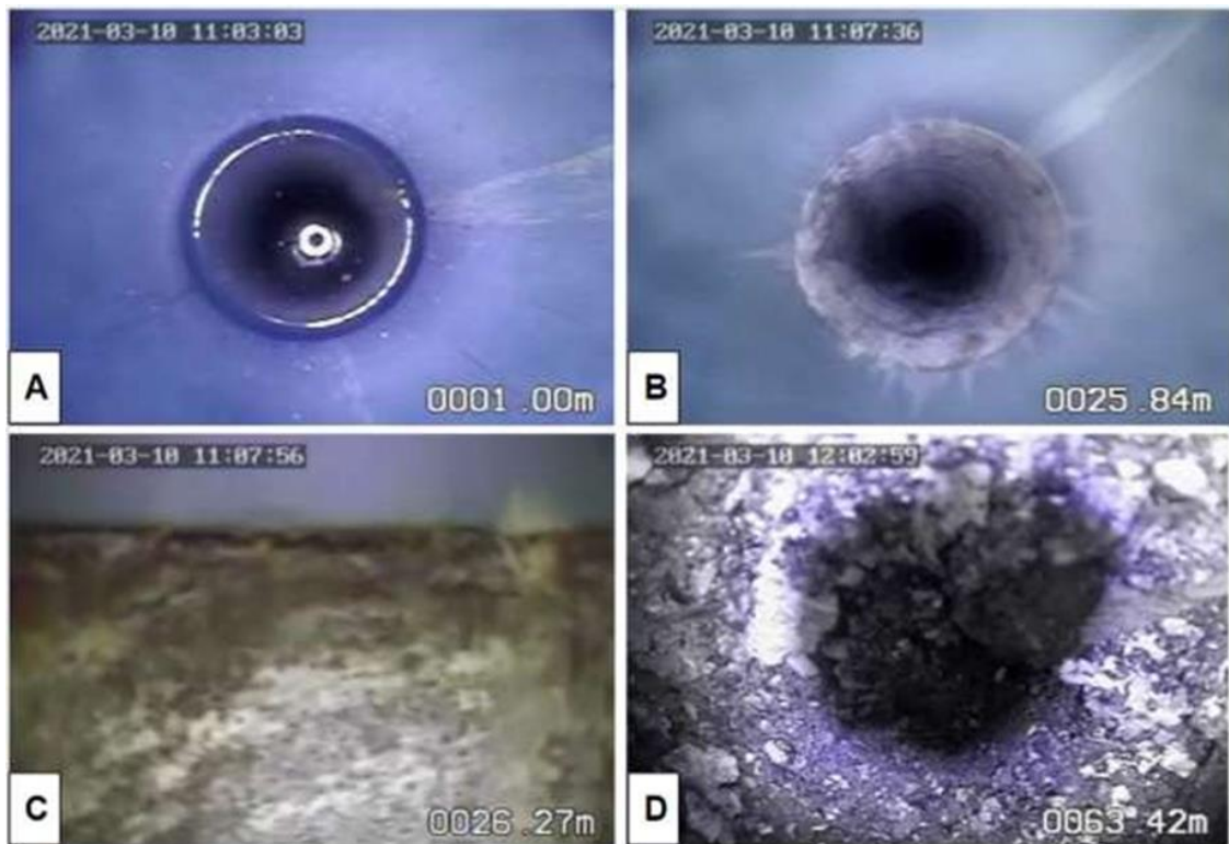
Figura 6.8 - Imagens obtidas pela inspeção por câmera do poço P1: (A) Nível de água estático em 1.3 metros de profundidade; (B) Final do revestimento em 26.15 metros; (C) Final do revestimento, filmado pela câmera lateral; (D) Fundo do poço (sombra da câmera) em 63.42 metros.
