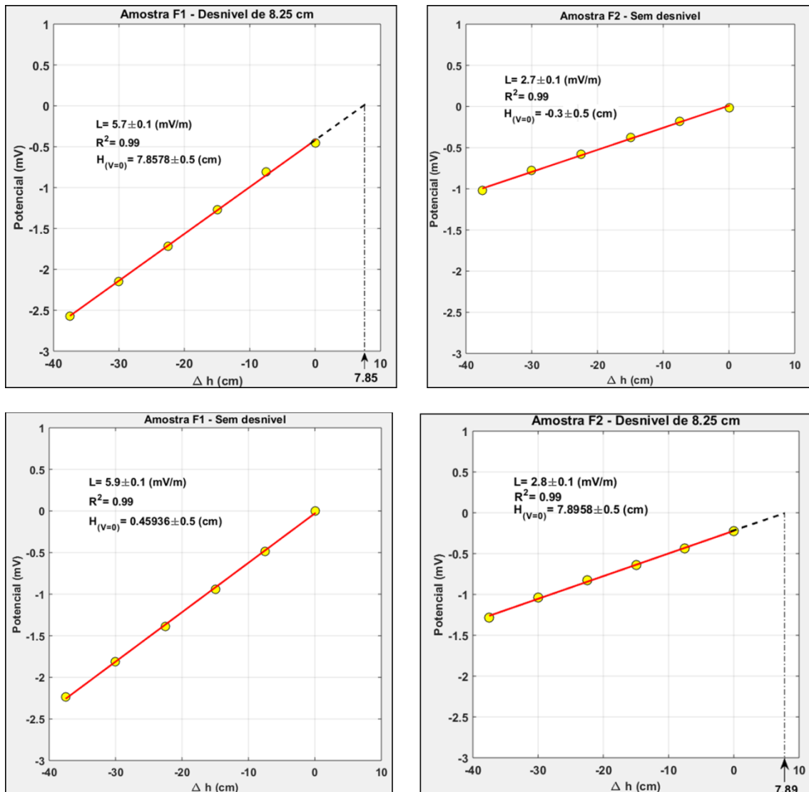
Figura 5.6 - Medidas do potencial elétrico nas células vermelha (F1) e azul (F2) para duas situações de cargas hidráulicas iniciais desconhecidas. (Topo) O barrilete azul (F1) foi deslocado em 8.25 cm; (Base) O barrilete vermelho (F2) foi deslocado inicialmente em 8.25 cm.
