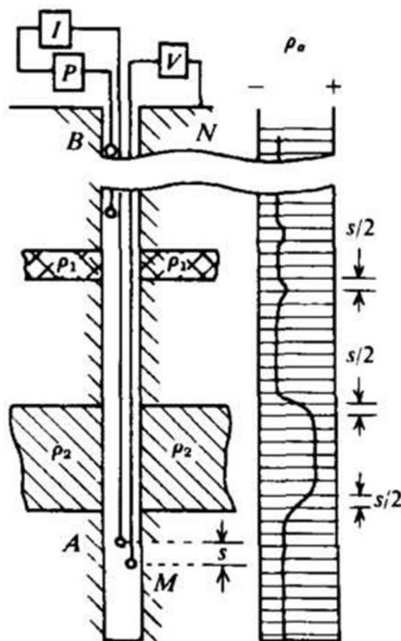
Figura 2.3 – Esquema ilustrativo da perfilagem normal para determinar a resistividade elétrica em uma camada fina ( \rho_1 ) e espessa ( \rho_2 ). s é o espaçamento entre os eletrodos A e M, o ponto P representa uma bateria ou outra fonte de energia elétrica, e os pontos I e V realizam medidas da corrente e do potencial elétrico resultante (Adaptado de Telford et al., 1990).
