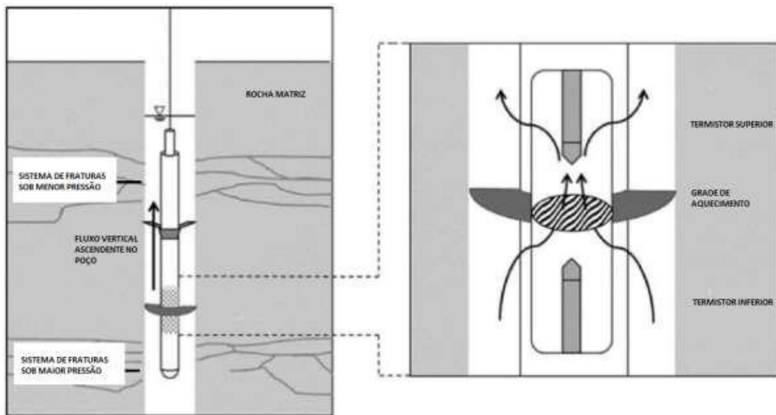
Figura 2.8 – Esquema ilustrativo do funcionamento de uma sonda heat pulse flowmeter . A diferença de pressão entre zonas fraturadas resulta em uma movimentação de água ao longo do poço e pode ser determinada através da análise do tempo que uma fração de água aquecida leva para atingir um dos termistores instalados dentro da sonda (Adaptado de Busse et al., 2016). O tempo de medida e grau de aquecimento são dimensionados para desconsiderar efeitos convectivos resultantes do aquecimento.
