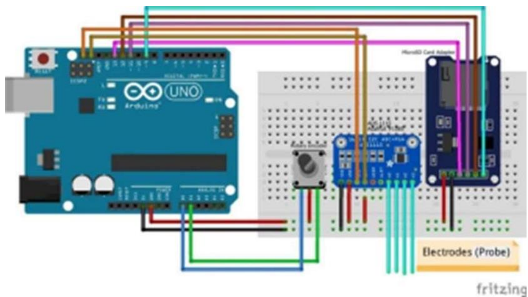
Figura 4.4 – Circuito que integra as medidas de profundidade e do potencial elétrico. Utilizou-se uma placa Arduino UNO conectada ao encoder, para registro da movimentação da sonda no poço, conversor analógico-digital (ADS 1115) e módulo MicroSD Card Adapter para armazenamento das leituras. Os códigos utilizados são apresentados no Apêndice II.
