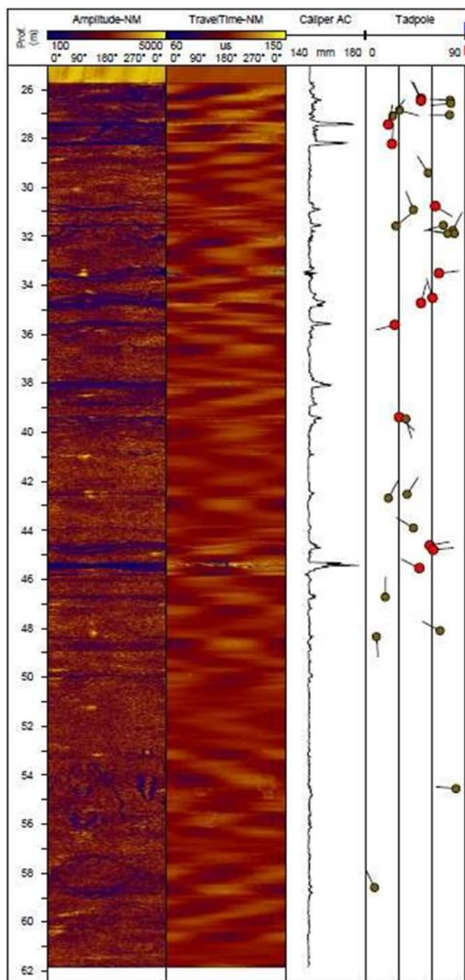
Figura 6.9 - Perfil de imageamento acústico mostrando a amplitude das ondas refletidas na parede do poço, o tempo de trânsito e o perfil caliper associado. O gráfico do tipo tadpole representa cada fratura por um símbolo tipo alfinete, sendo a coloração vermelha indicativa de aberturas maiores que 1 cm. A posição e orientação do alfinete indicam a atitude das fraturas identificadas.
