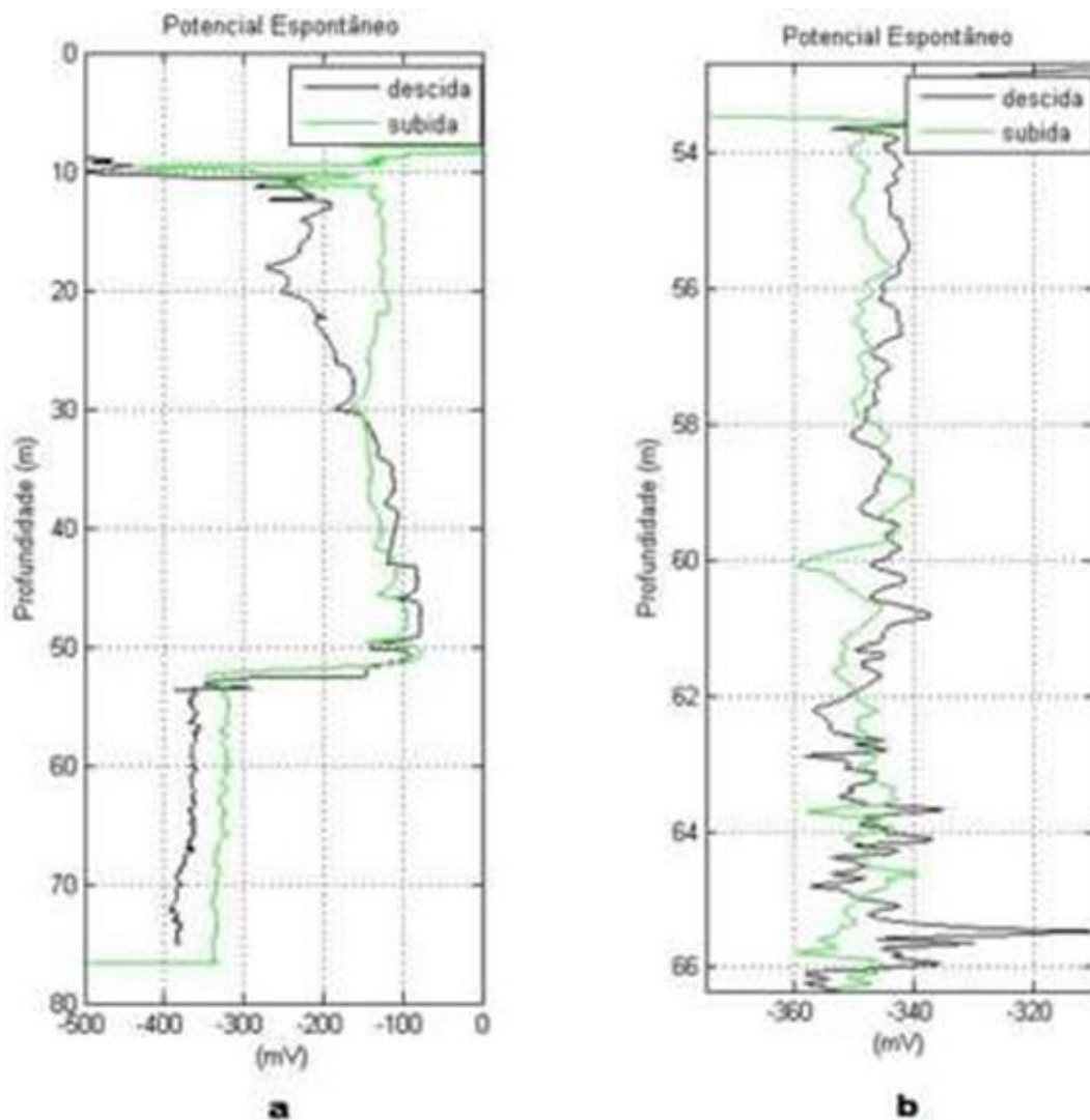
Figura 4.1 – Perfis do potencial espontâneo obtidos no poço P2 do Sítio Controlado de Geofísica Rasa do IAG/USP durante a descida e subida da sonda para comparação da repetibilidade das leituras. (a) Perfil do potencial espontâneo para todo o poço, incluindo o intervalo revestido de 0 a 53 m. Merece destaque a variação abrupta relacionada à transição do final do revestimento para a rocha sã. (b) Ampliação do trecho inicial do perfil do potencial espontâneo no intervalo aberto do poço, mostrando que a diferença entre as curvas atinge valores maiores que 50 mV.
