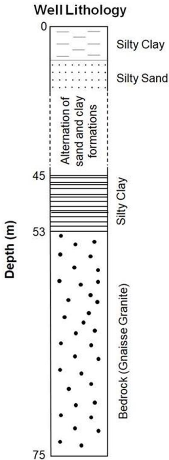
Figura 4.7 - Perfil litológico do poço P2 localizado no Sítio Controlado de Geofísica Rasa do IAG/USP onde foram realizados os primeiros testes de conceito da metodologia proposta. O poço é revestido ao longo das camadas sedimentares até 53 metros de profundidade e aberto até o fundo (80 m). A presença de uma camada espessa de argila siltosa entre 45 e 53 metros atua como uma barreira hidráulica para o fluxo entre as unidades aquíferas mais rasas e o sistema de fraturas mais profundo.
