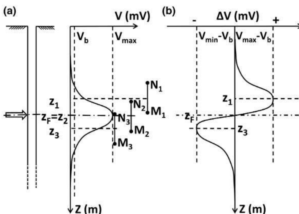
Figura 3.7 – Potencial elétrico esperado para o fluxo de água em uma fratura, na profundidade Z_F , com sentido da formação para o poço, medido por um par de eletrodos M-N. (a) Potencial espontâneo com polaridade positiva. (b) Diferença entre o potencial espontâneo entre os eletrodos. V_b é o valor base medido em intervalos distantes das fraturas hidráulicamente ativas, enquanto V_{max} e V_{min} são valores limites para a variação do sinal SP tal que V_{max} - V_b = V_b - V_{min} .
