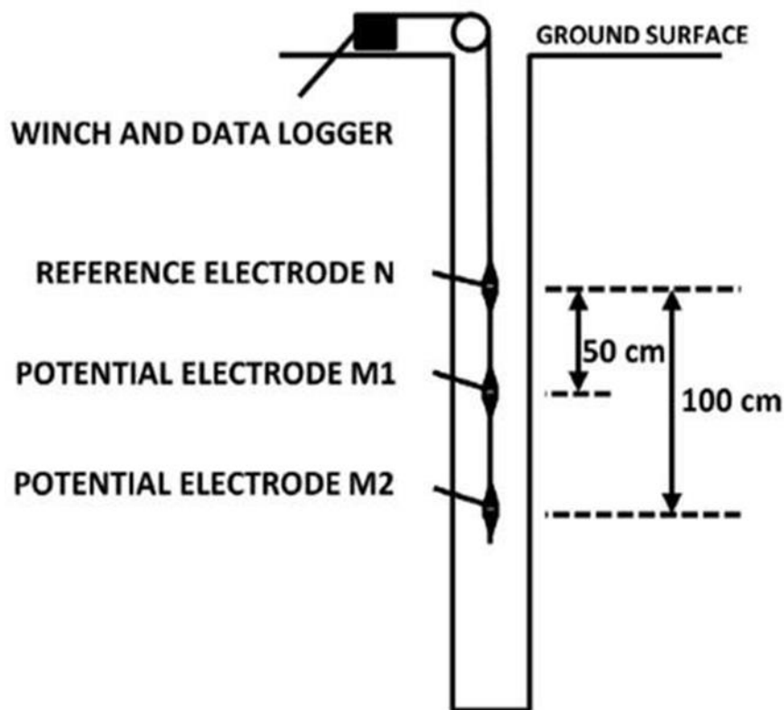
Figura 4.5 - Arranjo de campo montado para realizar a perfilagem geofísica do potencial espontâneo. Em superfície ficam localizados módulos de registro de dados e profundidade, enquanto no poço é movimentada uma sonda com dois espaçamentos entre os eletrodos de 50 cm e 100 cm, curto e longo, respectivamente.
