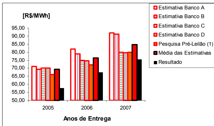
Gráfico 2: Comparação entre Preços Finais e Estimativas de Bancos Leilão de Energia Existente de 07/12/2004 Fonte: Relatórios de Bancos. Elaboração Própria
