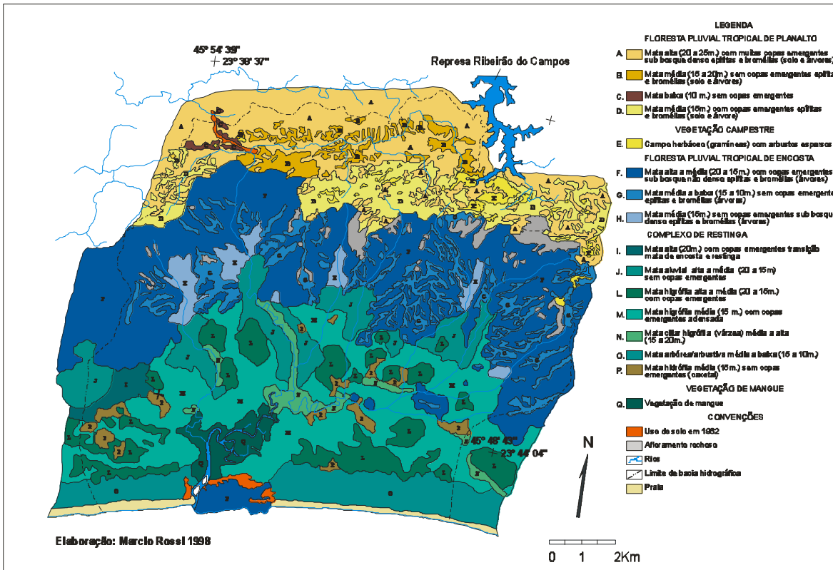
Figura 08: Mapa da cobertura vegetal natural da Bacia do Guaratuba.
