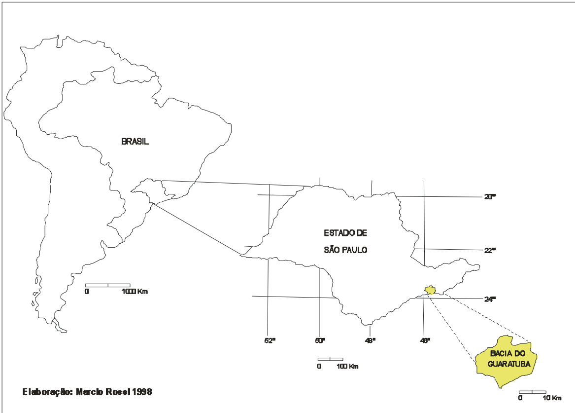
Figura 01: Mapa de localização da Bacia do Guaratuba.
