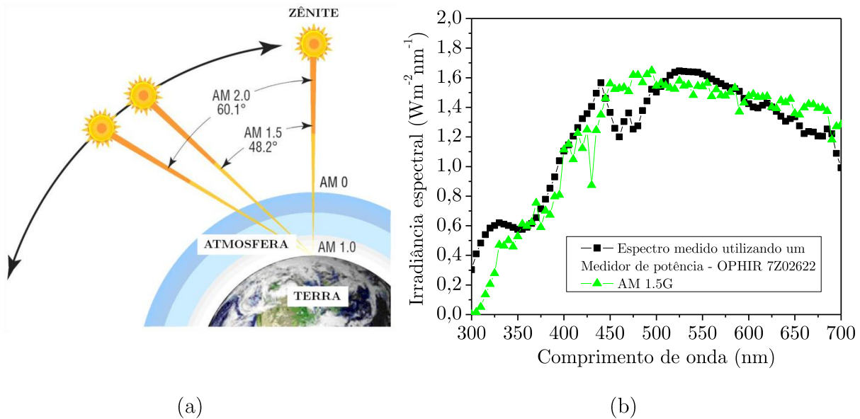
Figura 19 - (a) Diferentes condições para caracterização de células solares. (b) Curva de Irradiância padrão (AM 1.5) e o calculado em nosso laboratório para a caracterização dos dispositivos.
