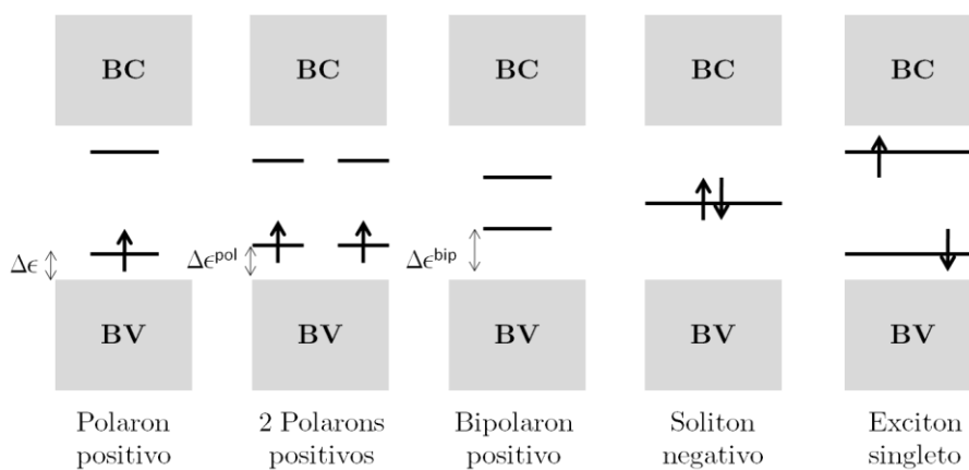
Figura 5 - Esquema de energia e as excitações elementares de um semicondutor.
