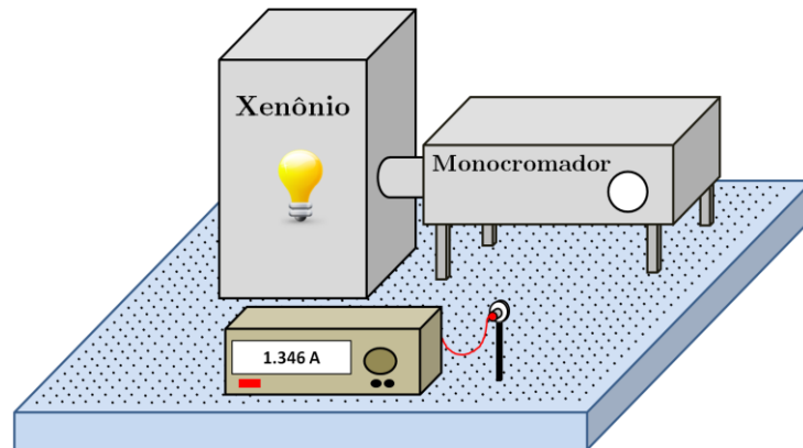
Figura 20 - Montagem experimental para calibração e medição de Irradiância.
