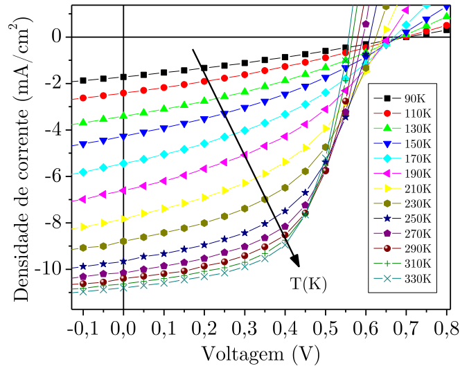
Figura 41 - Curvas J-V sob iluminação ( 100\text{mW}/\text{cm}^2 ) medidas em função da temperatura.
