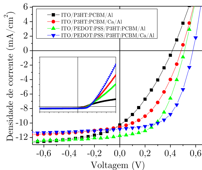
Figura 22 - Curvas J-V dos dispositivos contendo diferentes contatos.
