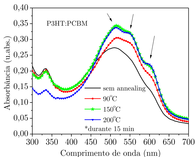
Figura 36 - Espectro de absorção do filme de P3HT:PCBM, tratado termicamente em diferentes temperaturas.
