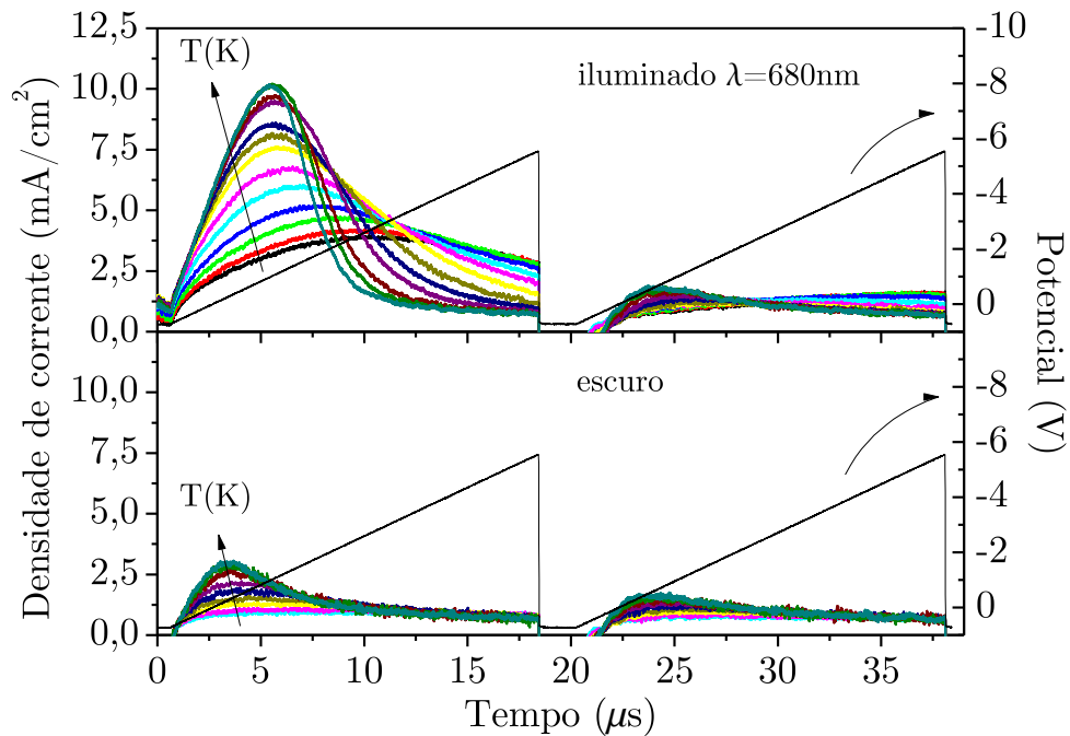
Figura 43 - Medidas de corrente de extração (foto-CELIV) realizadas sob iluminação (parte superior) e no escuro (inferior). Cada curva é representada pela média de 500 medidas.
