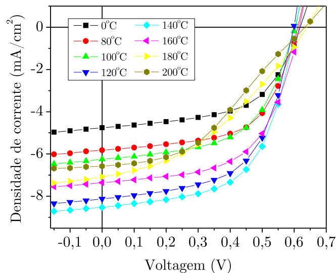
Figura 33 - Curvas J-V medidas para os dispositivos tratados termicamente em diferentes temperaturas.
