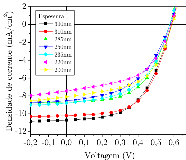
Figura 27 - Curvas J-V medidas para os dispositivos com diferentes espessuras de camada ativa.
