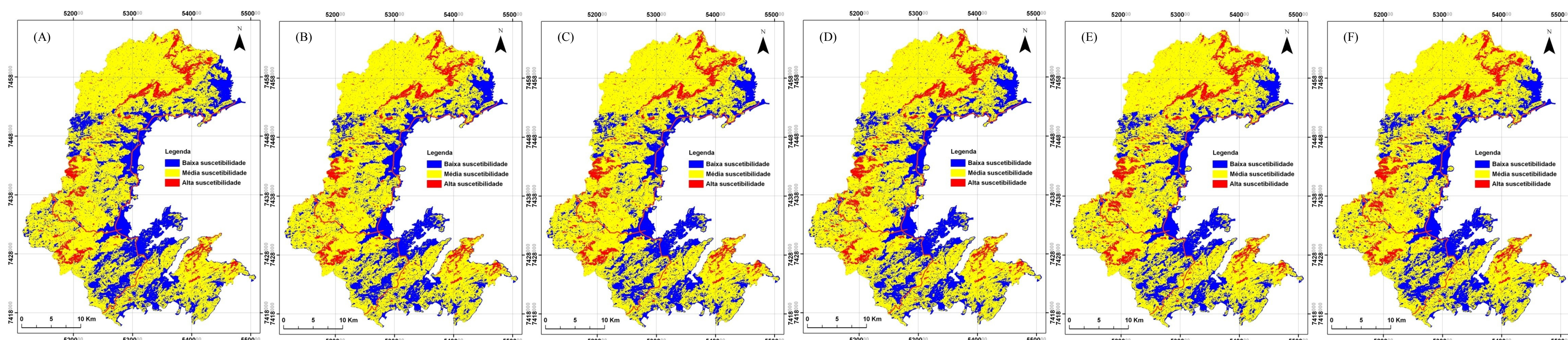
Figura 30- Cartas de suscetibilidade geradas a partir do MDE ASTER 15. (A) 1973, (B) 1986, (C) 1993, (D) 2000, (E) 2007 e (F) 2008
