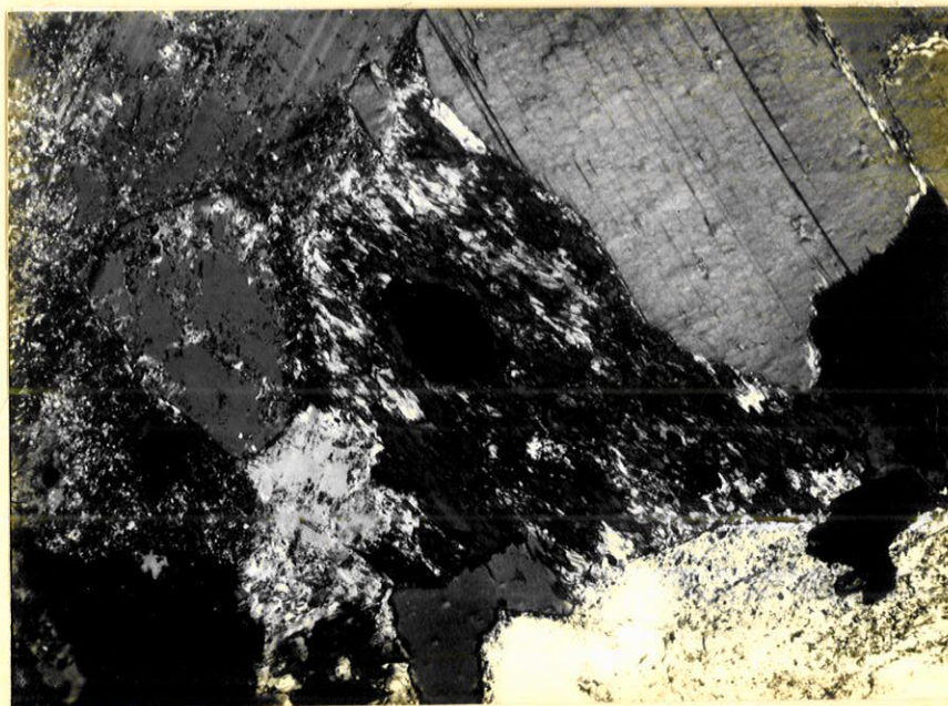
Fotomicrografia 18 - Cristal de riebeckita (cinza escuro) formando-se às expensas de biotita (branca e cinza claro). Ao lado aparece um outro cristal de biotita, porém, inalterado. Nícois cruzados. Aumento:
