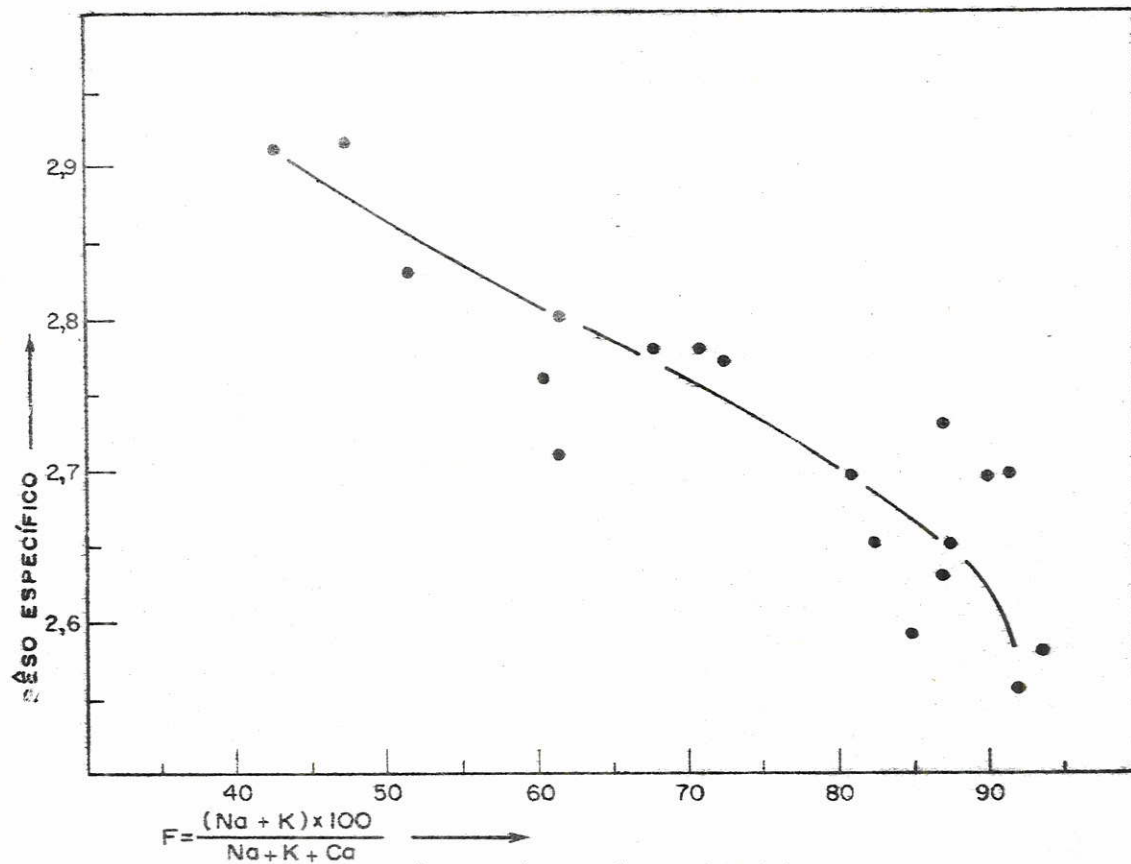
Fig.18- Gráfico relacionando o pêso específico e o índice félsico (F) das rochas de Itapirapuã.
