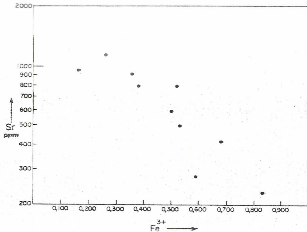
Fig.15 - Gráfico reunindo a molécula de Egirina, expressa pela proporção atômica de Fe 3+ , e o conteúdo em Sr dos piroxênios de Itaipapuá.
