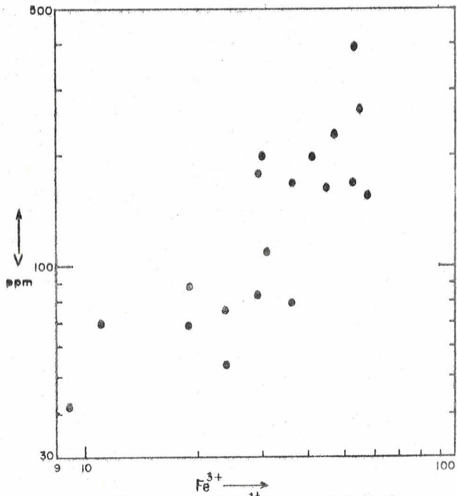
Fig.27- Relação entre V e Fe 3+ nas rochas de Itapirapuã.
