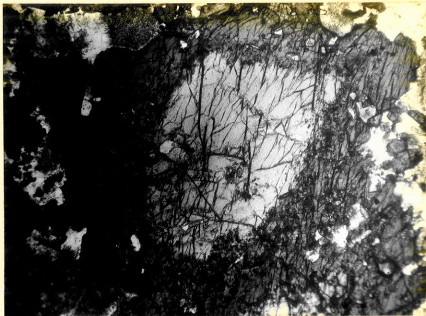
Fotomicrografia 3 - Cristal de piroxênio mostrando estrutura zonada. As partes centrais (cinza claro) correspondem à variedade soda-augita, enquanto que as bordas são de egirina-augita. Nícois paralelos. Aumento: 20 X.
