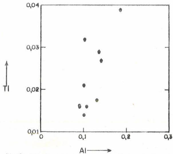
Fig.13 - Relação entre as proporções atômicas de Ti e Al nos piroxênios de Itapirapuã.
