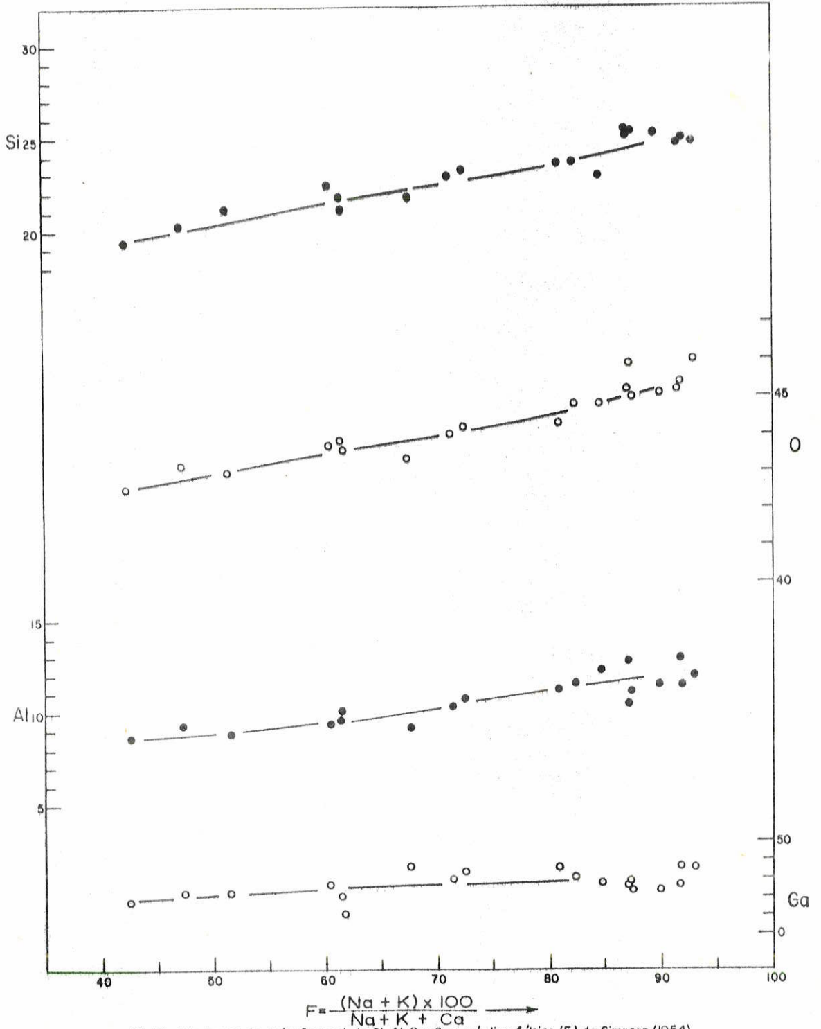
Fig. 21- Diagramas de variação reunindo Si, Al, O e Ga e o índice félsico (F) de Simpson (1954). Elementos principais expressos em % em peso e elementos traços em ppm.
