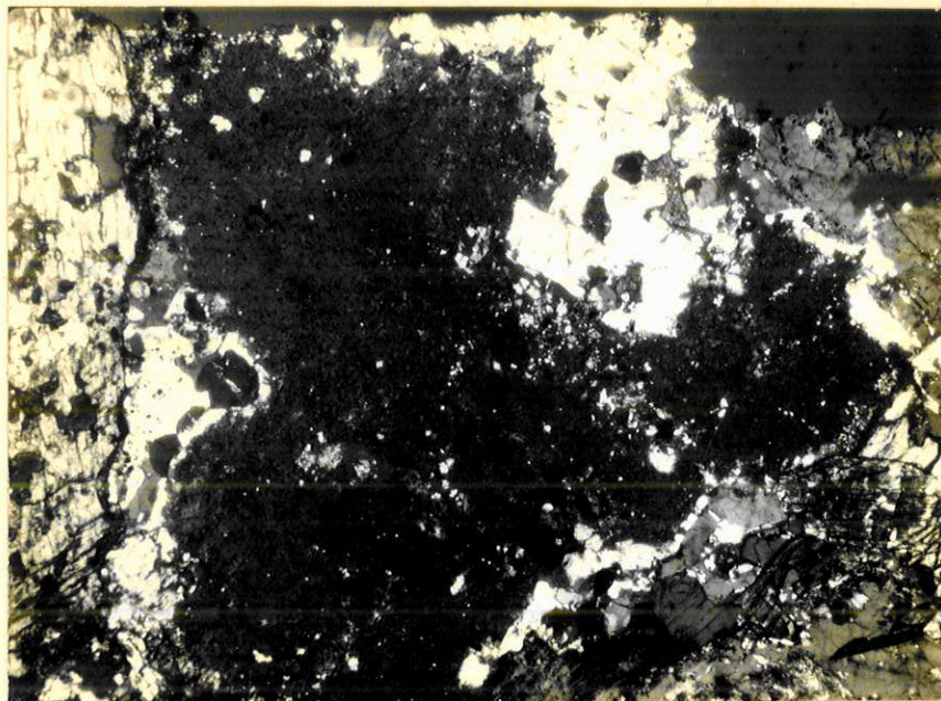
Fotomicrografia 2 - Agregado mineralógico semi-isotrópico (cinza escuro) resultante da alteração de nefelina. No seu interior vêem-se pontos claros correspondentes à cancrinita e calcita (maior relêvo). Nas bordas do agregado, ainda aparecem remanescentes (branca) do antigo cristal de nefelina, bem como cancrinita (alguns pontos cinzentos) e calcita (grânulos de maior relêvo). Nícois sub-paralelos. Aumento: 40 X.
