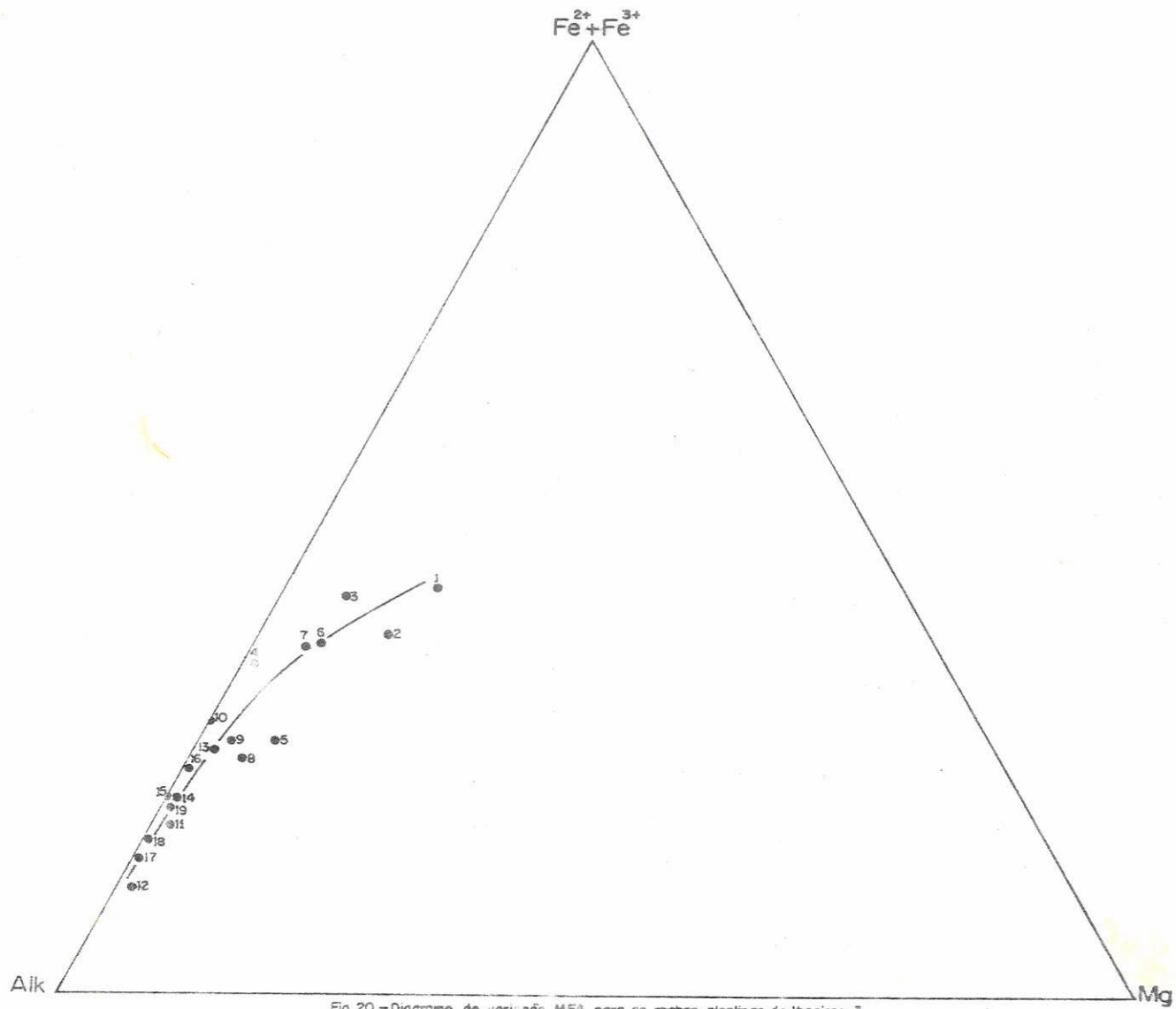
Fig. 20 - Diagrama de variação MFA para as rochas alcalinas de Itaipapuã.
