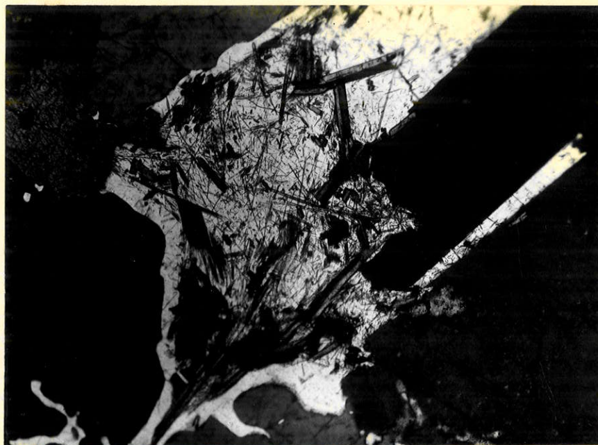
Fotomicrografia 5 - Mineral A, mostrando hábito alongado e geminação, imerso em cristais de cancrinita (branca). Lado esquerdo, parte inferior da foto, vê-se cancrinita (branca) formando-se a partir de nefelina (cinza médio e escuro). À direita da foto, cristais de feldspato alcalino (cinza) exibem contornos regulares e, à esquerda, lado superior, cristais de egrina-augita. Nícois cruzados. Aumento: 50 X.
