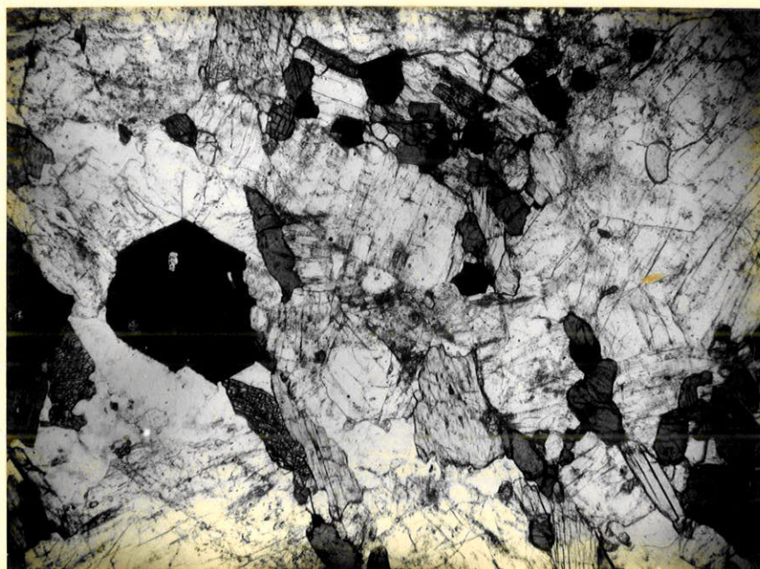
Fotomicrografia 12 - Wollastonita-melanita-nefelina sienito. Cristais idiomórficos de melanita (preta) associados à egiro-augita (cinza médio a escuro) e wollastonita (cinza claro, clivagem paralela ao alongamento e relêvo médio). O restante da rocha (cinza esbranquiçado) é constituído de nefelina e, em menor quantidade, de feldspato alcalino. Nícois paralelos. Aumento: 20 X.
