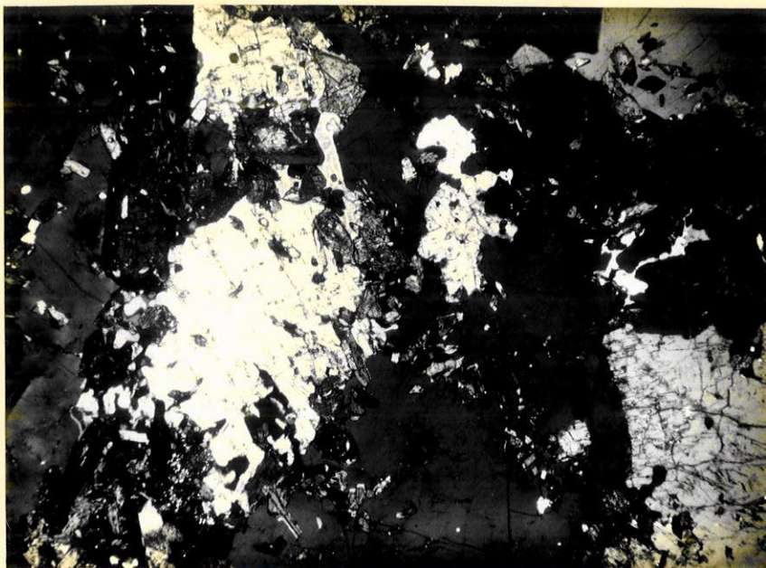
Fotomicrografia 7 - Nefelina sienito. Cristais de nefelina (branca a cinza claro) e cancrinita (formas irregulares esbranquiçadas) em associação com feldspato alcalino (cinza médio a escuro). Vêm-se também cristais zonados de egirina-augita e de titanita (minerais idiomórficos de relêvo alto). Nícois cruzados. Aumento: 20 X.
