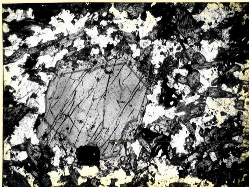
Fotomicrografia 10 - Biotita melteigito. Fenocristal zonado de soda-augita imerso em matriz constituída de soda-augite, nefelina e cancrinita (branca) e titanita (mine ralis idiomórficos de relêvo alto). Nícois paralelos. Au- mento: 20 X.
