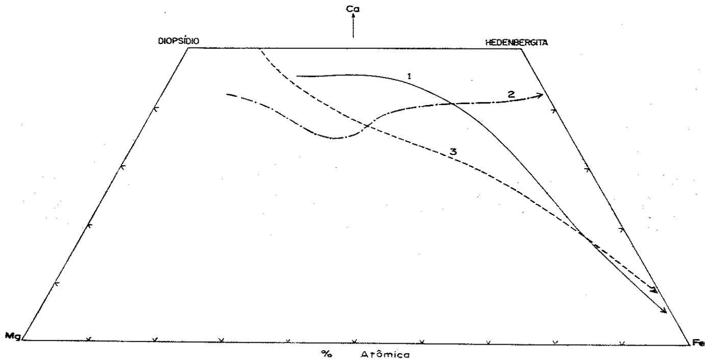
Fig. 10—Diagrama Ca-Mg-Fe para clinopiraxênios. 1, sentido de cristalização dos piraxênios de Itapetuba; 2, dos piraxênios de Skarogaard; e 3, dos piraxênios de Moratu.
