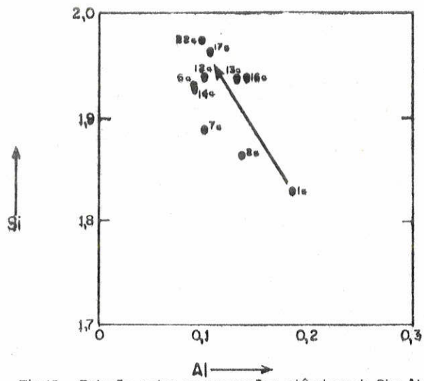
Fig.12 - Relação entre as proporções atômicas de Si e Al nos piroxênios de Itapirapuã.
