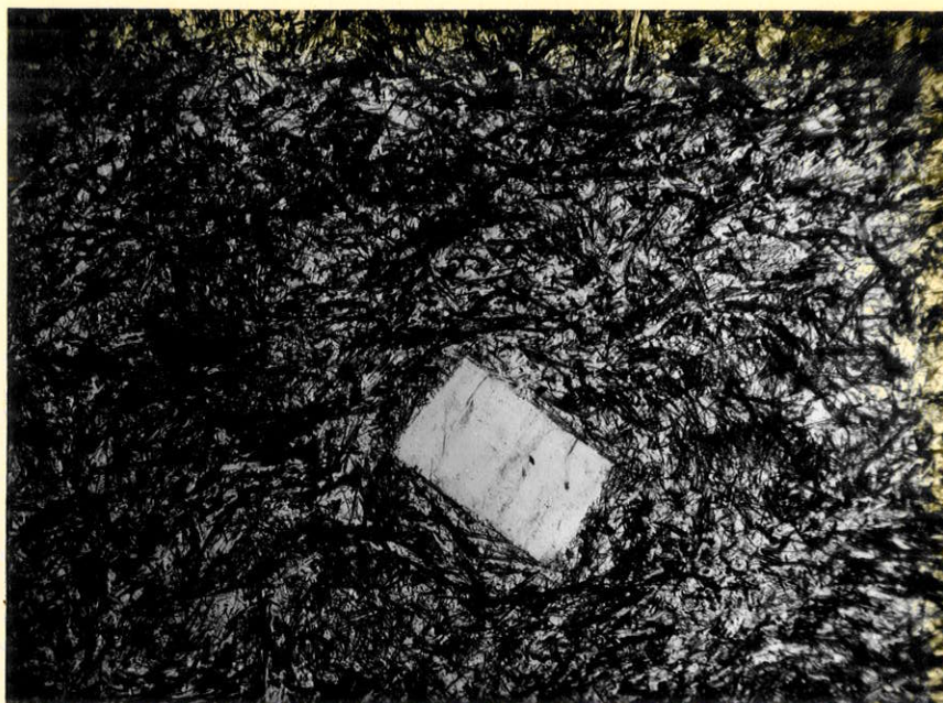
Fotomicrografia 15 - Tinguai to. Textura tinguai tica. Cris- tais aciculares de pirox nio dispersos ca ticamente e associados a material de c r branca e composto de can- crinta e feldspato alcalino. V -se tamb m um fenocris- tal de nefelina mostrando contornos regulares. N cois paralelos. Aumento: 20 X.
