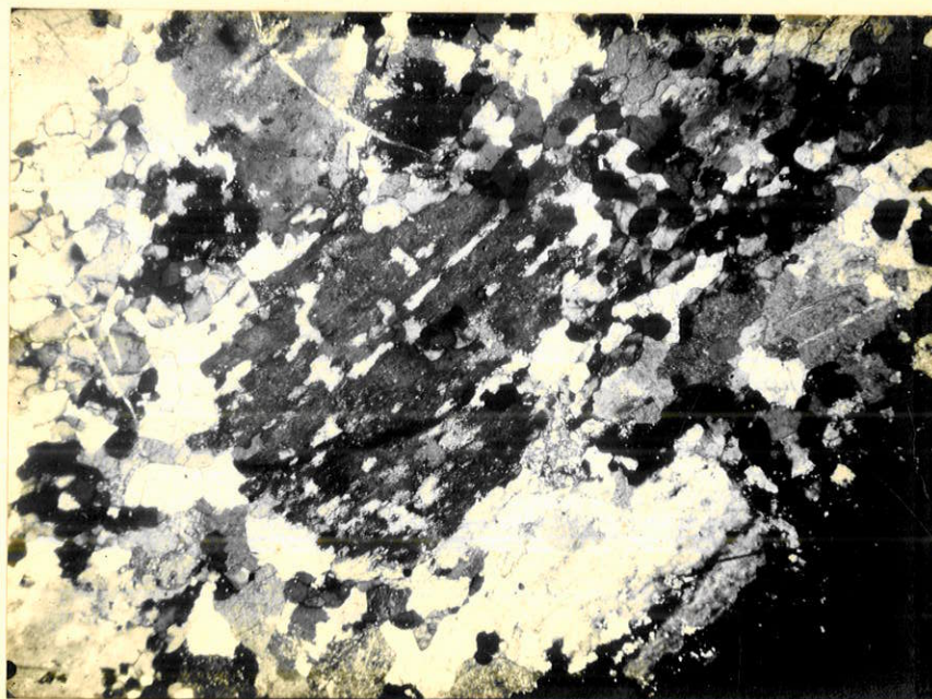
Fotomicrografia 16 - Carbonatito. Cristal de feldspato al- calino (cinza escuro) sendo substituído por calcita (branca e cinza claro e rel vo vari vel) nas suas partes marginais e ao longo das linhas de clivagem. V em-se tamb m cris- tais equidimensionais de apatita (cinza escuro e rel vo al- to). N cois cruzados. Aumento: 20 X.
