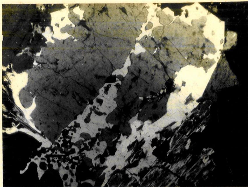
Fotomicrografia 1 - Cancrinita (branca) formando-se às expensas de nefelina (cinza). Cristal grande de egirina-augita, mostrando clivagem, na parte inferior da foto, lado direito. Nícois cruzados. Aumento: 40 X.
