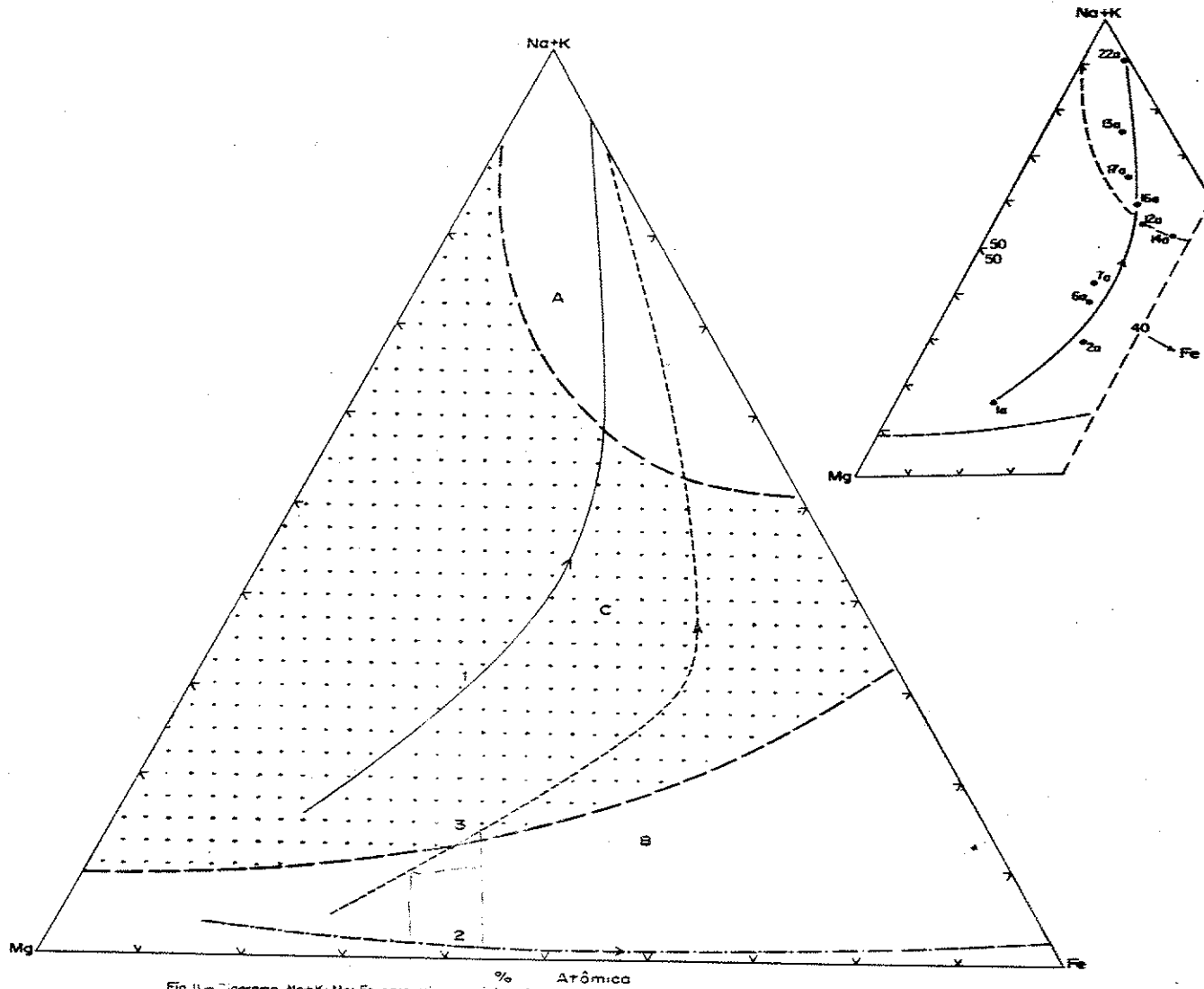
Fig. 11 - Diagrama Na+K, Mg, Fe para clinopiroxênios. A, campo dos piroxênios sodícos; B, campo dos piroxênios cálcicos e C, região de imiscibilidade (cf. Aoki, 1964). 1, sentido de cristalização dos piroxênios de Itapirapuã; 2, dos piroxênios de Skargaard e 3, dos piroxênios de Moratu.
