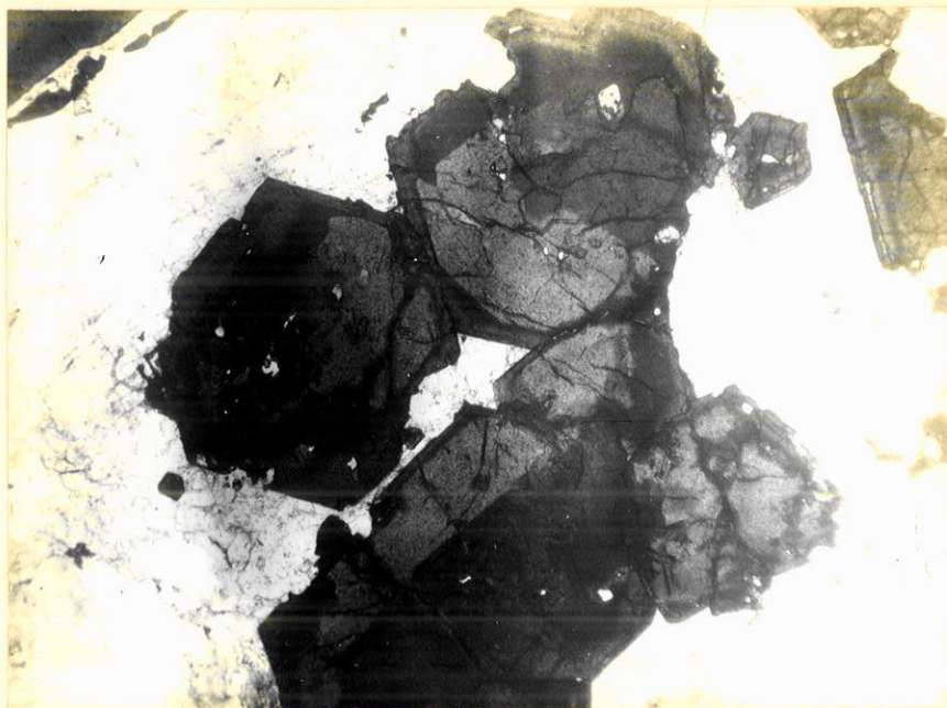
Fotomicrografia 4 - Cristais idiomórficos de granada mostrando estrutura zonada. Área branca, sem relêvo, é composta de nefelina e feldspato alcalino. Nícois paralelos. Aumento: 22,5 X.
