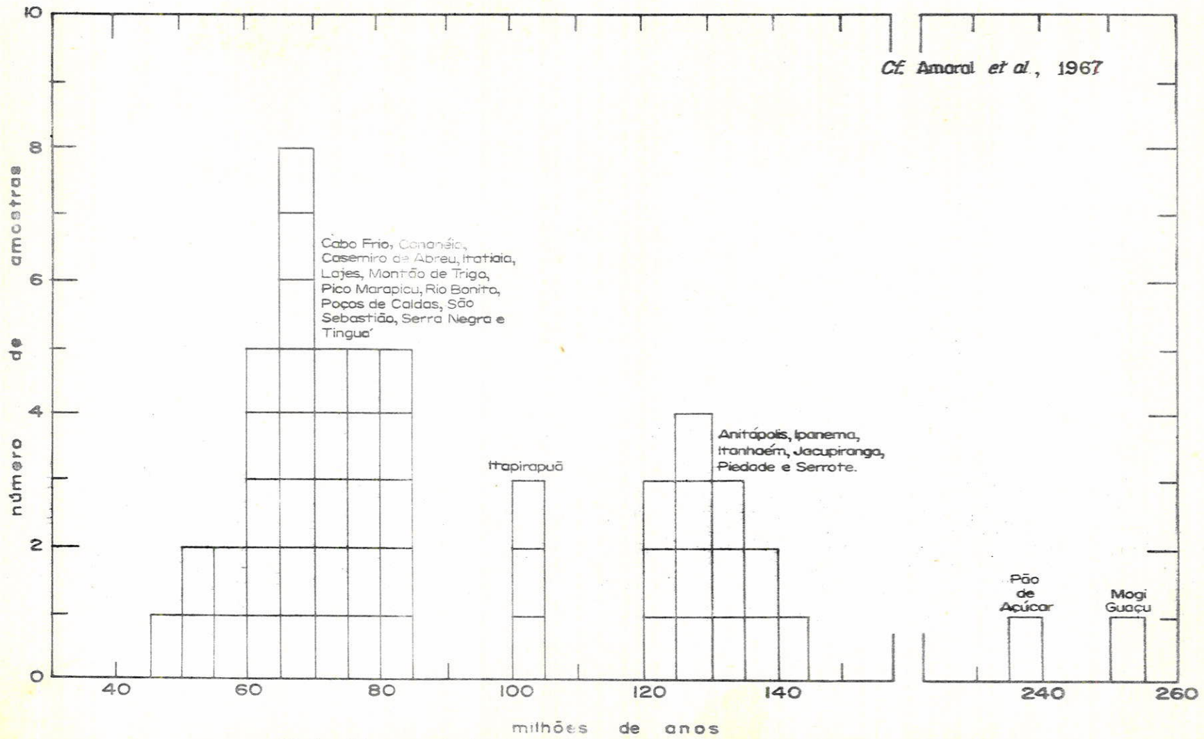
Fig. 5 — Histogramas de idades radiométricas das províncias alcalinas brasileiras.
