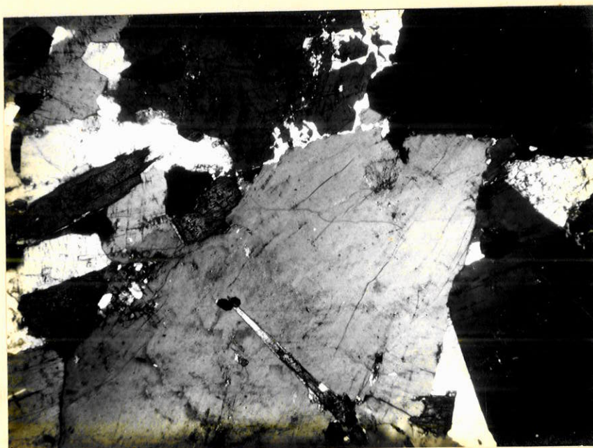
Fotomicrografia 14 - Pulaskito. Cristais de feldspato alcalino (cinza médio a escuro) associados à nefelina (cinza escuro, parte inferior da foto), Cancrinita (branca, formando-se às expensas da nefelina) e egerina-augita (cinza escuro, minerais prismáticos zonados mostrando clivagem). Nícois cruzados. Aumento: 20 X.
