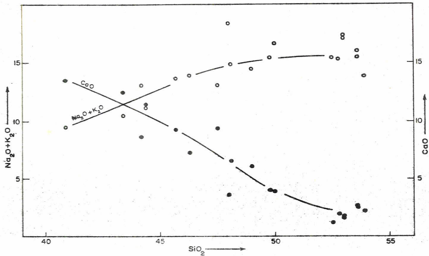
Fig. 17 — Índice cálcio-cálcico das rochas alcalinas de Itapirapuã.
