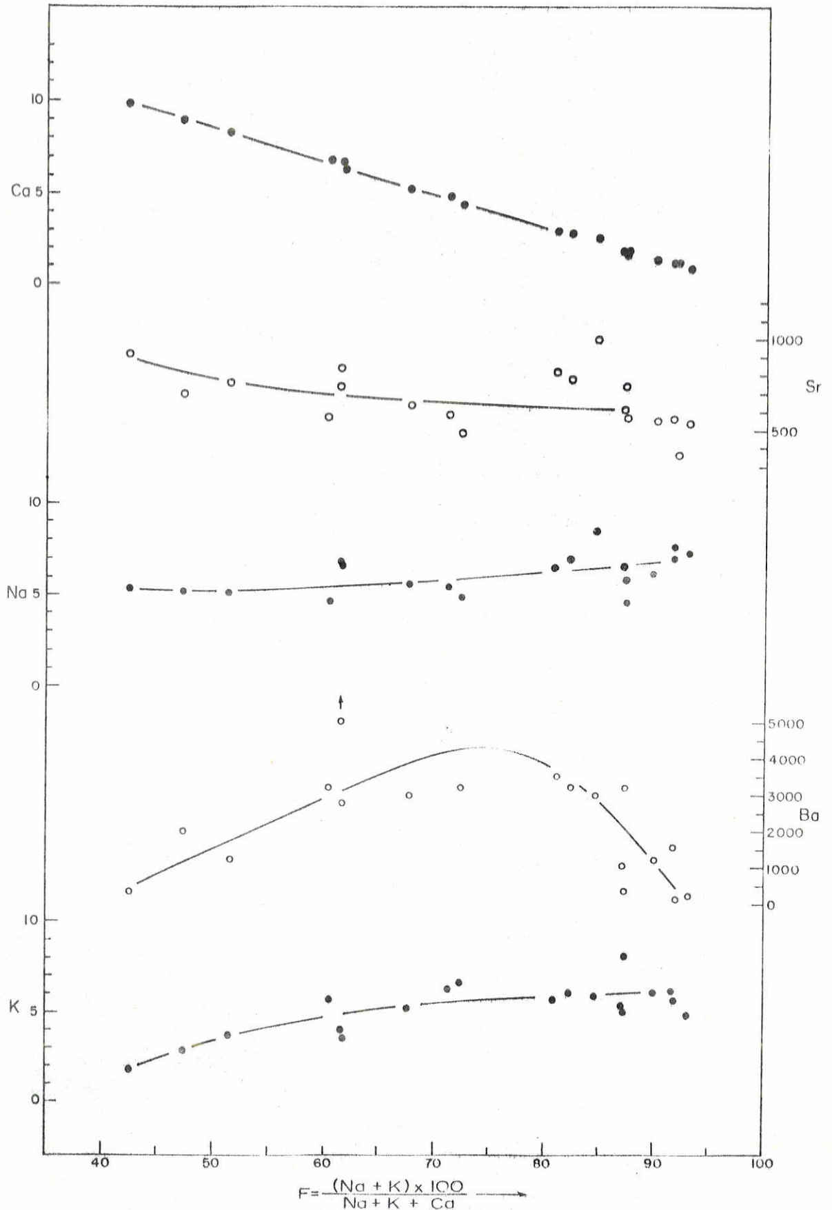
Fig.23-Diagramas de variação reunindo Ca,Na,K,Sr e Ba e o índice felsico (F) de Simpson (1954). Elementos principais expressos em % em peso e elementos traços em ppm.
