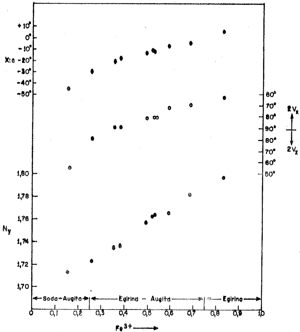
Fig. 9 — Gráfico relacionando a molécula de Egriina com as propriedades ópticas dos vários termos da série dos piroxênios de Itapirapuá.
