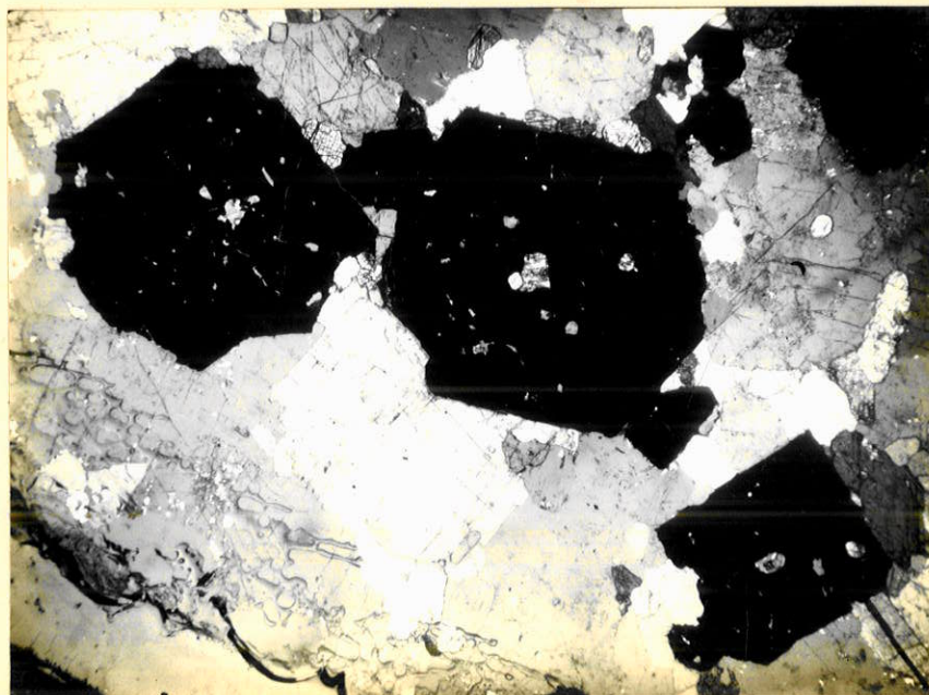
Fotomicrografia 8 - Cristais idiomórficos de granada mostrando estrutura poiquilítica. As inclusões são de nefelina e egirina-augita. Ao lado vêm-se cristais de nefelina, feldspato alcalino e egirina-augita. Nícois sub-paralelos. Aumento: 20 X.
