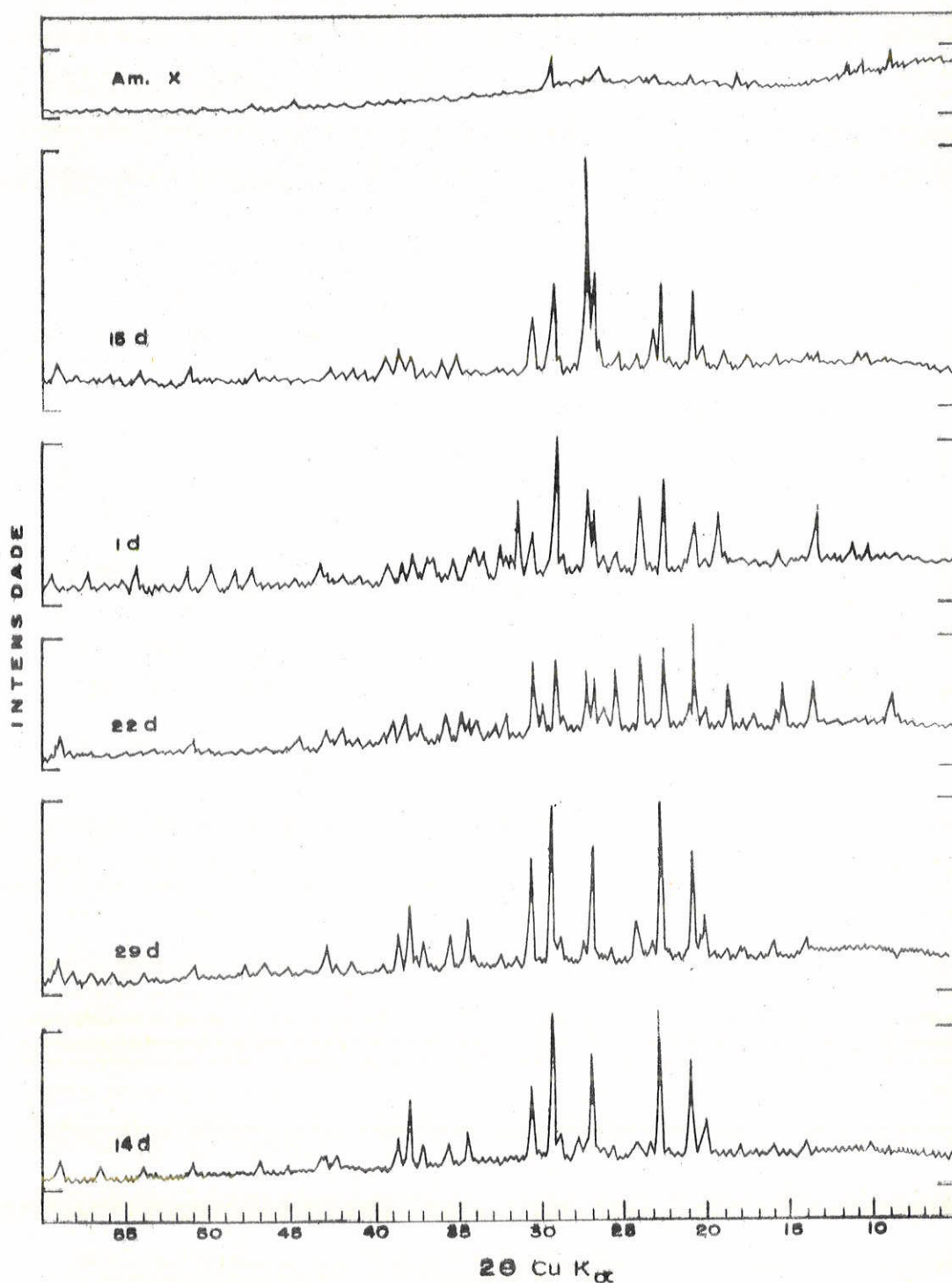
Fig. 7 - Difratogramas de nefelina e seus produtos de alteração.
