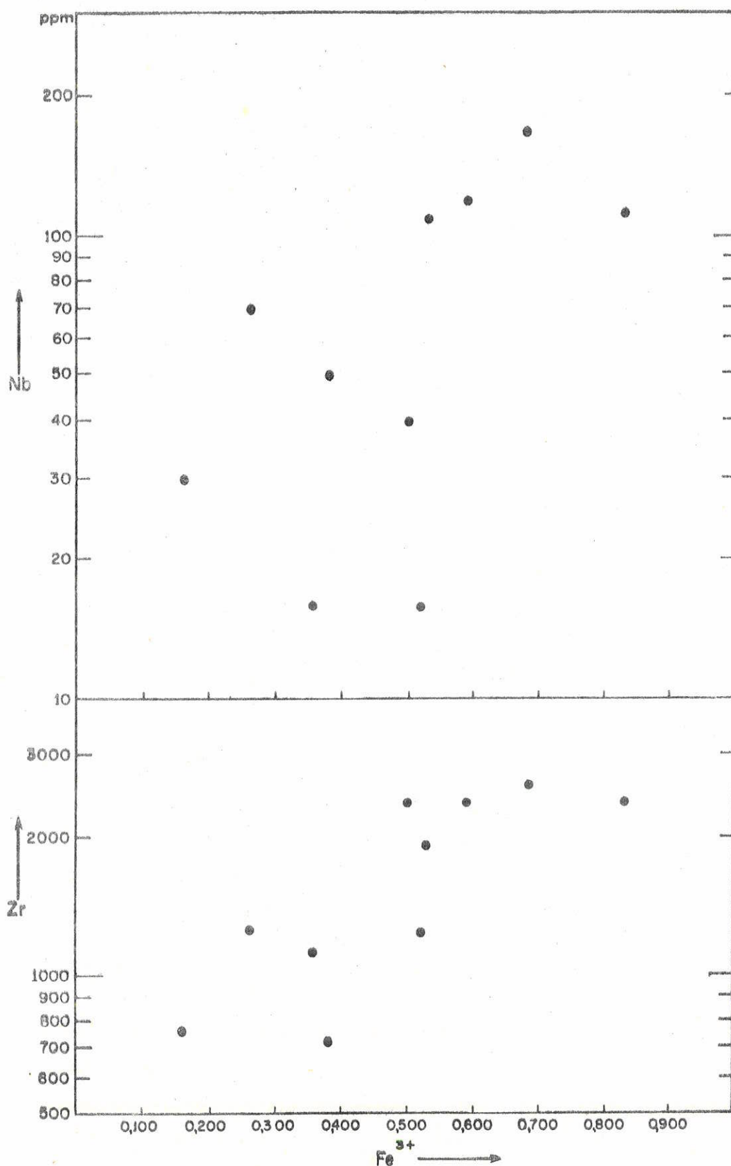
Fig.14 - Gráfico reunindo a molécula de Eglrina, expressa pela proporção atômica de Fe 3+ , e os conteúdos em Nb e Zr dos piroxênios de Itapirapuã
