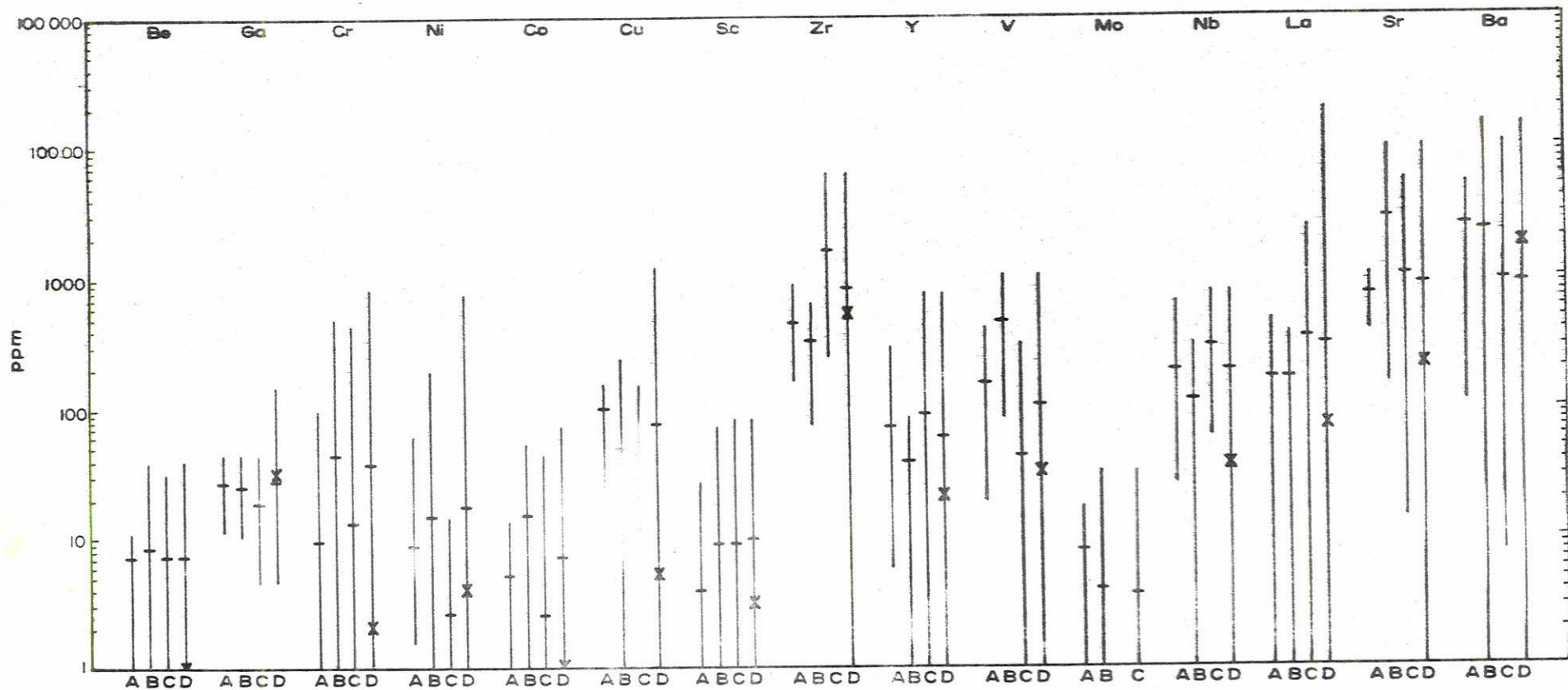
Fig. 19— Gráfico mostrando a variação no conteúdo em elementos traços das rochas de Itaipirapuã (A), Magnet Cove (B), alcalinas brasileiras (C) e mundiais (D). Os valores médios, determinados para cada elemento, estão assinalados por um pequeno traço horizontal. Uma segunda média, obtida por Turekian e Wedepohl (1961) e representada por uma marca na forma de cruz, é fornecida para as rochas alcalinas mundiais.
