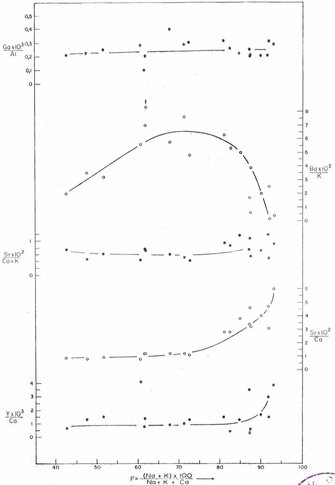
Fig. 24 - Diagramas de variaçao reunindo as relaço'es entre elementos principais e traço'es e o indice félsico (F) de Simpson (1954). Todos os valores são dados em ppm.
