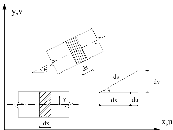
Figura 2.1 - Deformação de uma fibra genérica - SILVA (1996)
