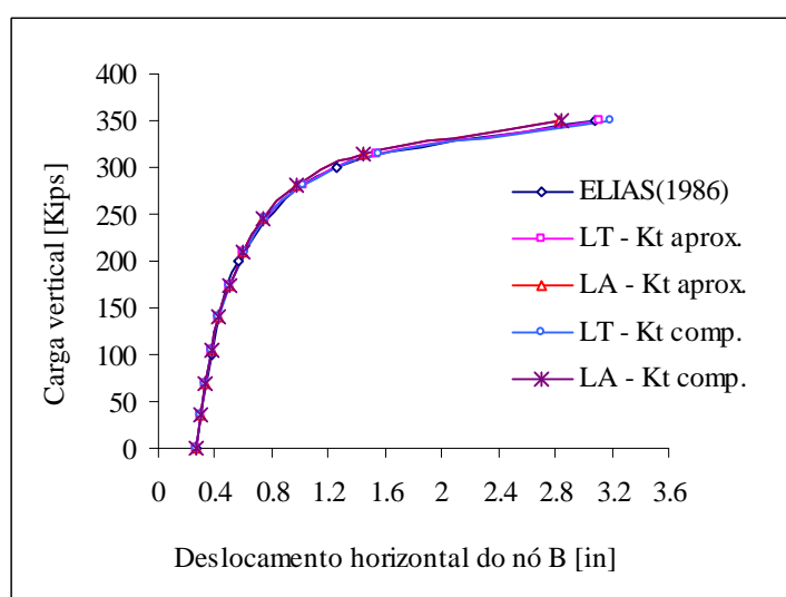
Figura 2.10- Curva carga-deslocamento
