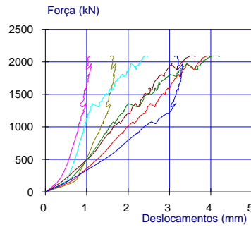
Figura 5.32 Deslocamentos da base
