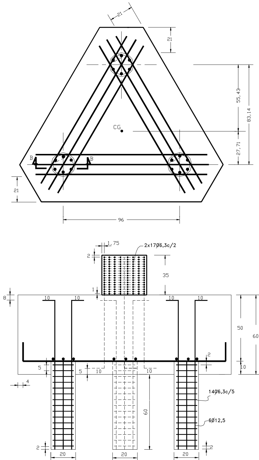
Figura 4.2. Detalhamento modelo de estacas de diâmetro de 20 cm
