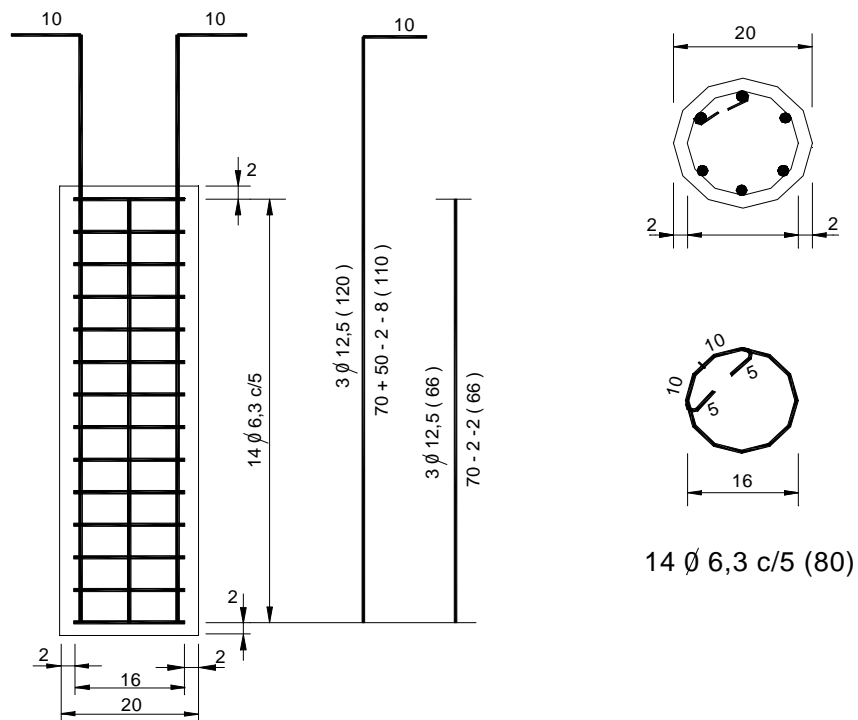
Figura 4.4. Detalhamento estacas com D = 20 cm
