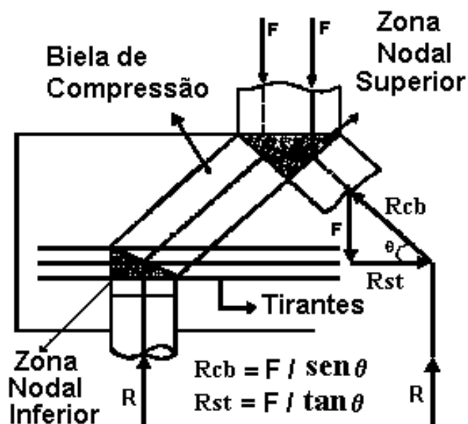
Figura 2.2. Zonas Nodais (ADEBAR et al., 1990)
