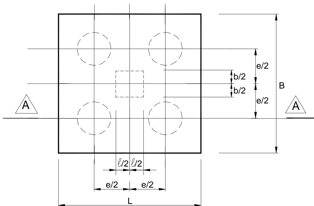
PLANTA
