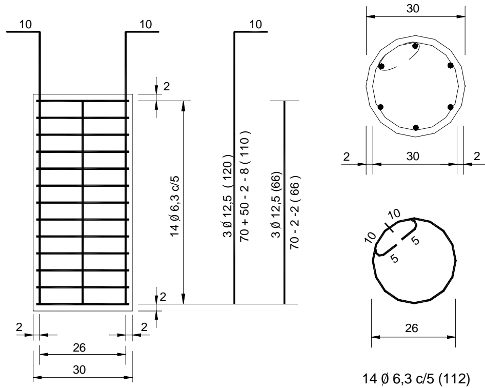
Figura 4.3. Detalhamento estacas com D = 30 cm
