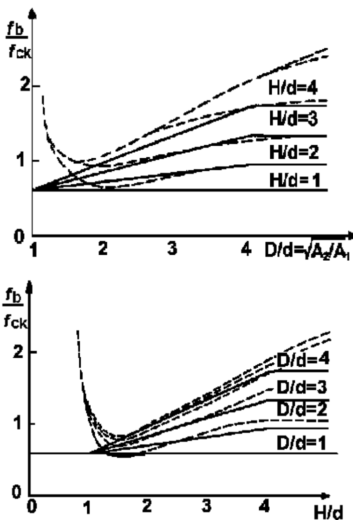
Figura 2.9. Influência do confinamento ( D/d ) e da altura ( H/d ) na capacidade das tensões para causar fendilhamento transversal: previsões analíticas (linhas tracejadas) e recomendações para projeto dadas pela Equação 1 (linhas cheias) (ADEBAR & ZHOU, 1993)
