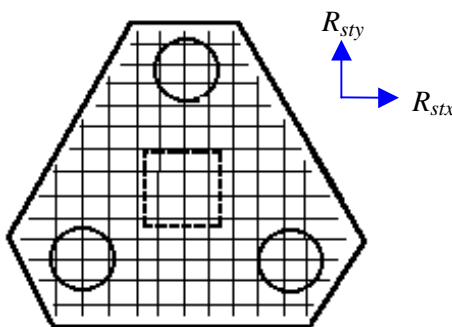
Figura 2.17. Bloco sobre três estacas com armadura em malha
