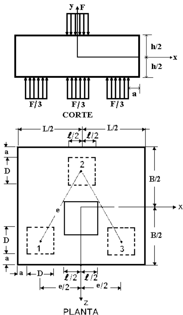
Figura 2.11. Dimensões dos blocos retangulares sobre três estacas (IYER & SAM, 1991)
