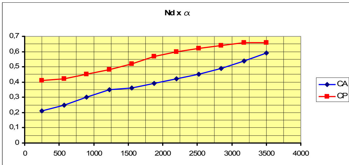
Figura 6.20 – Curva N_d \times \alpha do pilar.
